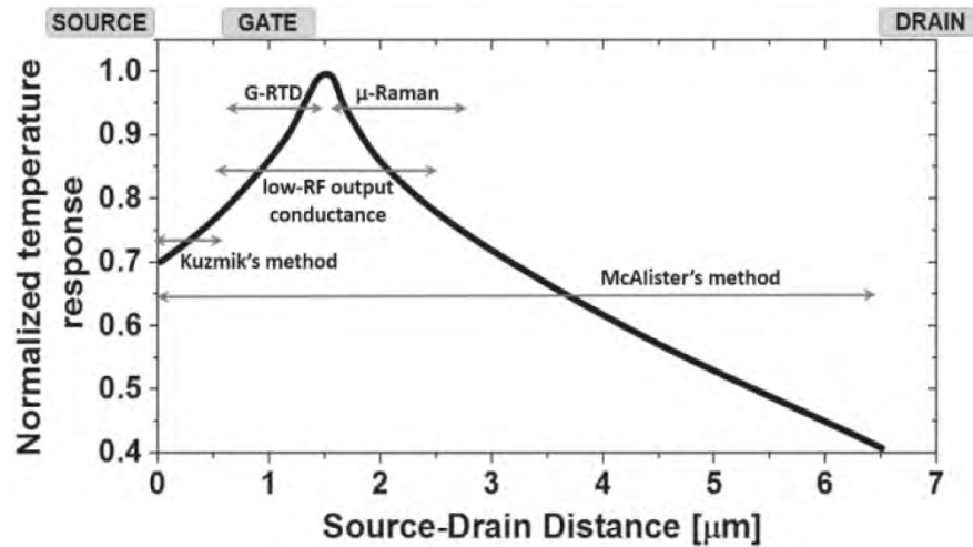
Figure I. 19 : distribution de la température simulée pour une puissance dissipée de 6,5W/mm entre les contacts de source et de drain. La courbe est normalisée par rapport au pic de température. Flèches : régions de détection de la température (moyenne) attendues pour toutes les méthodes expérimentales [66].
