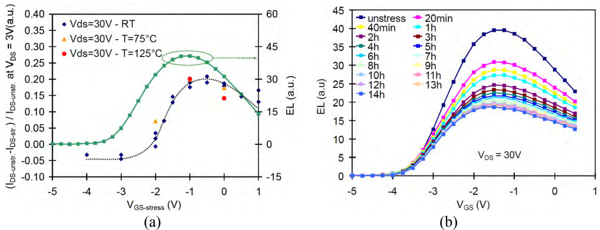
Figure I. 15 : (a) axe de gauche : dépendance du taux de dégradation sur le niveau V_{GS} appliqué durant le stress, pour des dispositifs vieillis à V_{DS}=30V . Axe de droite : intensité EL mesurée sur un dispositif avant stress. (b) signal EL en fonction de V_{GS} durant le stress à V_{DS}=30V et V_{GS}=-1V [42].
