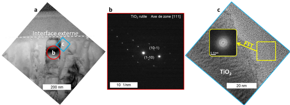
Figure IV-10 : Interface externe de l'échantillon oxydé 2 h avec un dépôt de NaCl (a) observée au MET, (b) cliché de diffraction d'un grain colonnaire, (c) grandissement au joint d'un grain colonnaire
