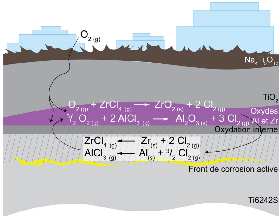
Figure IV-24 : Schéma de la formation des chlorures d'aluminium et de zirconium en parallèle de l'oxydation interne du métal
