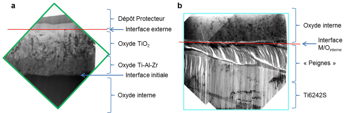
Figure IV-8 : Lames FIB extraites dans l'échantillon oxydé 2 h avec dépôt de NaCl (a) dans la couche d'oxyde et (b) à l'interface métal/oxyde
