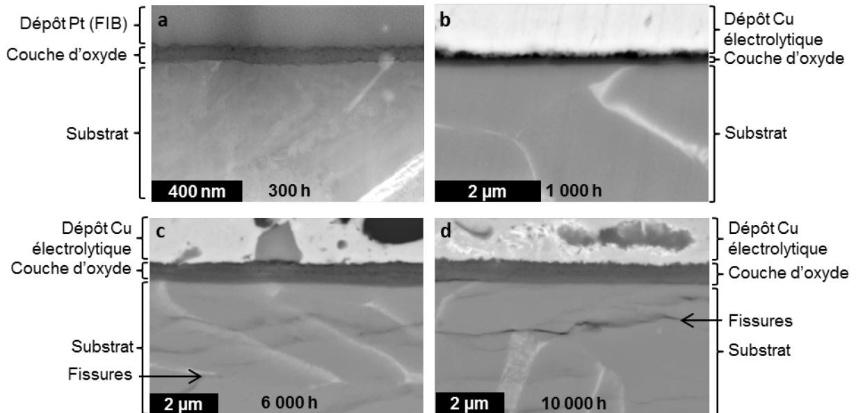
Figure III-3 : Coupes transverses des échantillons oxydés sous air (a) 300 h observée au MET, (b) 1 000 h, (c) 6 000 h et (d) 10 000 h observées au MEB
