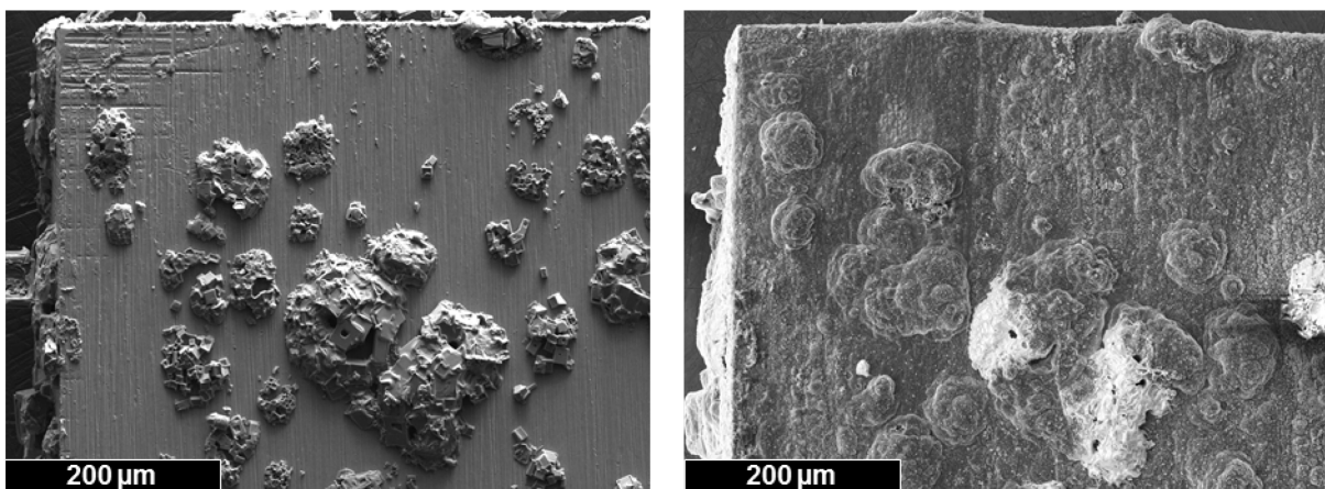
Figure IV-36 : Dépôt de NaCl sur l'échantillon de Ti6242S avant oxydation (à gauche) et après oxydation de 100 h (à droite)
