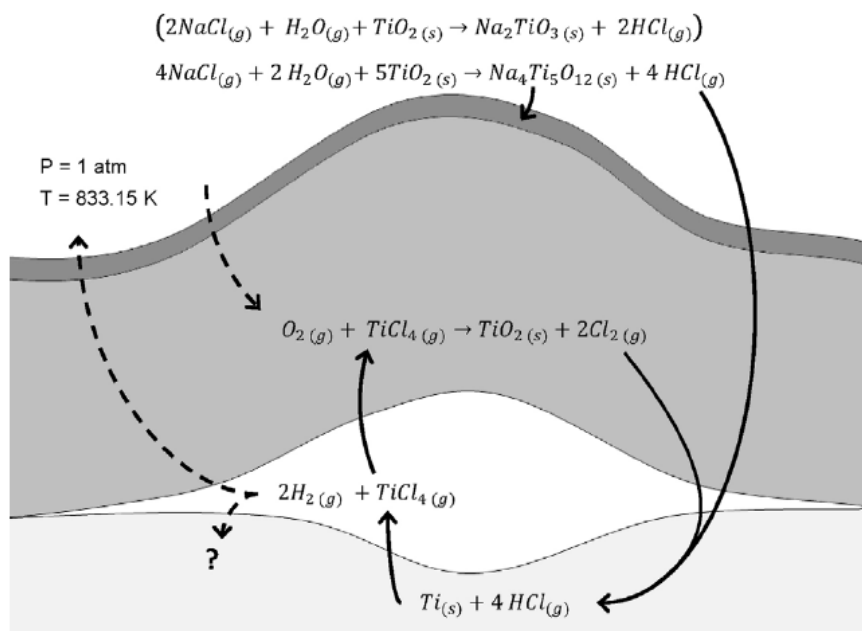
Figure I-20 : Mécanisme proposé par Ciszak et al. [126] pour la dégradation du TA6V en présence d'un dépôt solide de NaCl et de vapeur d'eau
