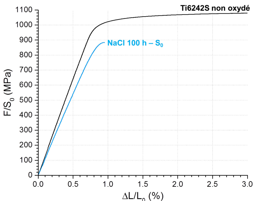
Figure V-11 : Courbe de traction l'éprouvette oxydée avec un dépôt couvrant de NaCl en considérant la section initiale S_0 de l'éprouvette
