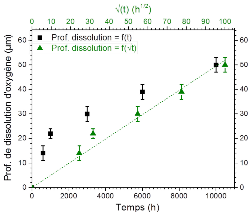
Figure III-11 : Profondeur de dissolution d'oxygène en fonction de la durée d'oxydation et en fonction de la racine carrée du temps d'oxydation
