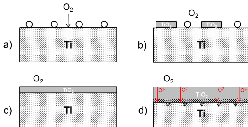
Figure I-9 : Schéma des étapes de croissance du \text{TiO}_2 sur le titane pur (figure adaptée d'après [30])
