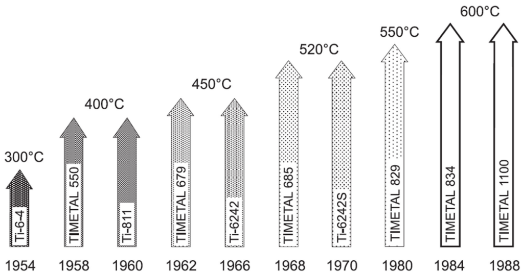
Figure I-1 : Augmentation de la température d'utilisation des alliages de titane au fil des années [30]
