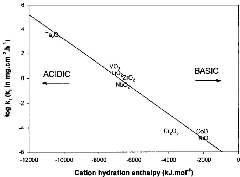
Figure I-14 : Corrélation entre la cinétique d'oxydation des métaux par la vapeur d'eau à 800°C et l'enthalpie d'hydratation du cation correspondant [116]
