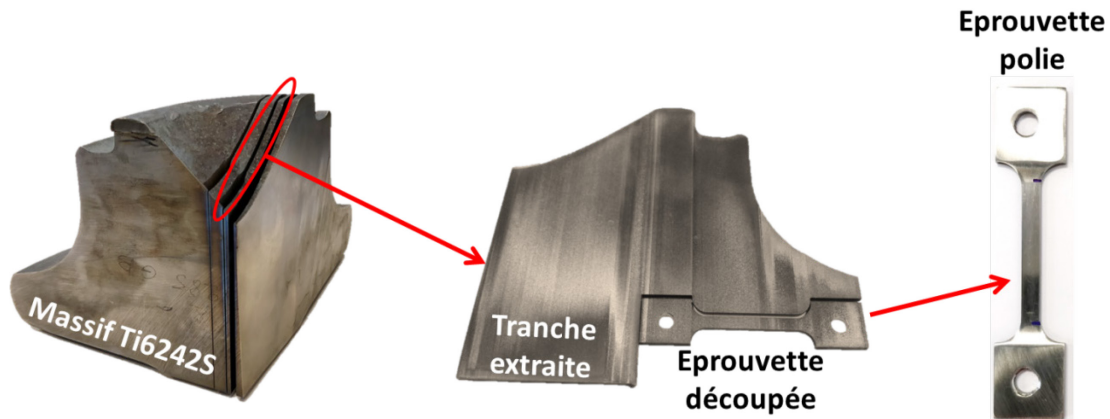
Figure II-9 : Etapes d'obtention d'une éprouvette de traction par électroérosion
