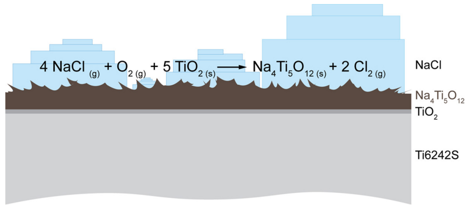
Figure IV-22 : Schéma de l'étape d'amorçage de la corrosion active en présence d'un dépôt couvrant de NaCl
