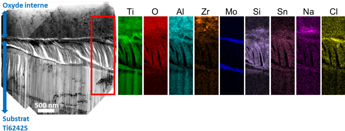
Figure IV-12 : Lame FIB de l'interface métal/oxyde d'un échantillon oxydé 2 h avec dépôt de NaCl et cartographie X de l'oxyde et du substrat Ti6242S
