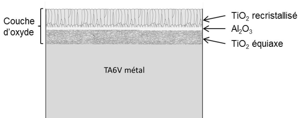
Figure I-12 : Schéma d'une couche d'oxyde formée sur TA6V oxydé par la vapeur d'eau entre 750 et 900°C
