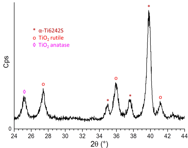
Figure III-4 : Diffractogramme obtenu en incidence rasante sur un échantillon de Ti6242S oxydé sous air de laboratoire à 560°C pendant 10 000 heures
