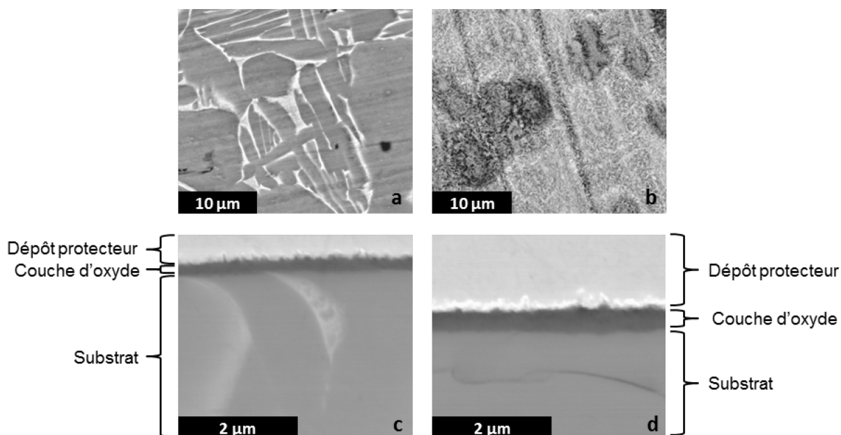
Figure III-17 : Surfaces (a) après oxydation de 100 h sous air de laboratoire, (b) de 100 h sous air enrichi en vapeur d'eau, et coupes transverses après oxydation sous air humide (c) de 100 h et (d) de 1 000 h
