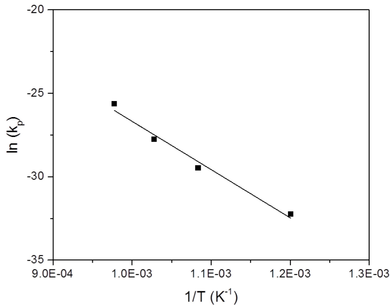
Figure III-15 : Dépendance de la constante cinétique parabolique d'oxydation de l'alliage Ti6242S avec la température
