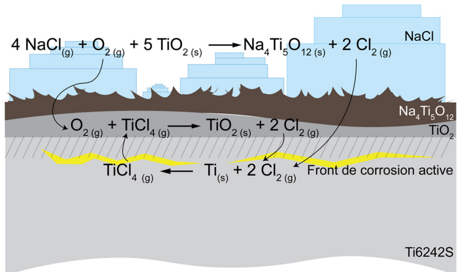
Figure IV-23 : Schéma de la formation de chlorures volatiles et consommation rapide du titane après la phase d'initialisation de la corrosion active
