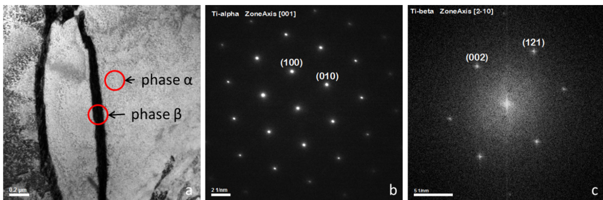
Figure II-3 : (a) Image en champ sombre de l'échantillon et clichés de diffraction correspondants à la phase \alpha (b) et à la phase \beta (c)
