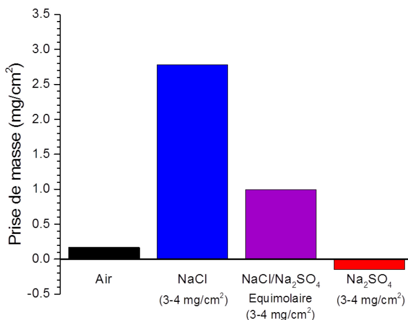
Figure IV-39 : Comparaison des prises de masse après 1 000 h d'oxydation sans dépôt de sel, avec un dépôt couvrant de NaCl, d'un mélange équimolaire \text{NaCl}/\text{Na}_2\text{SO}_4 , de \text{Na}_2\text{SO}_4
