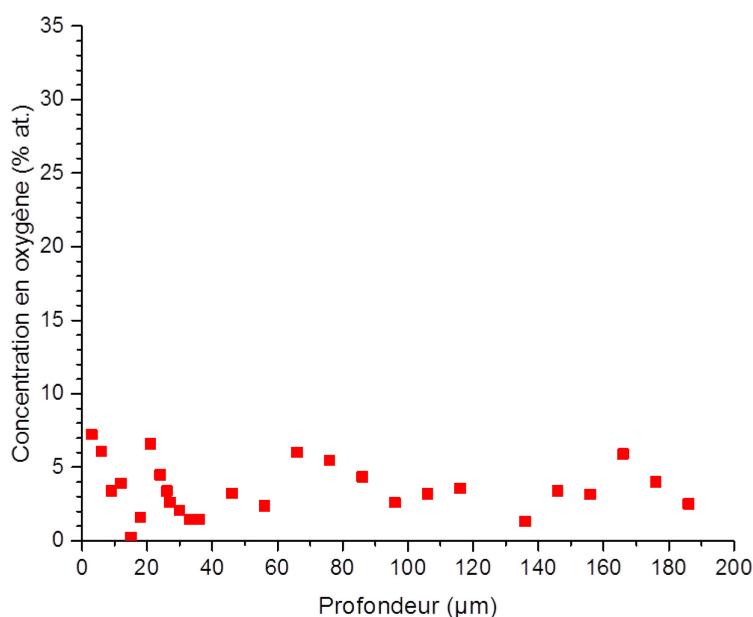
Figure V-20 : Profil EDX réalisé sur la coupe transverse de l'éprouvette oxydée 100 h avec le dépôt de \text{NaCl}/\text{Na}_2\text{SO}_4
