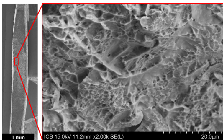
Figure V-3 : Fractographies MEB de l'éprouvette rompue
