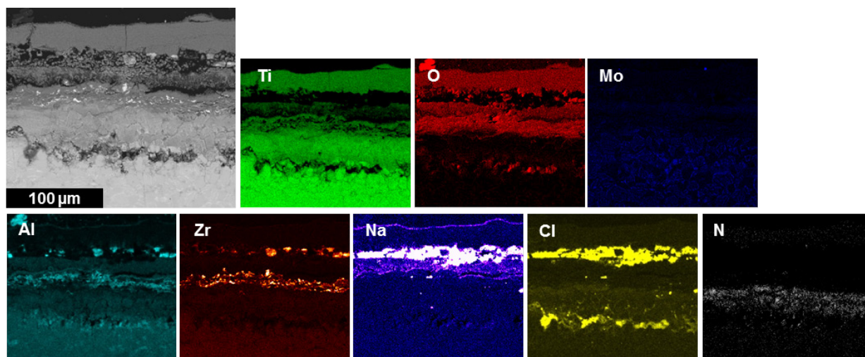
Figure IV-34 : Cartographie X en coupe transverse de l'échantillon oxydé 10 000 h avec un dépôt de 1 \text{ mg/cm}^2 de NaCl
