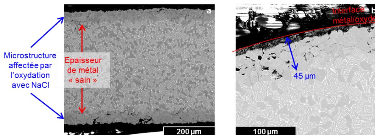
Figure V-10 : Observation au MEB en coupe transverse (a) de toute l'épaisseur et (b) avec un plus grand grandissement de l'éprouvette oxydée 100 h avec un dépôt couvrant de NaCl à l'endroit de la rupture
