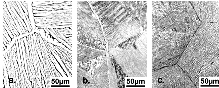
Figure I-4 : Microstructures lamellaires obtenues par refroidissement à : a) 1 K/min, b) 100 K/min et c) 8 000 K/min [34]
