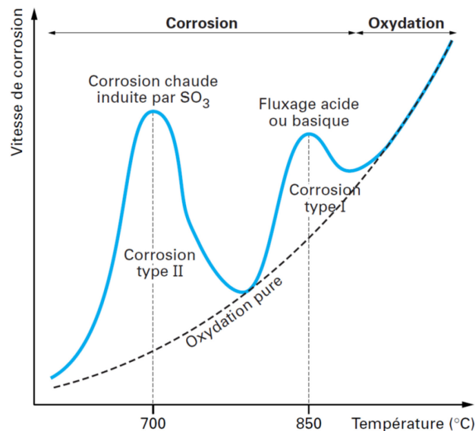
Figure I-17 : Evolution de la vitesse de corrosion en fonction de la température dans des conditions de « hot corrosion » [129] (d'après Streiff [130])
