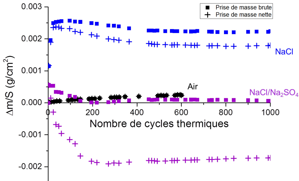
Figure IV-42 : Courbes de prise de masse brute (carrés pleins) et nette (symbole +) des échantillons de Ti6242S recouverts de NaCl ou d'un mélange NaCl/ \text{Na}_2\text{SO}_4 équimolaire
