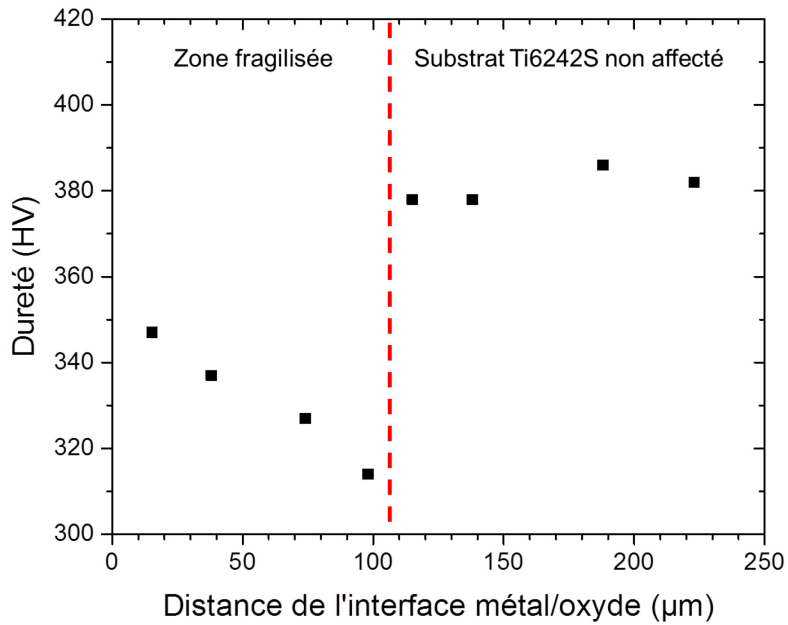
Figure IV-18 : Profil de dureté en surface d'un échantillon oxydé 1 000 h avec un dépôt de 3 à 4 mg/cm 2 de NaCl
