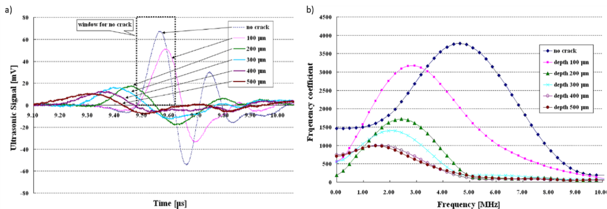
Figure 2-19 (a) Diminution de l'amplitude de l'onde réfléchi avec la hauteur de l'entaille. (b) Diminution de la fréquence de l'onde réfléchi avec la hauteur du défaut, extrait de [78].
