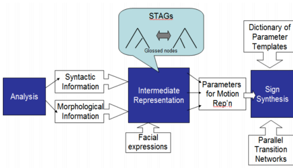
Figure 3.9 : Architecture de TEAM PROJECT (Zhao et al, 2000)
