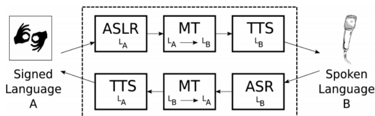
Figure 3.13: Les différents composants du projet SignSpeak (Dreuw et al, 2010)
