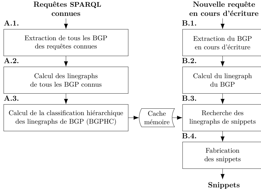
Figure 4.5 – Schéma du workflow de génération des snippets de SPARQLets-Finder où A.1-3 construit le BGPHC nécessaire à B.1-4 afin de générer des propositions de snippets pour une requête en cours d'écriture.
