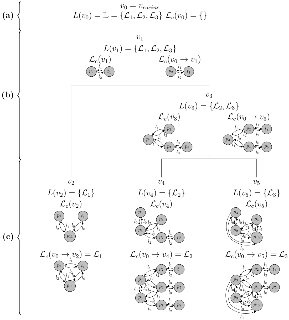
Figure 4.4 – Exemple de classification hiérarchique des linegraphs de BGP (BGPHC) à l'issue du processus A.3 à partir des BGP BGP_1 , BGP_2 et BGP_3 des figures 4.2 et 4.3.
