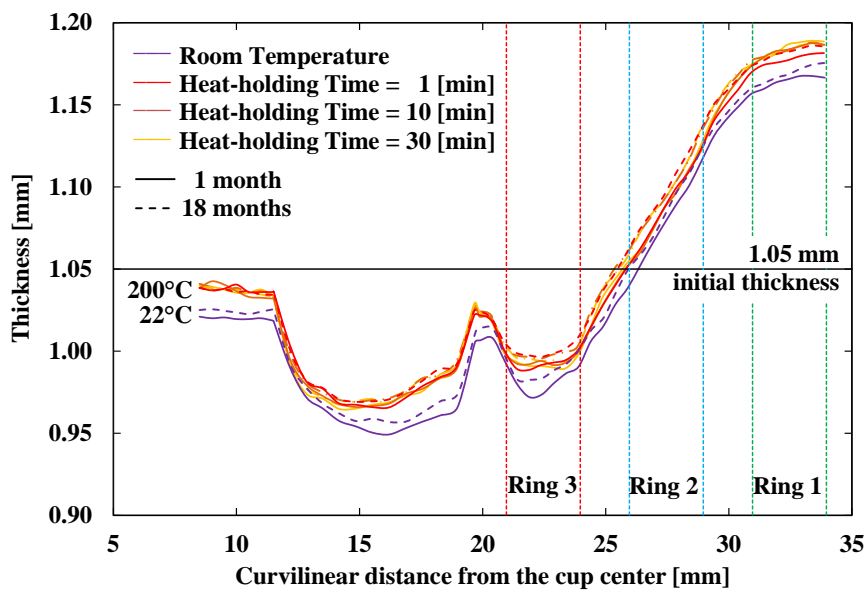
a) EN AW 6016-T4
