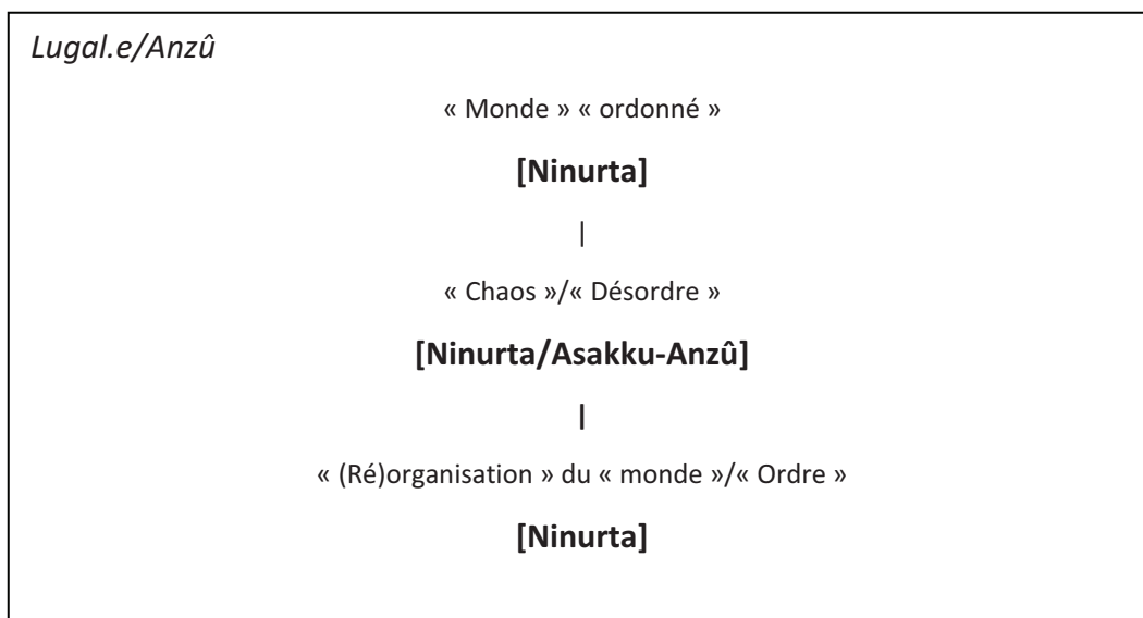
Figure 6. « "Chaos" cratogonique »
