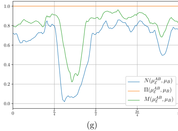
Figure 6.11 – Profils directionnels de nécessité-possibilité (en bleu et orange) et moyens (en vert) d'entourement pour l'image du bassin d'Arcachon présentée en Figure 6.9.
