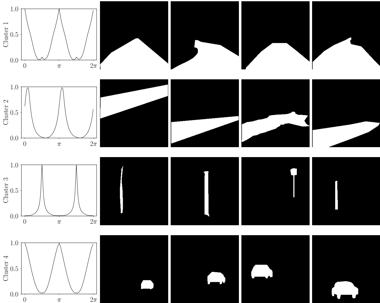
Figure 8.5 – Exemples illustratifs de mots de formes obtenus pour des images de scènes d’extérieur. Chaque ligne correspond à un cluster différent. À gauche : le centroïde du cluster représenté par une courbe. À droite : quelques exemples de formes dont l’histogramme de forces à été rattaché à ce centroïde.
