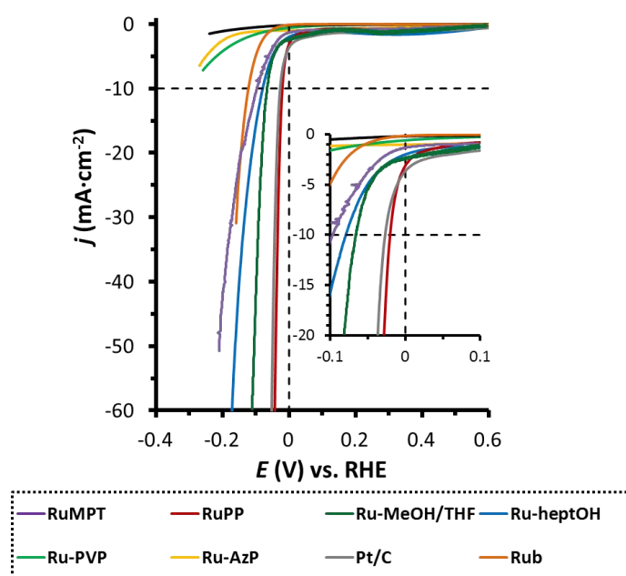
Figure 9. Courbes de polarization des différents systèmes de RuNPs testés dans une solution \text{H}_2\text{SO}_4 1 M.
