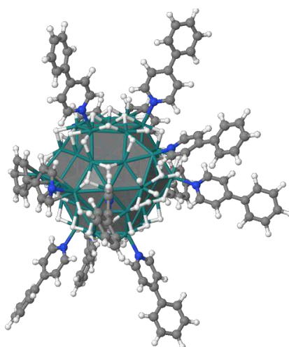
Figure 11. Modèle 1 nm de RuNP protégée par le ligand (Ru 55 H 53 σPP 9 πPP 2 ).
