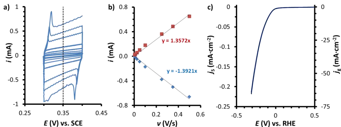
Figure 19. Calcul ECSA par la méthode électrochimique décrite par Jaramillo et al. (a et b) et c) Courbe de LSV normalisée par ECSA (à gauche) et par la surface estimée S = 0,3 \text{ cm}^2 (à droite) en condition 1 M H_2SO_4 .
