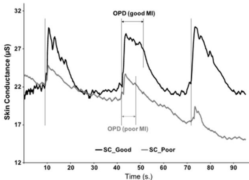
Figure 15. Variation du niveau de conductance cutanée au cours de la simulation mentale de l'action. D'après Collet et al. 2011.
