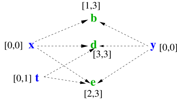
FIGURE 4.4 – Le graphe abstrait de E_1 . Les chemins des entrées vers les sorties sont remplacés par de simples arcs.
