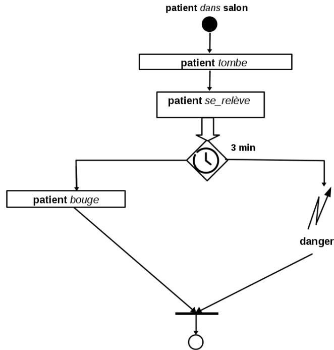
FIGURE 3.13 – Deuxième format graphique de l'exemple (ADeL)
