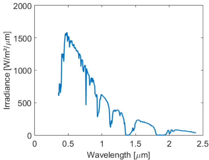
Figure 3.25 : Spectre d'éclairissement BOA simulé par DART pour la configuration atmosphérique du 24.06.2016 à 10:37 à Bâle (Suisse). Simulation réalisée avec 410 bandes spectrales de 5nm de largeur, entre 0.350\mu m et 2.4\mu m
