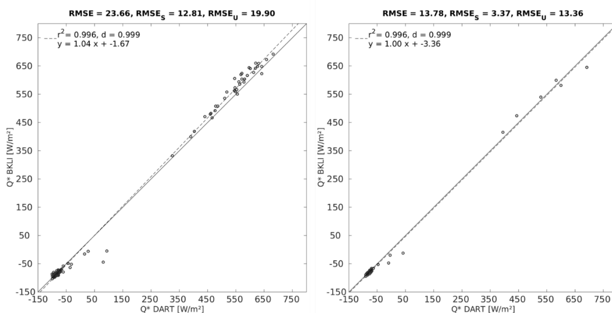
Figure 4.31 : Corrélogrammes de comparaison entre les valeurs de Q^* simulées et mesurées au niveau des tours de flux BKLI à Bâle (droite) et KSSW à Londres (gauche), pour la série d'acquisition de Sentinel-3
