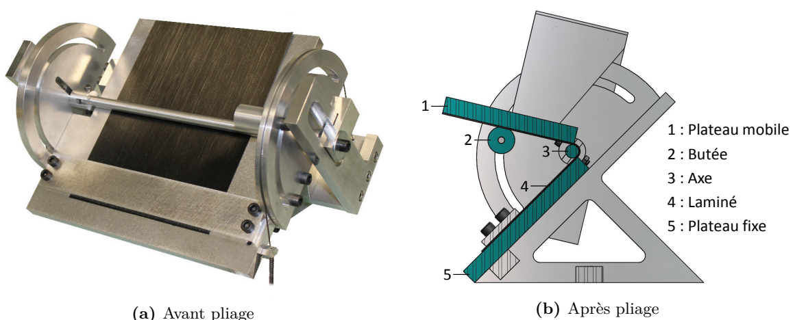
Figure 3.5 – Dispositif de thermo-plieuse pour composites
