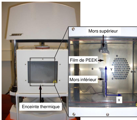
Figure 4.2 – Dispositif expérimental
