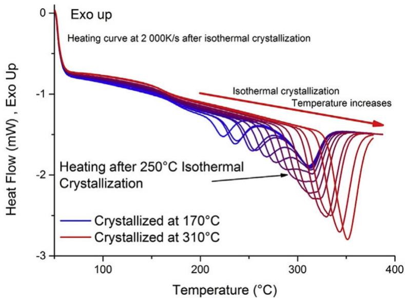
Figure 1.14 – Thermogrammes pour une vitesse de rampe de 2000 K.s -1 après la cristallisation du PEEK à des isothermes compris entre 170°C et 300°C [Tardif+2014]
