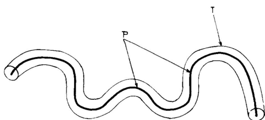
Figure 2.11 – Théorie de la reptation [De Gennes1971]
