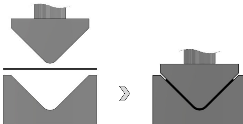
Figure 1.24 – Procédé d'estampage
