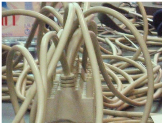
Illustration 60 (gauche) : Octopus , connecteur central, douze câbles 25 broches.
