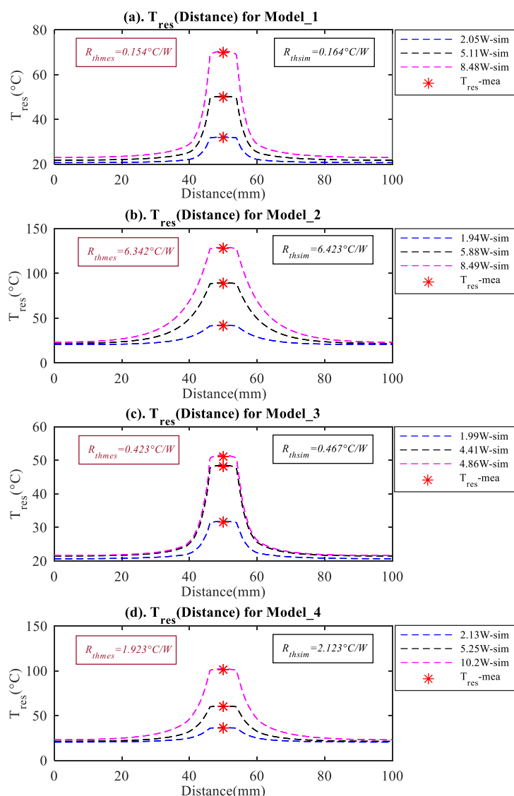
Figure 7: Comparaisons des résultats de simulation et des résultats d'expérience. Les températures au milieu de la surface de PCB sont obtenues par simulation thermique 3D. La température de l'élément chauffant est mesurée par thermocouple.
