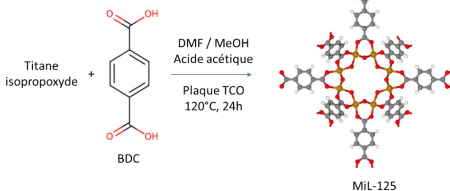
Figure 65 : Schéma de la synthèse du MIL-125 sur TCO par croissance solvothermale directe in situ sur FTO, dans les conditions de références.
