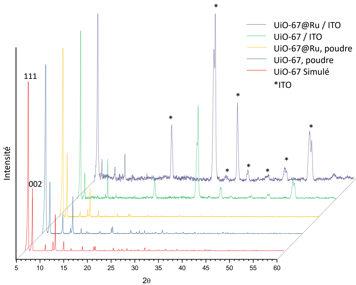
Figure 40 : Diffractogrammes DRXP des composés suivants : UiO-67 simulé, UiO-67 et UiO-67@Ru sur poudre et greffés sur le support ITO.
