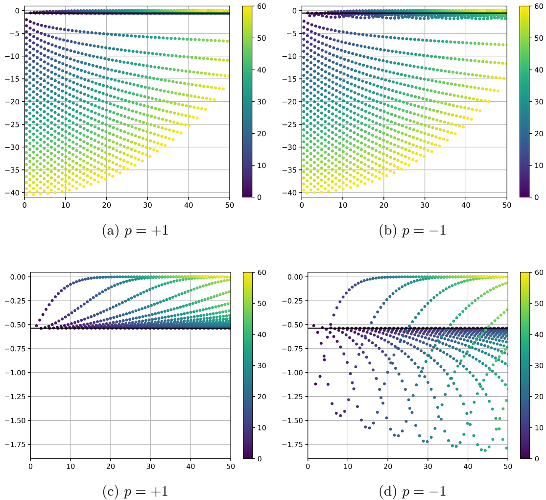
FIGURE 3.3 – Représentation graphique des zéros, dans le plan complexe, de la fonction modale \mathcal{D}_{p,m} définie en (3.5) pour p \in \{\pm 1\} , n_0 = 1.5 et 0 \leq m \leq 60 . La colonne de gauche représente p = +1 et celle de droite représente p = -1 . La ligne du haut représente une vue globale des résonances. La ligne du bas est un zoom sur les résonances internes et on y observe la droite horizontale correspond à la constante \frac{1}{2n_0} \ln\left(\frac{n_0-1}{n_0+1}\right) (la limite de \text{Im}(k_j(m)) quand j \rightarrow +\infty ).
