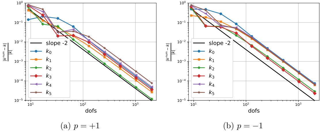
FIGURE 2.9 – Erreur relative des 6 premières résonances en échelle logarithmique. Les valeurs des paramètres sont celles de l'exemple de référence 2.5 page 28 : \alpha = 0.5 , \beta = 1 , n_0 = 2 . La PML utilisé est celle de classe \mathcal{C}^2 (PML2) avec les paramètres : r_0 = 2 , r_1 = 3 , \sigma_0 = 2 et R = 4 .
