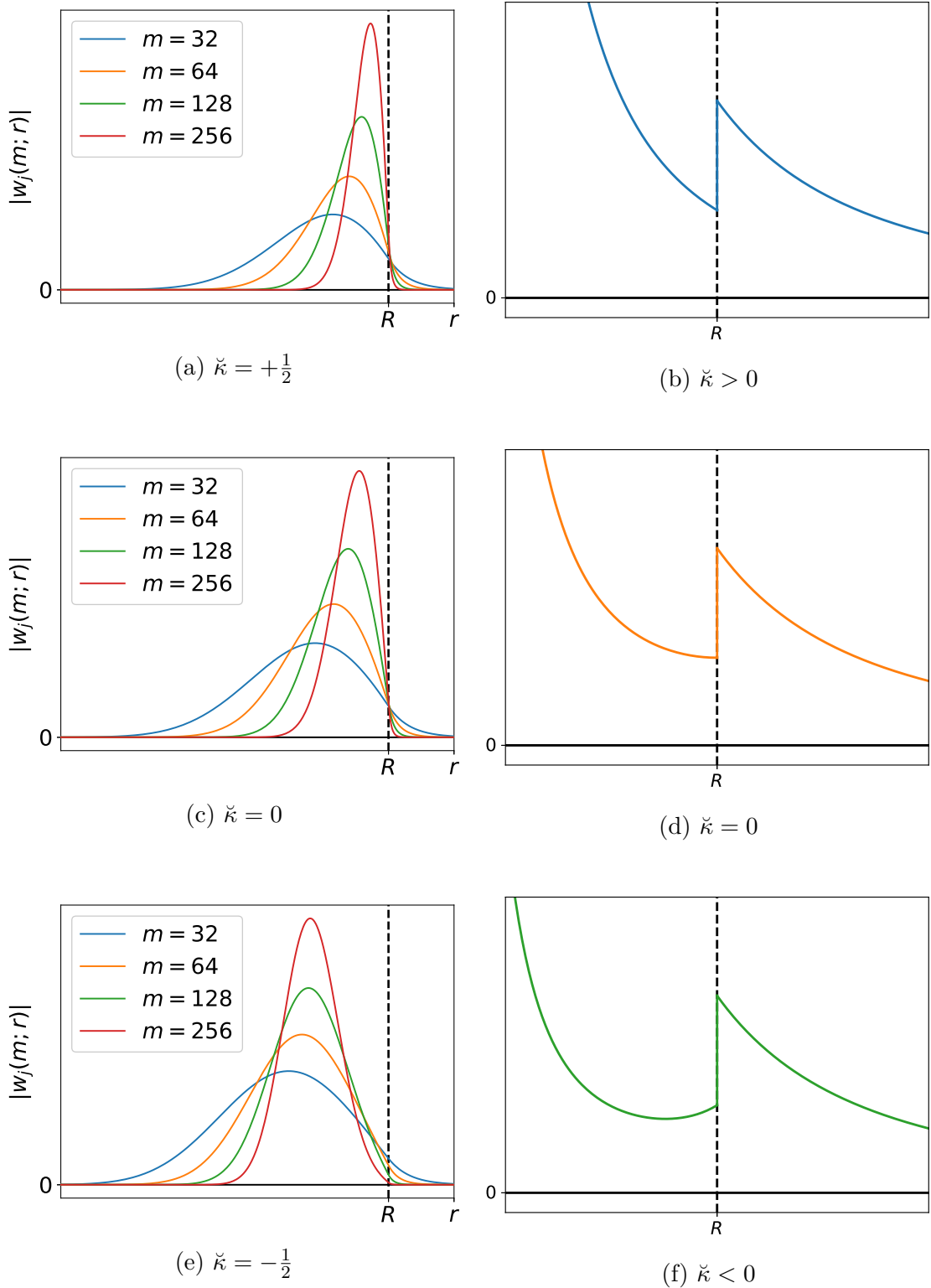
FIGURE 6.2 – Sur la colonne de gauche, graphes des modes résonnants w_{p;j}(m) pour p = +1 , j = 0 et m \in \{32, 64, 128, 256\} . La fonction n a pour paramètres n_b = 5 et \check{\kappa} = \{-\frac{1}{2}, 0, \frac{1}{2}\} . Sur la colonne de droite, allure des fonctions W pour \check{\kappa} > 0 , \check{\kappa} = 0 et \check{\kappa} < 0 .
