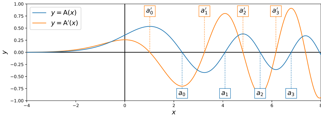
FIGURE C.1 – Graphes des fonctions A et A' et localisation des zéros de A et A' .
