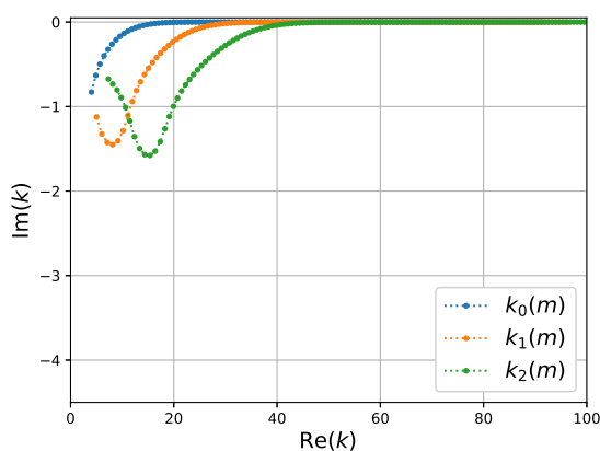
(a) Disque
