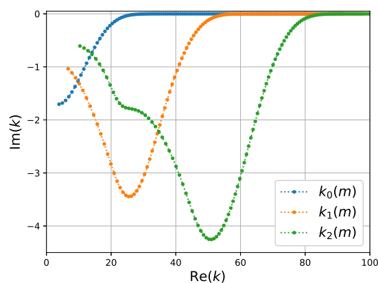
(b) Anneau
