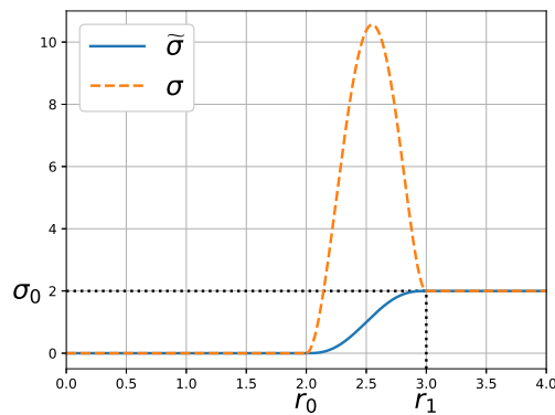
FIGURE 2.4 – Représentation graphique des fonctions \tilde{\sigma} et \sigma , avec les paramètres r_0 = 2 , r_1 = 3 et \sigma_0 = 2 pour les trois cas de régularité considérés.
