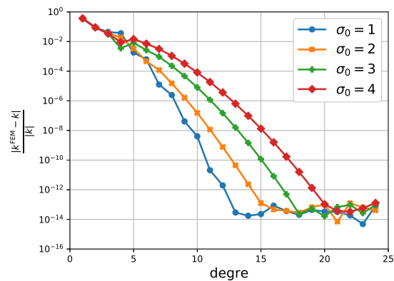
(d) k_{1,1}
