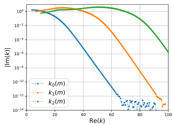
(d) Anneau
