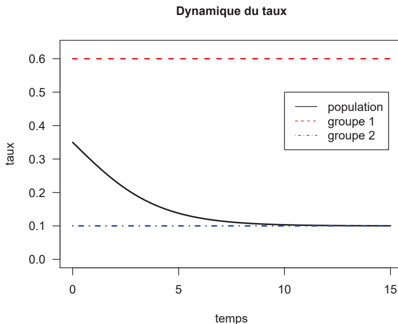
Figure 2.3 – Mélange de deux taux constants
