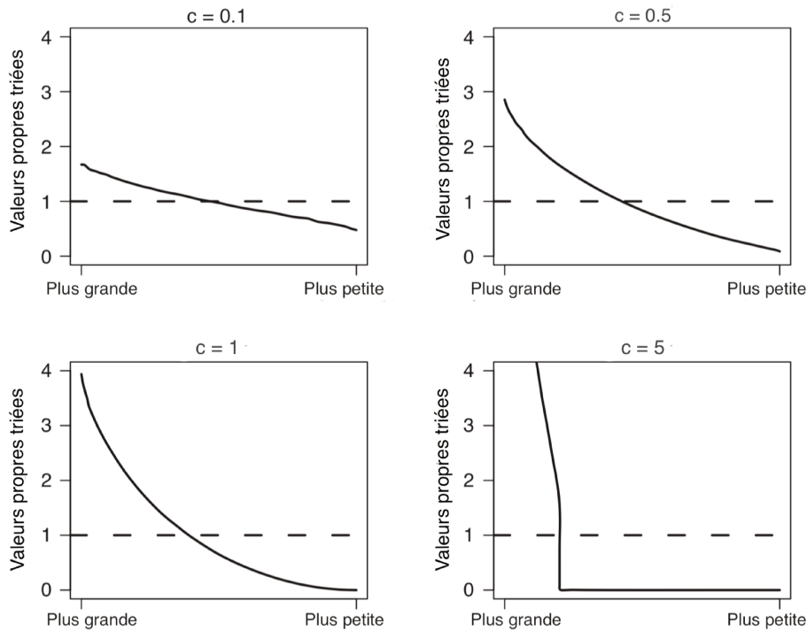
FIGURE 1.1 – Estimation des valeurs propres de \Sigma = I_p par \hat{\Sigma}_{1/n-1} .
