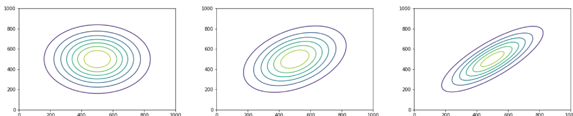
FIGURE 5.4 – Contours de la loi normale avec des covariances positives.
