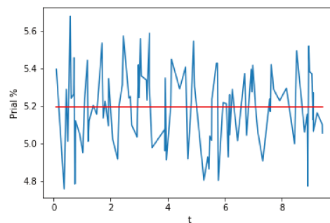
FIGURE 5.7 – Effet de t sur le PRIAL lorsque (\Sigma)_{ij} = 0.9^{|i-j|} pour (p, n) = (120, 100)
