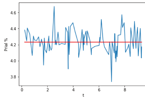
FIGURE 5.6 – Effet de t sur le PRIAL lorsque \Sigma = I_p pour (p, n) = (120, 100)
