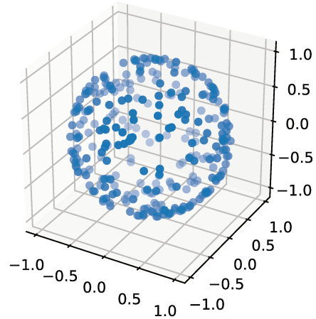
FIGURE 5.2 – Loi uniforme sur la sphère unité.
