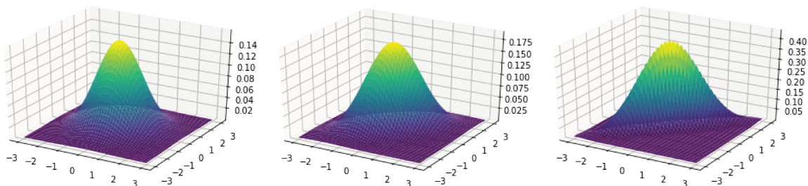
FIGURE 5.3 – Densités de la loi normale pour \Sigma proportionnel à I_2 .
