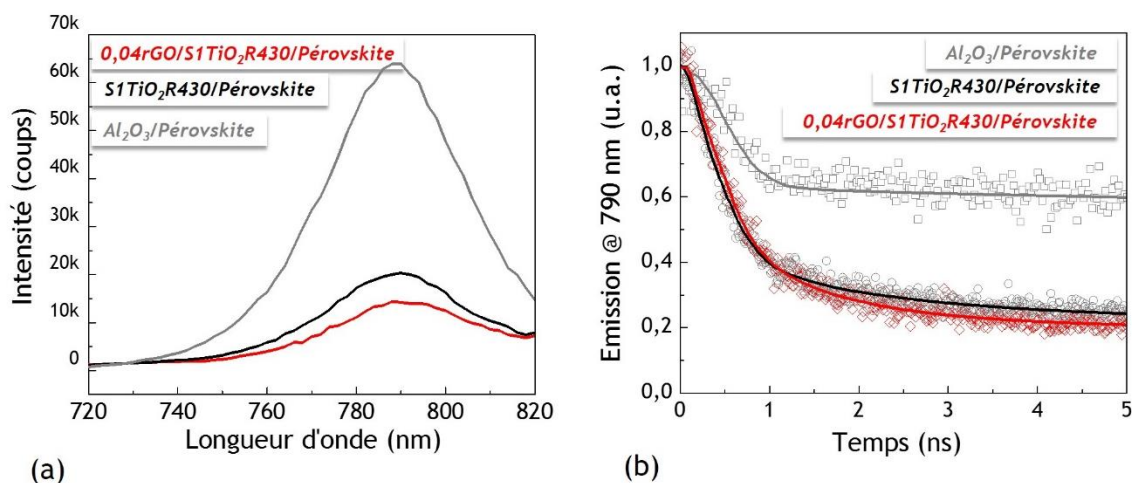
Figure IV-8 Spectroscopie de photoluminescence sur \text{Al}_2\text{O}_3 (couche isolante) \text{TiO}_2 - et \text{TiO}_2\text{-rGO} (couches transporteuses d'électrons)/Pérovskite, respectivement courbes grise, noire et rouge (a) En régime stationnaire – excitation à 510 nm (b) Résolue en temps – émission à 790 nm
