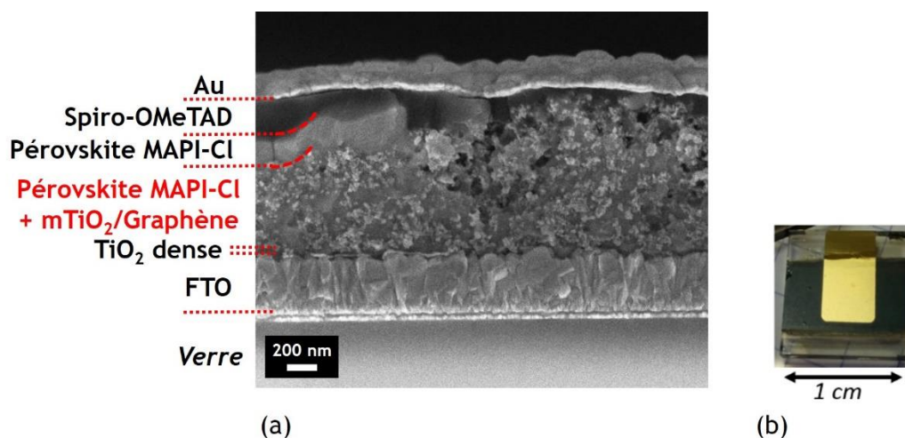
Figure IV-12 (a) Image MEB en coupe d'une cellule photovoltaïque pérovskite élaborée dans le cadre de ce travail de thèse (b) photographie d'une cellule solaire pérovskite – vue du dessus
