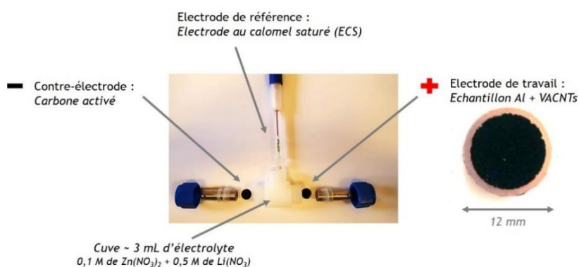
Figure V-21 Montage à trois électrodes pour l'électrodépôt de ZnO sur Al/VACNTs
