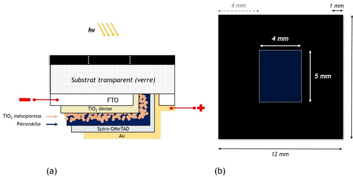
Figure II-34 (a) Schéma en coupe d'une cellule solaire pérovskite sous éclairement (b) Schéma de la cellule solaire masquée laissant la surface active apparente mesurée (4 mm x 5 mm) (vue du dessus)
