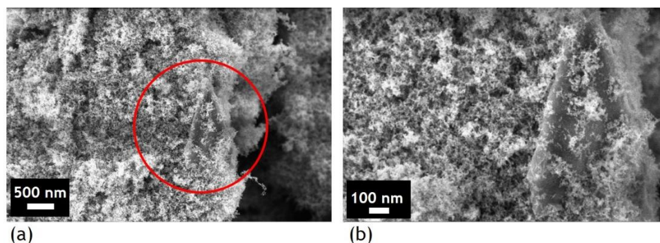
Figure III-32 Images MEB d'une poudre recuite de nanocomposites TiO_2 /graphène synthétisée par pyrolyse laser (a) nanoplaquette de graphène GNP observée au sein de la poudre de nanoparticules de TiO_2 (b) zoom sur la nanoplaquette de graphène GNP – images réalisées sur la poudre 0,08GNP/S3 TiO_2 R450
