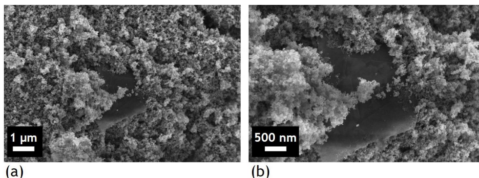
Figure III-31 Images MEB d'une poudre recuite de nanocomposites TiO_2 /graphène synthétisée par pyrolyse laser (a) nanoplaquette de graphène GNP observé au sein de la poudre de nanoparticules de TiO_2 (b) zoom sur la nanoplaquette de graphène GNP – images réalisées sur la poudre 0,08GNP/S2 TiO_2 R450
