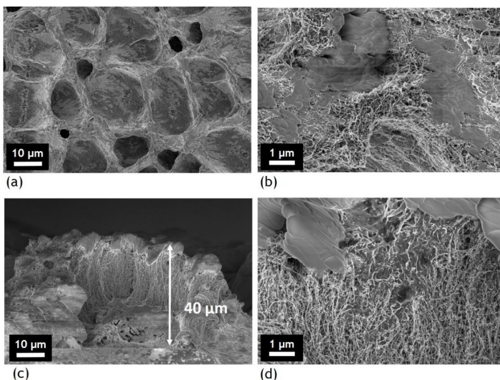
Figure V-11 Images MEB en surface (a) et (b) et en coupe (c) et (d), après dépôt en une étape de pérovskite de type \text{CH}_3\text{NH}_3\text{PbI}_{3-x}\text{Cl}_x (MAPI-Cl) sur VACNTs de 40 \mu\text{m}
