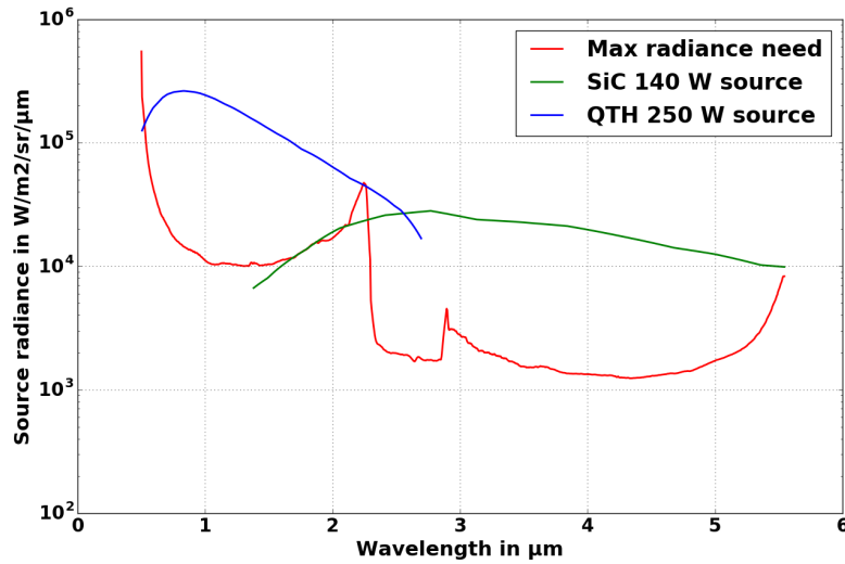
Fig. 5.28. : Radiance spectrale requise au minimum pour satisfaire les spécifications de mesure de lumière parasite (contraste de 10^5 ) en rouge, et radiance spectrale disponible avec les deux sources sélectionnées pour cette voie : QTH de 250 W en bleu et barre de SiC 140 W en vert.
