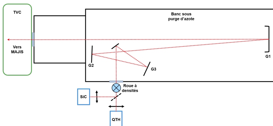
Fig. 5.36. : Schéma de la voie de mesure de la lumière parasite de MAJIS.
