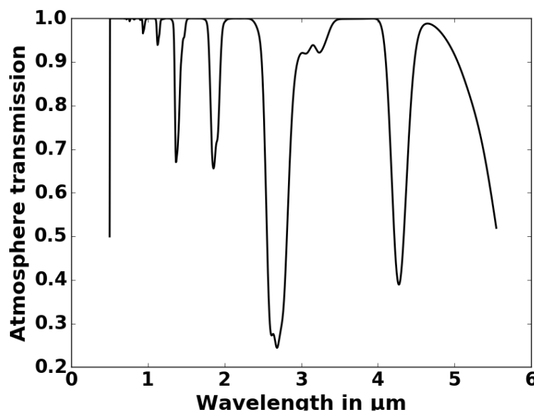
Fig. 5.5. : Transmission d'une colonne d'air de 10.5 m en considérant une composition standard d'atmosphère, sous 1 bar et à 20°C avec une hygrométrie de 50 %.
