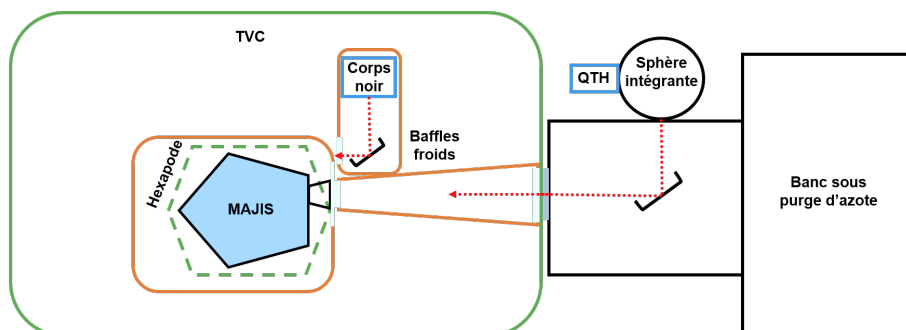
Fig. 5.31. : Schéma des voies optiques d'étalonnage radiométrique absolu de MAJIS.
