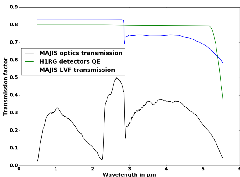
Fig. 5.3. : Courbes de transmission (ou de conversion dans le cas de la QE) instrumentales considérées pour les applications numériques du modèle utilisé dans la suite.
