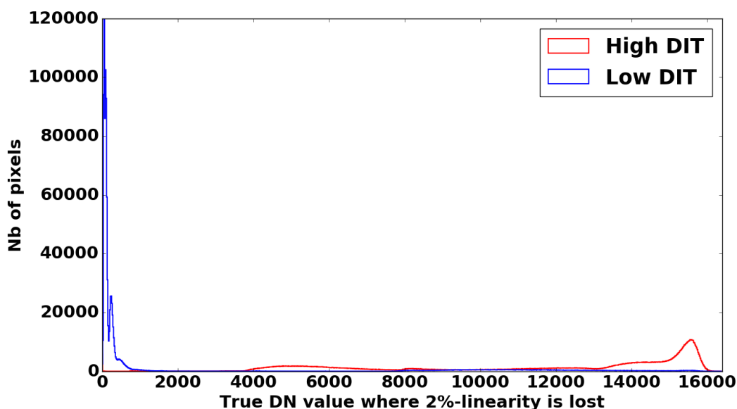
Fig. 3.21. : Histogramme du premier niveau auquel le critère de linéarité à 2% n'est plus respecté pour les temps de pose élevés (rouge) et faibles (bleu), ici pour un détecteur à 86 K.
