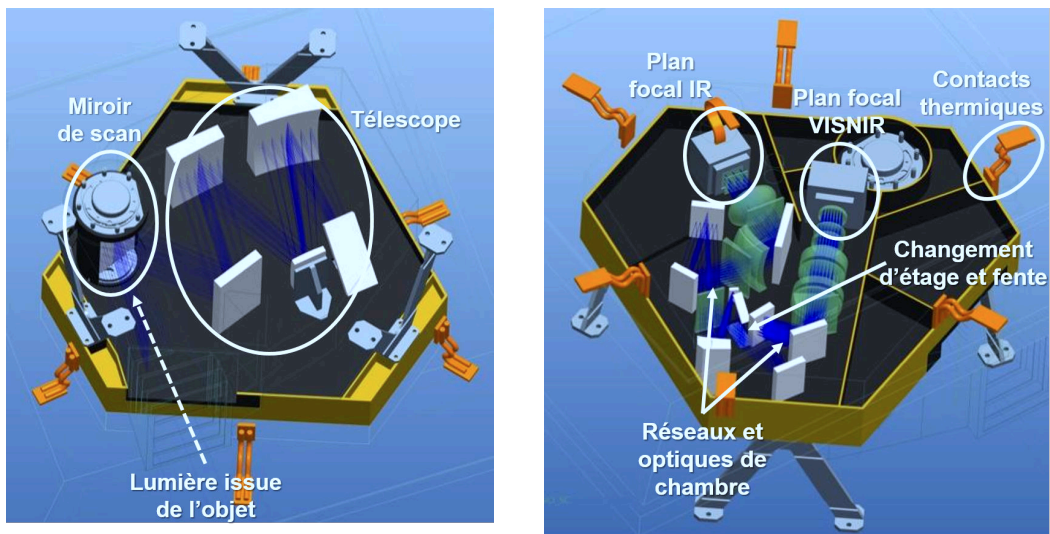
(a) Modèle opto-mécanique de l'étage du télescope de MAJIS. (b) Modèle opto-mécanique de l'étage du spectromètre de MAJIS.
