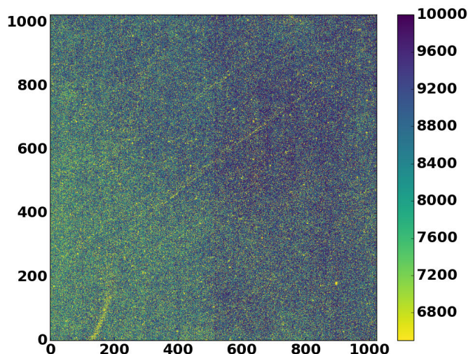
Fig. 3.24. : Image moyenne obtenue avec un flux lumineux en bande spectrale étroite dans BIRD en configuration 2 avec un détecteur à 80 K.
