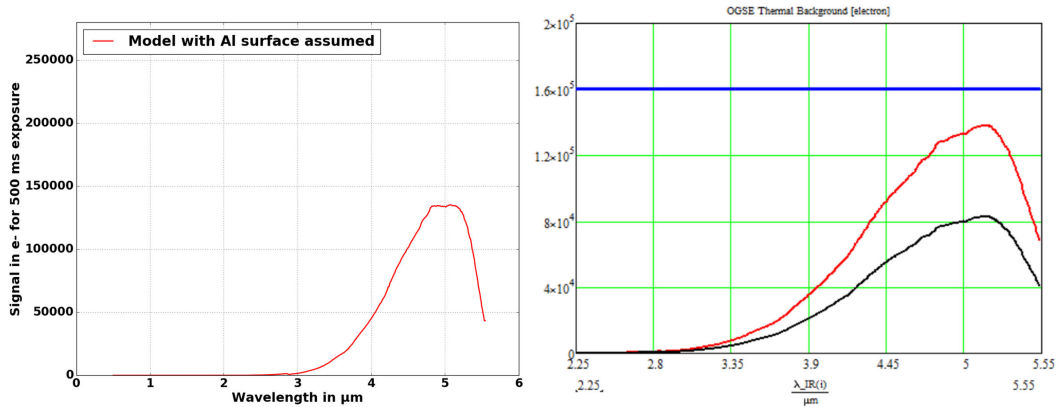
Fig. 5.2. : Comparaison entre le modèle présenté ici du signal vu par MAJIS à gauche, et celui de Leonardo Company qui fournit la partie optique de l'instrument à droite. Pour les deux figures l'échelle des abscisses est en microns et les ordonnées en électrons. Le temps de pose utilisé pour les courbes rouge est de 500 ms (courbe noire : 300 ms), la surface émettrice est de l'aluminium non poli ( \varepsilon = 7\% ) dont le flux thermique est supposé transmis à 50 %. Figure de droite réalisée par Alessandra Barbis
