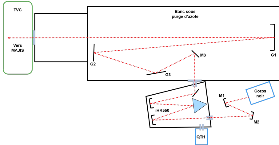
Fig. 5.32. : Schéma de la voie d'étalonnage spectral et spatial de MAJIS.
