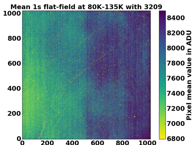
Fig. 3.23. : Image moyenne obtenue avec un flux lumineux dans Vénus en configuration 1 avec un détecteur à 80 K.
