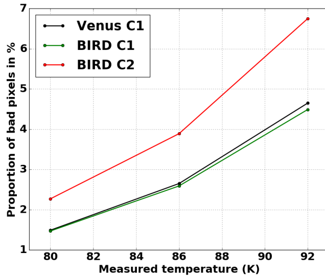
Fig. 3.13. : Proportions de pixels défectueux d’après la méthode des pixels chauds, pour trois températures et sur les trois configurations étudiées. Les mesures Venus C1 datent de mars 2017, Bird C1 de mai 2017 et Bird C2 de juillet 2018.
