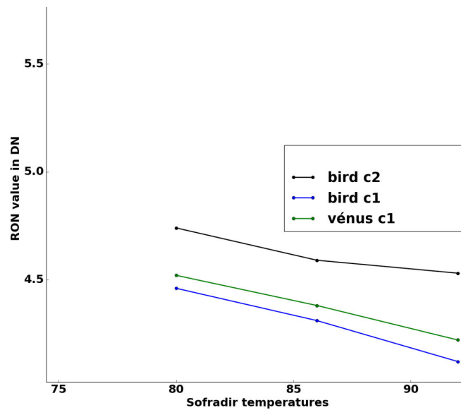
Fig. 3.15. : Évolution du RON avec la température dans chacune des configurations.
