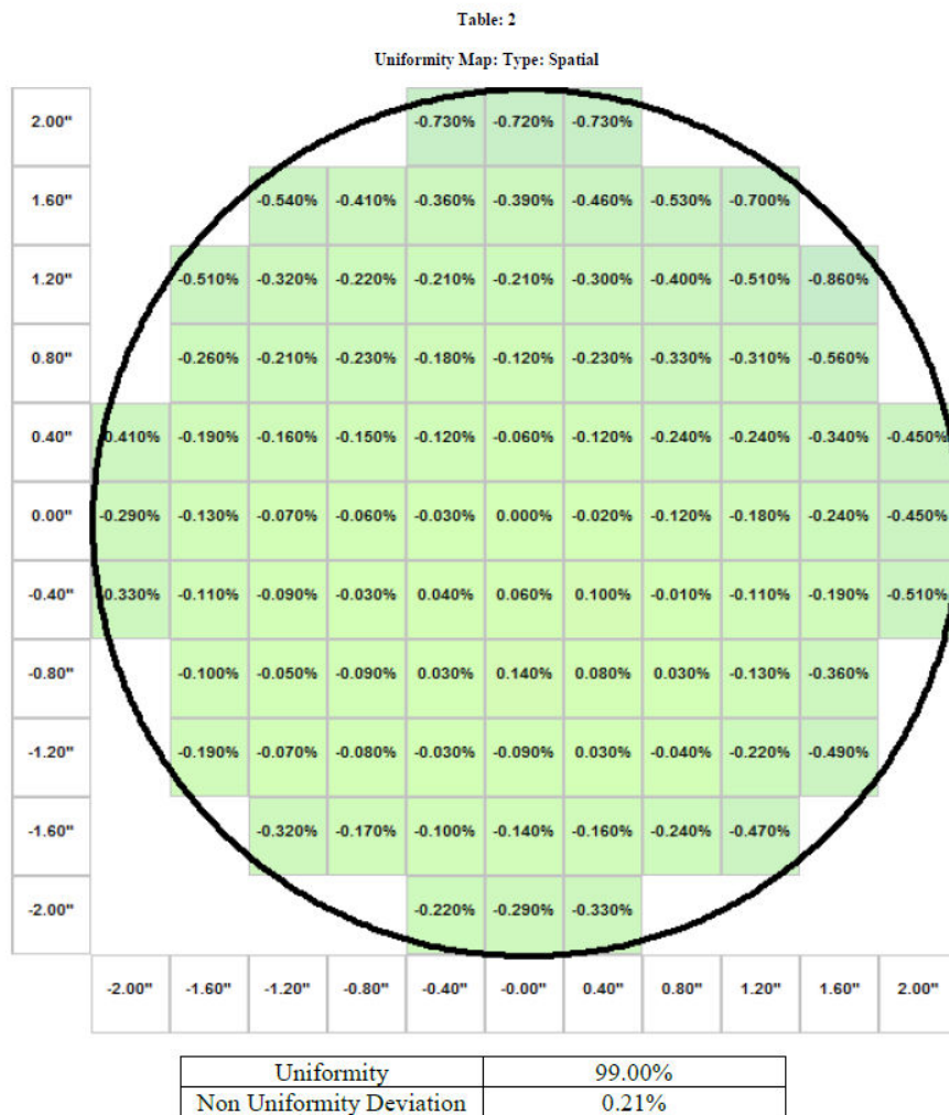
Fig. 5.15. : Écart relatif spatial en terme de flux par rapport au centre de la sortie de sphère intégrante, mesuré par Labsphere avant livraison de la source. Les pas spatiaux sont indiqués en pouces. Figure réalisée par Labsphere
