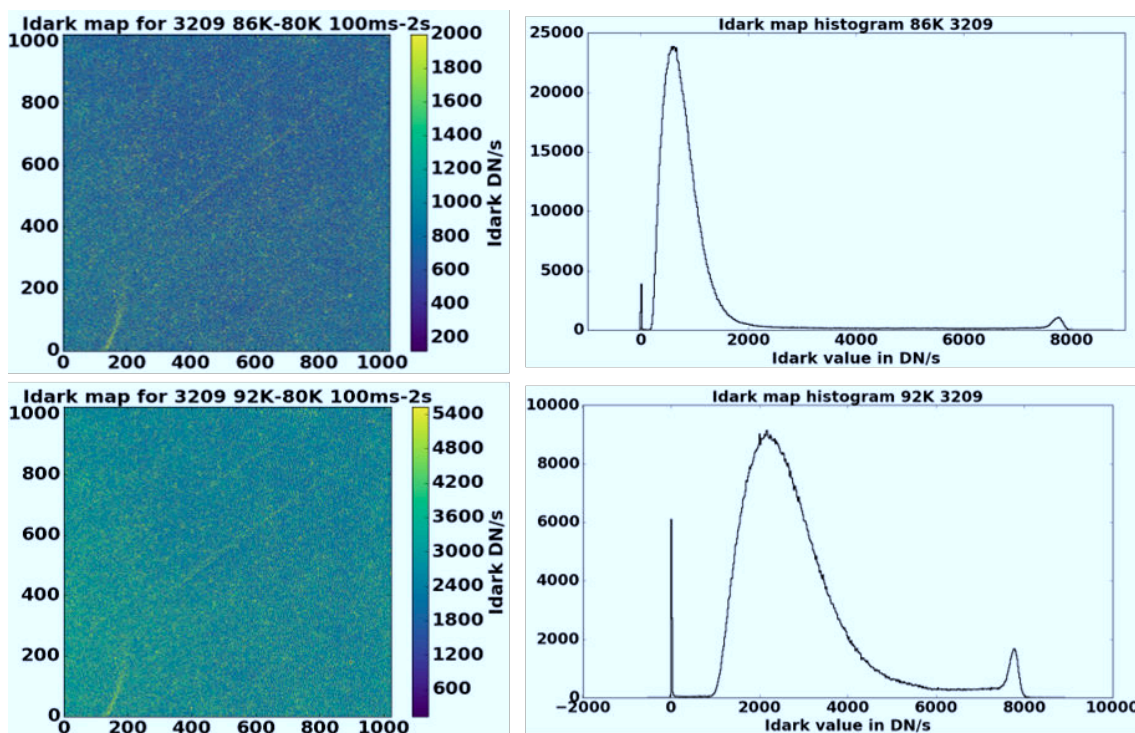
Fig. 3.17. : Évolution des cartes de courant d'obscurité par unité de temps et de leurs histogrammes en fonction de la température du détecteur : 86 K en haut et 92 K en bas.
