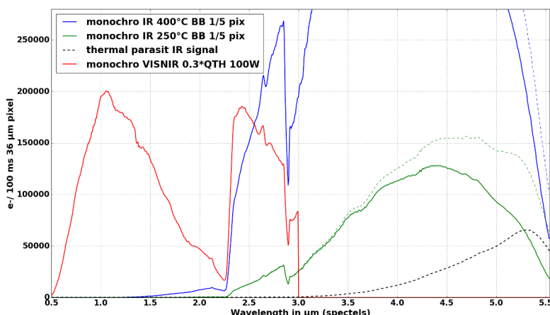
Fig. 5.26. : Flux attendus sur les détecteurs de MAJIS en fonction de la longueur d'onde dans les conditions proposées de l'étalonnage spectral.
