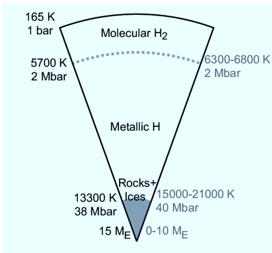
Fig. 1.7. : Schéma de la structure interne de Jupiter issu de Fortney et al. (2009), en fonction de la pression et de la température, des indications de composition chimique sont données et la masse du cœur est estimée en masses terrestres. Les valeurs à droite du schéma sont celles de Guillot (2005) tandis que celle à gauche sont de Militzer et al. (2008).
