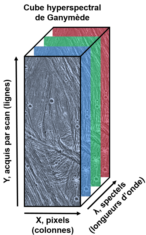
Fig. 1.16. : Schéma décrivant le contenu du cube de données final acquis par un spectro-imageur comme MAJIS avec ses deux dimensions spatiales X et Y (image) et sa dimensions spectrale \lambda (spectre de chaque pixel). Ici l'image de la surface de Ganymède est acquise par l'instrument SSI sur Galileo ( Image NASA/JPL ).
