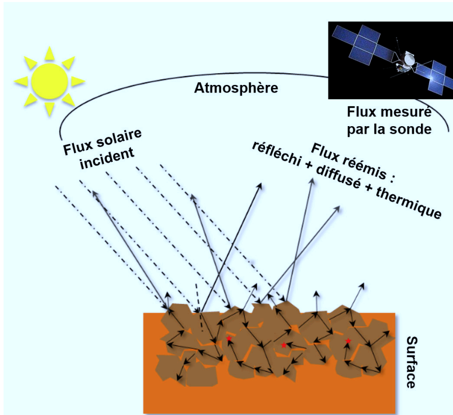
Fig. 1.19. : Schéma représentant les différentes contributions au spectre lumineux observé par une sonde pour une surface éclairée par le Soleil et possédant une atmosphère. Figure adaptée de Ody (2012)
