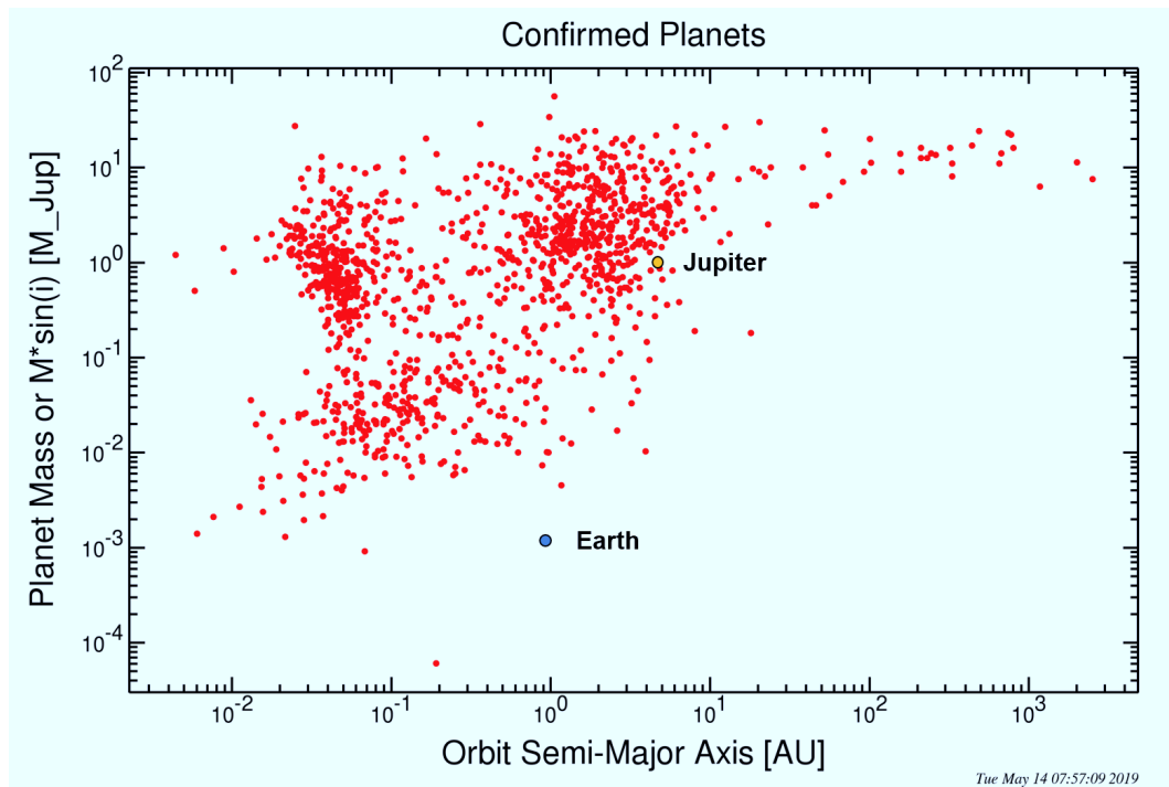
Fig. 1.11. : Masse (en masses joviennes) en fonction du demi-grand axe (en UA) des exoplanètes dont la détection est confirmée en mai 2019. Données issues de NASA Exoplanet Archive .
