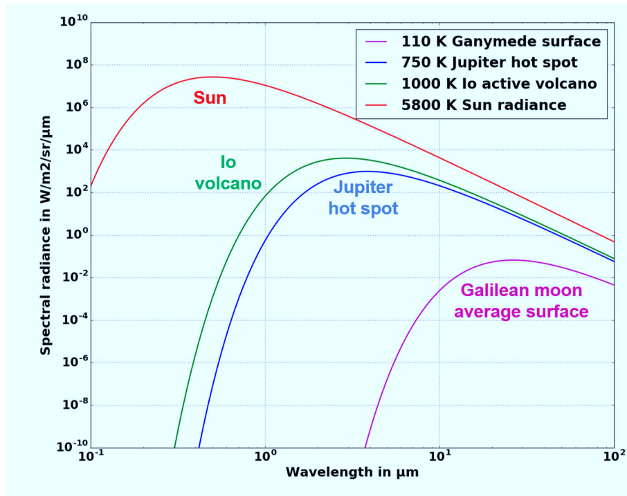
Fig. 1.18. : Radiance spectrale d'un corps noir à la température de quelques objets caractéristiques du système jovien, et radiance solaire.
