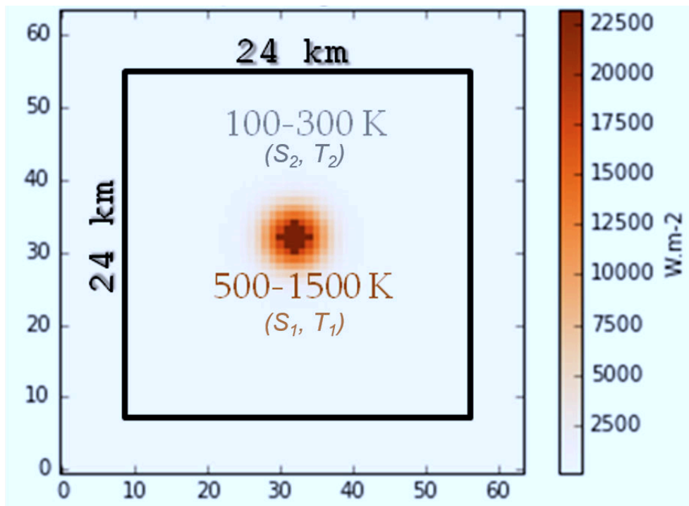
Fig. 2.5. : Modèle de surface avec un point chaud à 800K au centre, un gradient exponentiel, et une surface environnante à 200K. Le carré noir représente la taille d'un pixel et donc la surface d'intégration pour les calculs de puissance totale.
