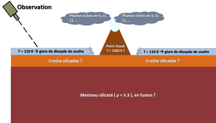
Fig. 2.3. : Schéma illustrant les hypothèses de notre recherche de silicates à la surface d'Io : leurs signatures spectrales cachées par le givre de dioxyde de soufre doivent être exposées directement à proximité des points chauds où la température de surface est suffisante pour sublimer ce givre.
