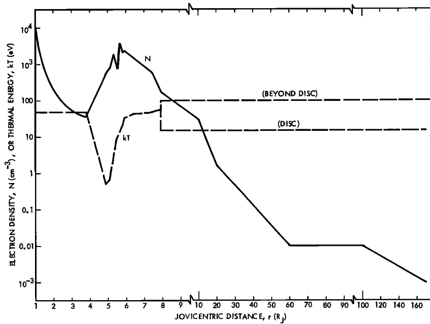
Fig. 4.2. : Évolution radiale modélisée de la densité et de l'énergie thermique des électrons dans le plasma de la magnétosphère de Jupiter e.g. Divine and Garrett, 1983 .
