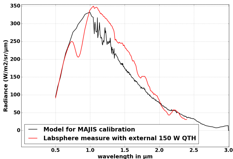
Fig. 5.18. : Radiance spectrale à la sortie de la sphère intégrante, modélisée pour répondre aux besoins de MAJIS en noir, et mesurée par Labsphere avant livraison à l'IAS en rouge.
