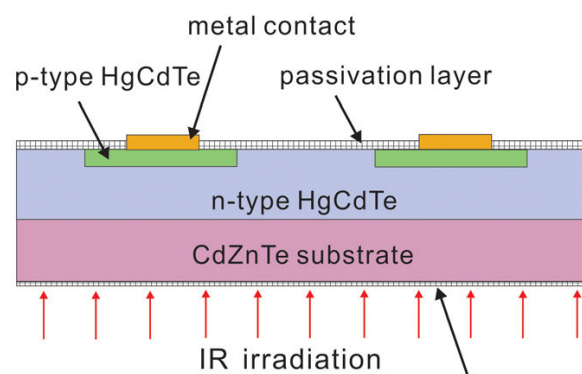
Fig. 3.2. : Schéma de la structure de deux pixels de détecteur CMOS HgCdTe dopé p sur n, similaire aux détecteurs de vol H1RG de MAJIS. Ici le substrat de CdZnTe sur lequel croît le cristal semi-conducteur n'est pas retiré, contrairement aux H1RG. Schéma issu de Lei et al. (2015)
