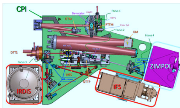
(b) Modèle optique de SPHERE, la voie que nous utilisons ici est l'Integral Field Spectrometer (IFS).
