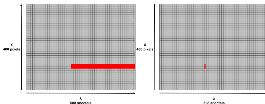
Fig. 5.33. : Schéma des images attendues pour les mesures de PSF spatiale à gauche et de PSF spectrale à droite, avec la source infrarouge. Ici le détecteur est représenté à l'échelle 1/10 ème, les spectels les plus à gauche correspondent à 2.25 \mu\text{m} de longueur d'onde et ceux les plus à droite à 5.54 \mu\text{m} .
