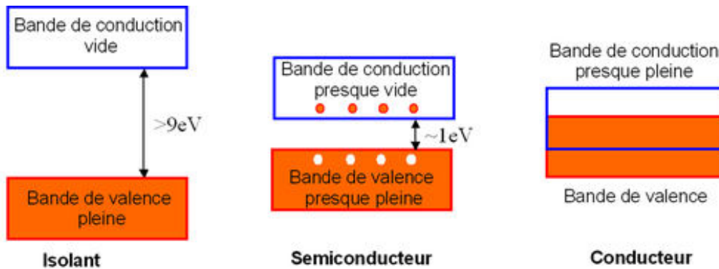
Fig. 3.1. : Niveaux d'énergie hauts dans des matériaux isolants, semi-conducteurs et conducteurs
