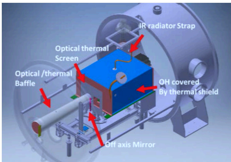
Fig. 5.8. : Représentation 3D de la cuve à vide Jupiter et de son aménagement intérieur prévu pour accueillir MAJIS durant son étalonnage. Figure réalisée par J. Barbay
