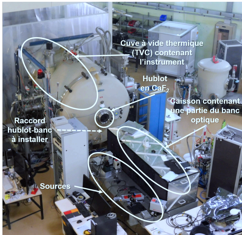
Fig. 5.11. : Photo du dispositif d'étalonnage en cours de développement dans le hall blanc dédié. Au premier plan de la photo se trouveront la plupart des sources de lumière ainsi que leur contrôle-commande, tandis que les optiques sont situées dans le caisson noir prévu pour être purgé à l'azote. Puis un raccordement avec le hublot d'entrée dans la TVC sera installé, et on voit au second plan la cuve qui accueillera MAJIS.
