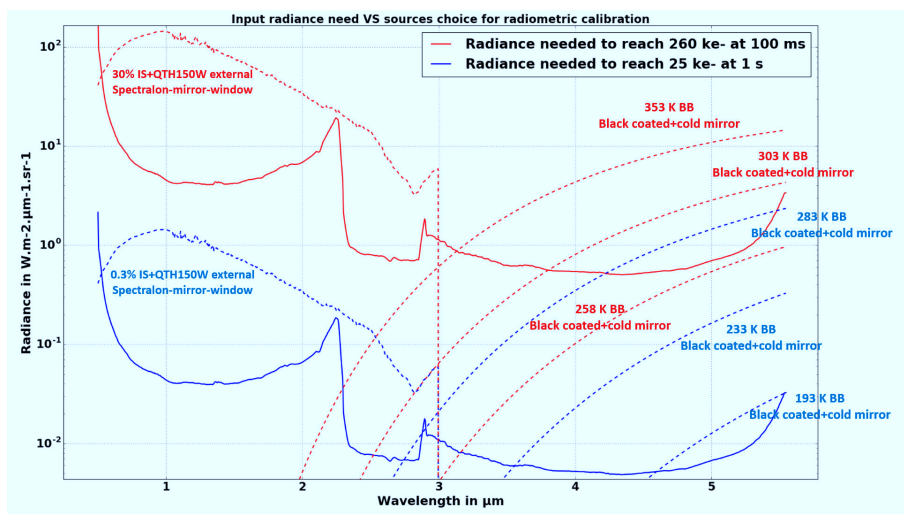
Fig. 5.17. : Besoin en flux maximal (rouge) et minimal (bleu) pour l'étalonnage radiométrique absolu. Les courbes pointillées correspondent à des configurations des deux sources d'OP3 et OP4 (sphère intégrante et corps noir froid) permettant de répondre à ces besoins.
