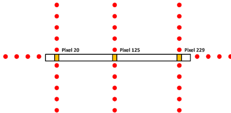
Fig. 5.34. : Positions du faisceau de lumière issu des sources en rouge, correspondantes aux déplacements de l'hexapode autour de la fente d'entrée représentée par le rectangle central. La lumière parasite est ainsi mesurée dans les deux directions par rapport à la fente, pour quelques pixels spatiaux représentés comme exemples par les carrés oranges.
