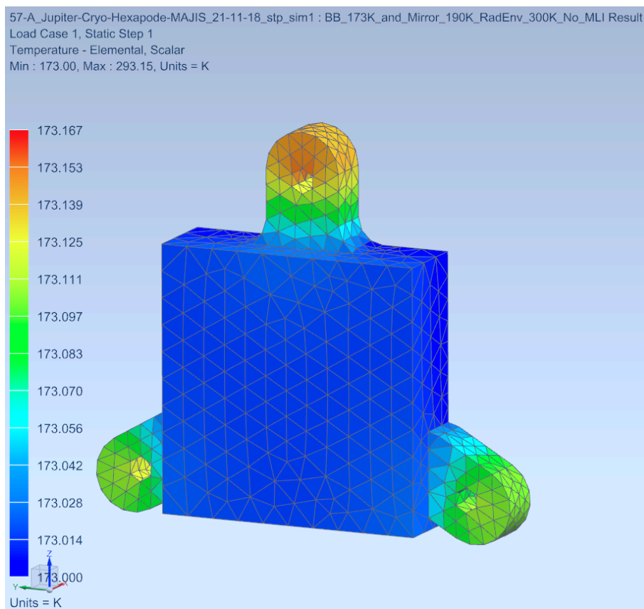
Fig. 5.24. : Modèle thermo-mécanique du corps noir source situé à l'intérieur de la cuve à vide avec sa régulation thermique : l'échelle de couleur code les inhomogénéités de température, on constate qu'elles sont inférieures à 0.1 K sur la surface émissive, ce qui correspond au besoin d'homogénéité spatiale comme vérifié dans le texte. Figure réalisée par J.C. Le Clec'h
