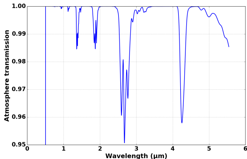
Fig. 5.7. : Transmission de la même colonne d'air qu'en Figure 5.5, convoluée à la résolution spectrale de MAJIS, en supposant une purge à l'azote sec permettant d'atteindre 1 % d'hygrométrie dans les mêmes conditions de température et de pression.
