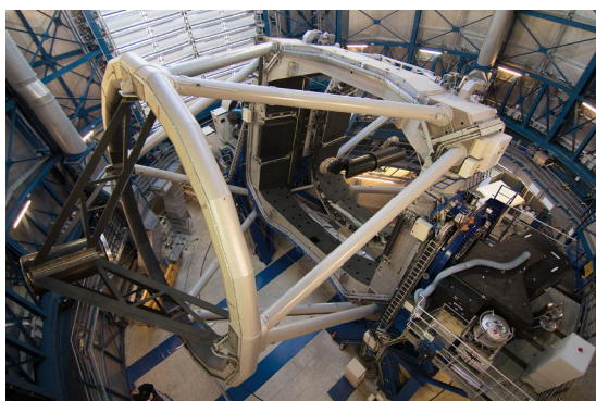
(a) L'UT3 du VLT avec l'instrument SPHERE sur sa plate-forme Nasmyth à droite.
