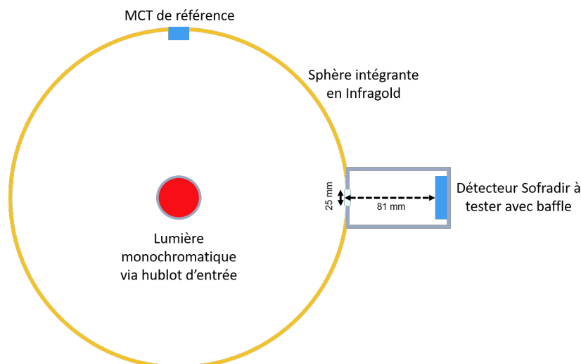
Fig. 3.28. : Schéma de la sphère intégrante placée dans la cuve à vide en configuration 2. Le hublot d'entrée du flux lumineux issu du monochromateur est situé en retrait par rapport au plan du schéma.
