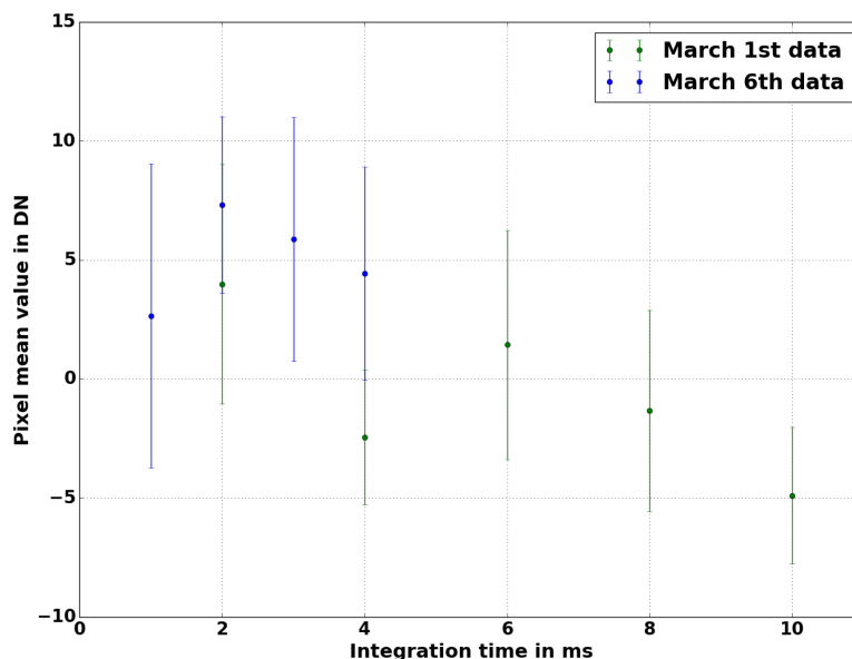
Fig. 3.10. : Variabilité des mesures à faible temps d'intégration : les points verts sont acquis le 1er mars, les points bleu le sont le 6 mars, sur le même pixel 589 :855, à la même température de détecteur et dans les même conditions. Chaque point est moyenné sur dix acquisitions, les barres d'erreur représentent l'écart-type sur ces dix acquisitions.
