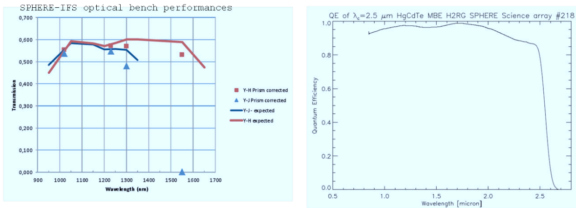
(a) Transmission théorique et mesurée du banc optique de SPHERE, selon la configuration spectrale choisie. (b) Efficacité quantique mesurée du détecteur Hawaii de SPHERE.
