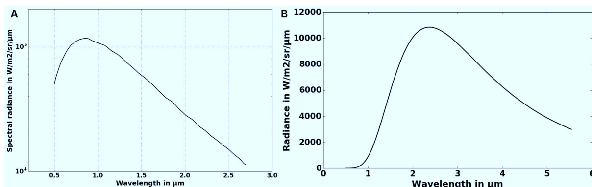
Fig. 5.13. : A : radiance spectrale de la lampe QTH 100 W fournie par Newport utilisée comme source VISNIR du monochromateur. B : radiance spectrale du corps noir CIsystems SR-200 32 utilisé comme source infrarouge du monochromateur, ici chauffé à 950^\circ C avec une émissivité de 97 %.
