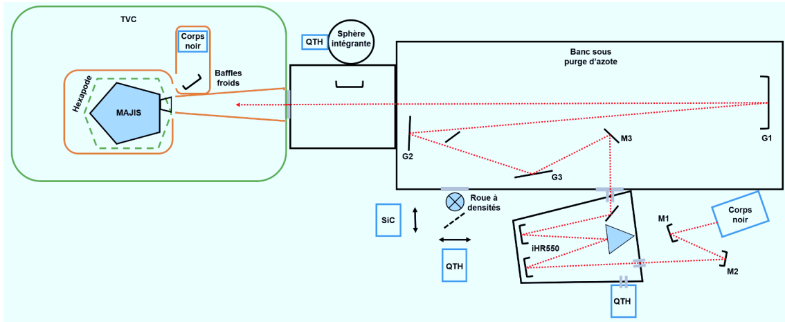
Fig. 5.40. : Schéma complet des voies optiques d'étalonnage de MAJIS avec leurs sources.
