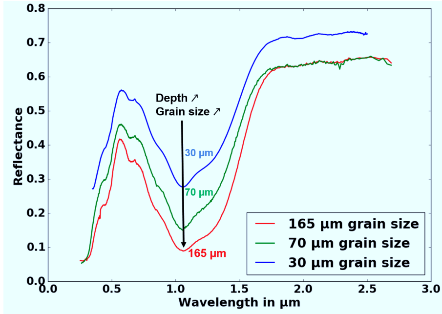
Fig. 1.20. : Spectres de réflectance de grains de l'olivine (silicate) illustrant l'influence de la taille des grains, de 30 à 165 \mu\text{m} , sur la profondeur des bandes d'absorption par rapport au continuum. Données issues de l'USGS Spectral Library (Kokaly et al., 2017).
