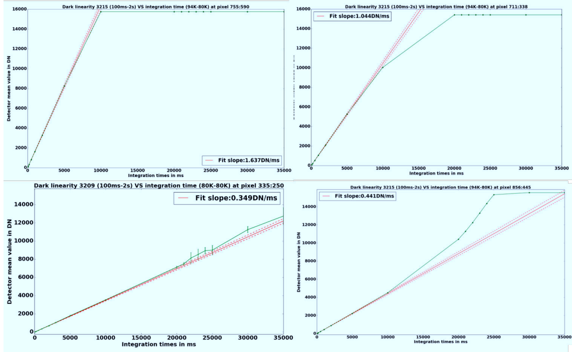
Fig. 3.22. : Exemples de comportements de pixels s'éloignant de la linéarité de façon inattendue.
