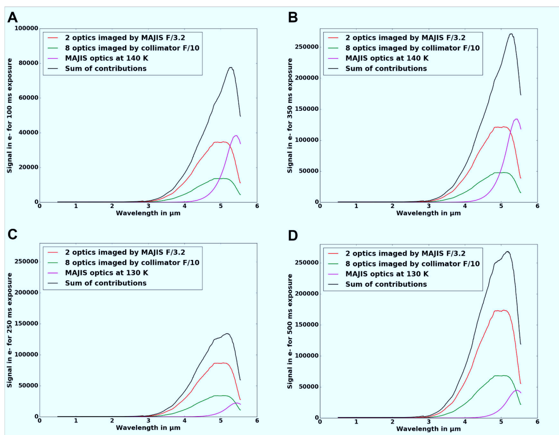
Fig. 5.4. : Signal sur les détecteurs de MAJIS, en électrons, dû au seul rayonnement thermique de l'environnement : en violet la modélisation de l'optique de MAJIS à 140 K en A et B, à 130 K en C et D. En vert, la contribution de 8 dioptries à 3 % d'émissivité et 97 % de transmission chacun imagés par le collimateur ( F/D = 10 ) du banc optique, en rouge même contribution pour seulement 2 dioptries imagés par MAJIS ( F/D = 3.2 ). En noir, la somme de ces trois contributions typiques d'une observation de source placée en entrée du banc optique.
