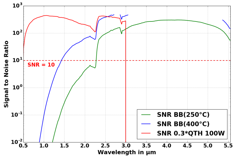
Fig. 5.27. : SNR attendu sur les détecteurs de MAJIS en fonction de la longueur d'onde dans les conditions proposées de l'étalonnage spectral.
