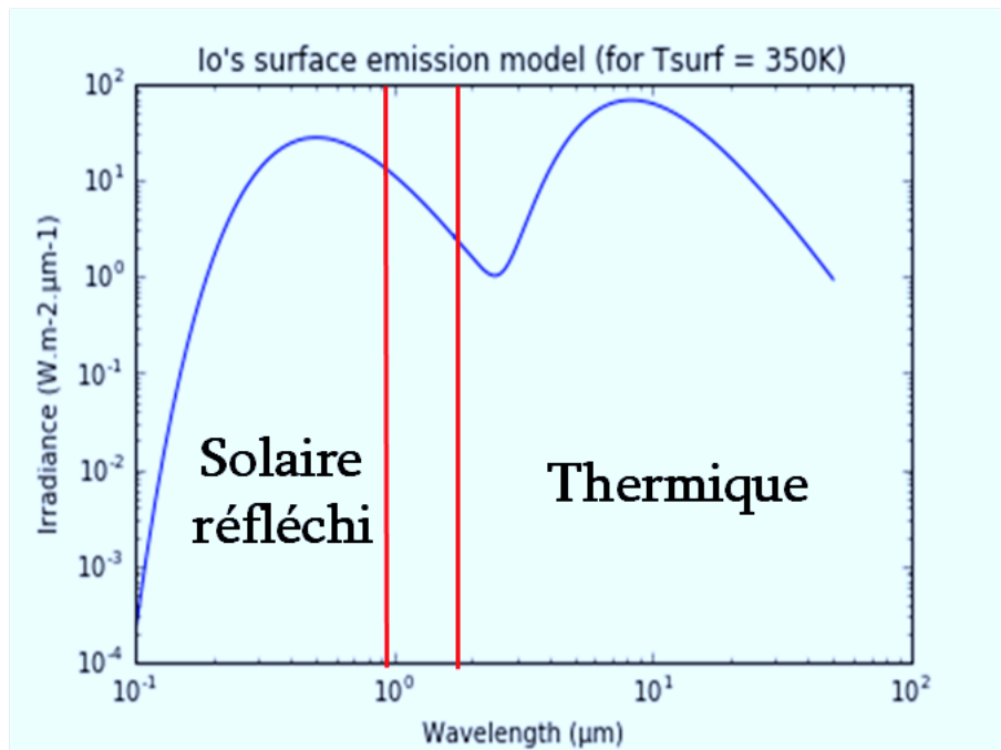
Fig. 2.4. : Modèle de l'émission de corps noir de Io : partie solaire réfléchi à gauche avec un albédo de 0.6 et partie thermique propre à droite pour une surface à 350K. La gamme spectrale de nos données se trouve entre les traits rouges.
