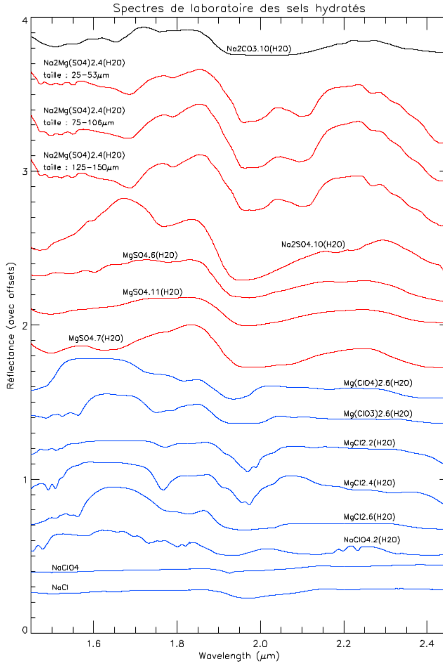
Fig. 1.23. : Spectres de réflectance (translatés) de plusieurs sels hydratés de magnésium, de sodium et de chlore dont la présence est suspectée sur Europe, d'après Ligier (2016) . Données issues de Dalton & Pitman (2012) , McCord et al. (2001b) et Hanley et al. (2014) .
