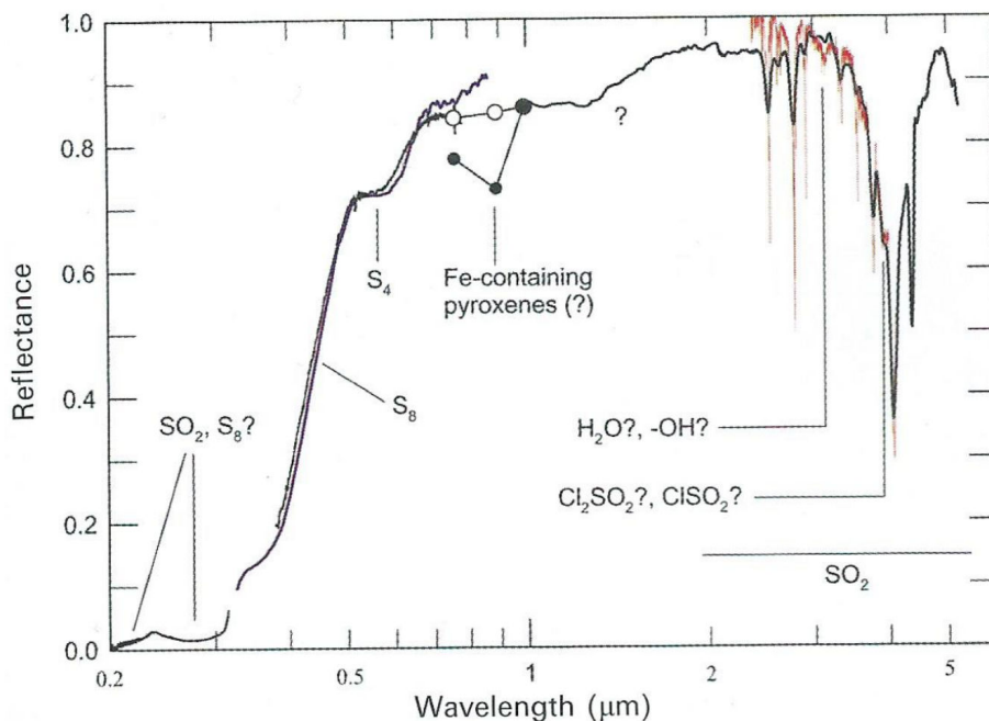
Fig. 1.5. : Spectre visible et infrarouge en réflectance de la surface d'Io : assemblé par Carlson et al. (2007) à partir de données issues de Galileo/NIMS/SSI, d'ISO, et d'observations au sol. Les signatures spectrales sont attribuées lorsqu'elles ne font pas débat, les signatures autour de 1 \mu\text{m} peuvent être attribuées à des minéraux silicatés mais leur détection n'est pas confirmée.
