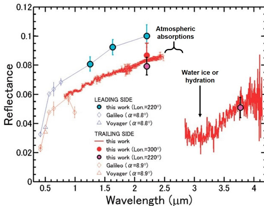
Fig. 1.9. : Spectre infrarouge en réflectance du satellite irrégulier Amalthée, obtenu avec le télescope Subaru par Takato et al. (2004), comparé à d'autres jeux de données. La partie du spectre autour de 2.7 \mu\text{m} est parasitée par l'absorption de l'atmosphère terrestre due à l'eau. La seule signature spectrale détectée sans ambiguïté est l'absorption à 3 \mu\text{m} discutée dans le texte.
