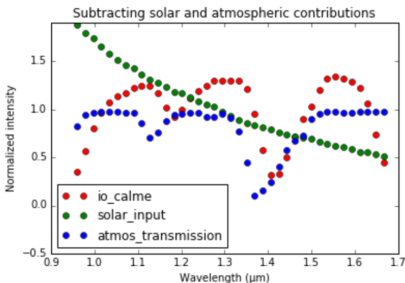
Fig. 2.11. : Spectre de Io par SPHERE dans une zone exempte de structures spatiales en rouge, spectre atmosphérique convolué à la résolution spectrale de SPHERE en bleu, et spectre solaire mesuré en vert. Tous ces spectres sont divisés par leur valeur moyenne pour les rendre comparables.
