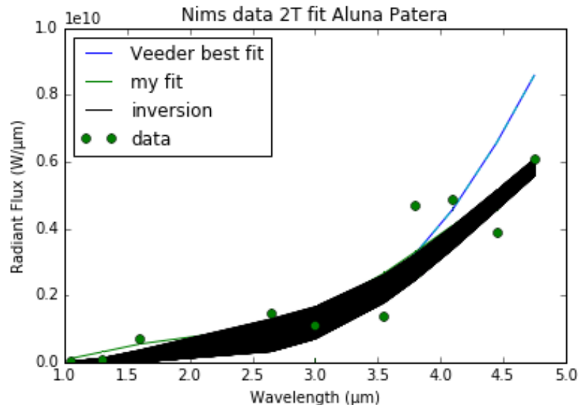
Fig. 2.10. : Ce graphique est le même que celui de la Figure 2.6. Le faisceau de courbes noires représente les solutions de RMS minimum en laissant la température du point central varier avec une amplitude de 250K.
