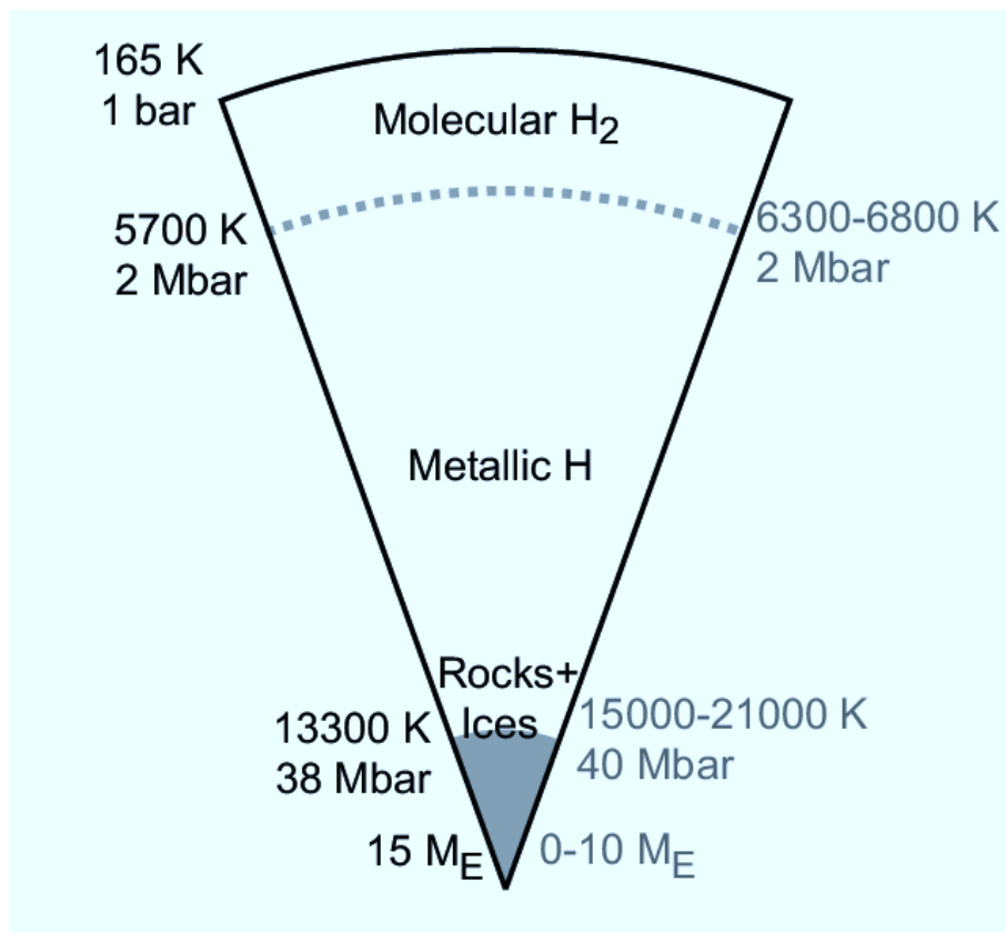
Fig. 1.7. : Schéma de la structure interne de Jupiter issu de Fortney et al. (2009), en fonction de la pression et de la température, des indications de composition chimique sont données et la masse du cœur est estimée en masses terrestres. Les valeurs à droite du schéma sont celles de Guillot (2005) tandis que celle à gauche sont de Militzer et al. (2008).
