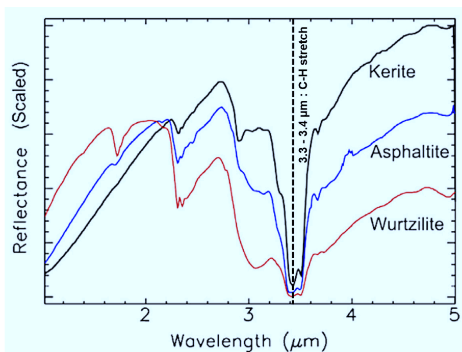
Fig. 1.24. : Spectres de composés organiques illustrant l'absorption à 3.4 \mu\text{m} par étirement des liaisons C-H, utilisés pour l'interprétation spectrale des résultats de Dawn sur Cérès. Figure issue de Combe et al. (2019) et données de Moroz et al. (1998).
