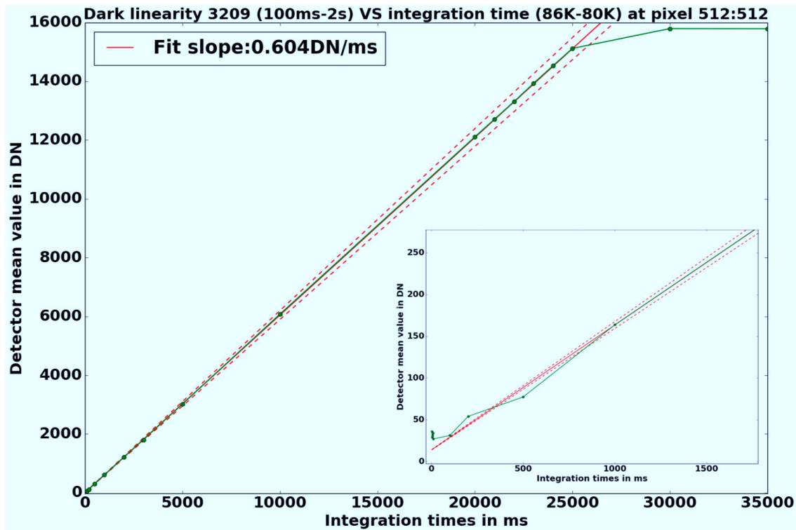
Fig. 3.16. : Ajustement linéaire des valeurs de courant d'obscurité d'un pixel en fonction du temps de pose, avec un zoom sur les temps de pose faibles.
