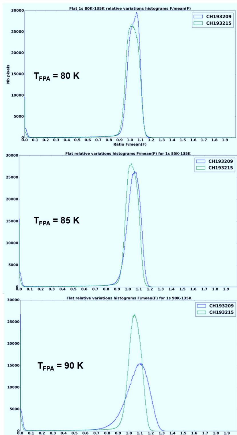
Fig. 3.26. : Évolution de l'histogramme des variations relatives du Flat pour deux détecteurs en fonction de leur température.
