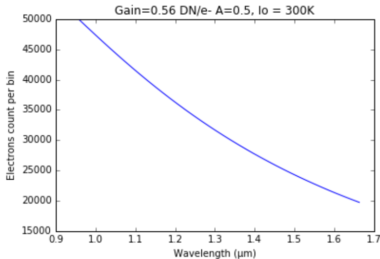
Fig. 2.8. : Nombre d'électrons attendus dans le détecteur d'après mon modèle instrumental et avec mon modèle thermique d'émission de Io en entrée. On attend par exemple pour une image à 1.3 \mu\text{m} : 32000 \cdot 0.56 = 18000 DN.
