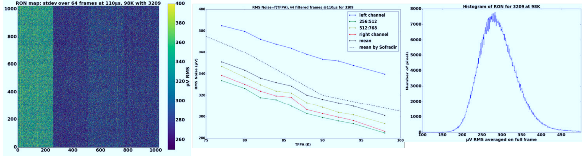
Fig. 3.14. : Mesures de bruit de lecture : la première colonne donne la carte de RON en \mu V mesuré pour une température détecteur de 98 K, la seconde donne l'évolution des valeurs de ce RON en fonction de la température pour chacun des quatre canaux vidéos, et la troisième donne l'histogramme des cartes.
