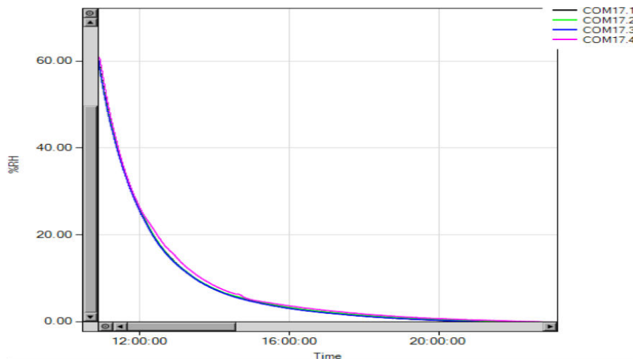
Fig. 5.6. : Évolution du taux d'humidité à l'intérieur du caisson optique au cours du temps, en heures, pour quatre capteurs d'humidité placés à quatre endroits différents à l'intérieur, lorsqu'un débit d'azote gaz de 20 l/min est appliqué à une extrémité du banc. Figure réalisée par B. Lecomte
