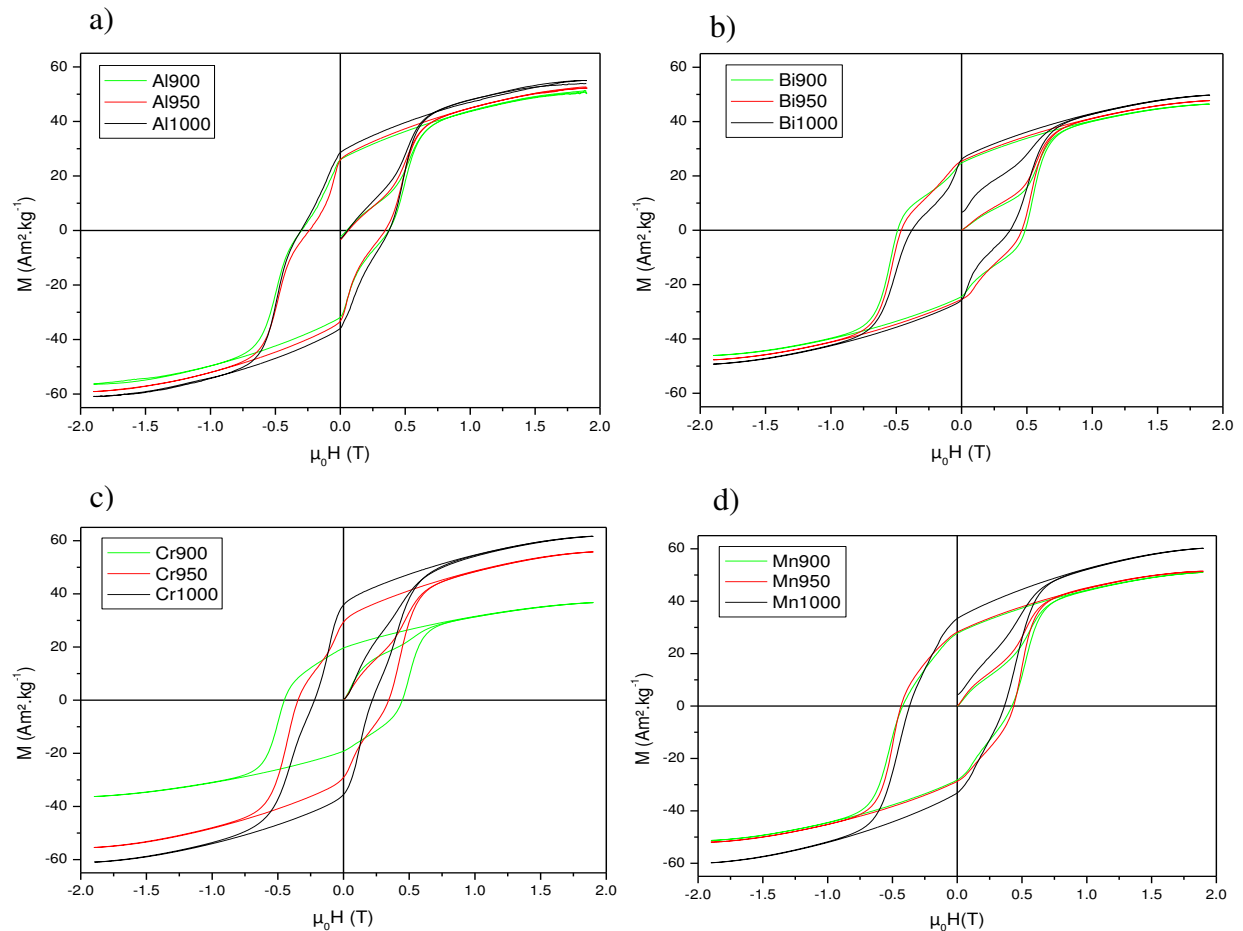
Figure III. 27. Cycles hystérésis ( M-\mu_0 H ) de a) \text{BaAlFe}_{11}\text{O}_{19} , b) \text{BaBiFe}_{11}\text{O}_{19} , c) \text{BaCrFe}_{11}\text{O}_{19} et d) \text{BaMnFe}_{11}\text{O}_{19} calcinés à différentes températures
