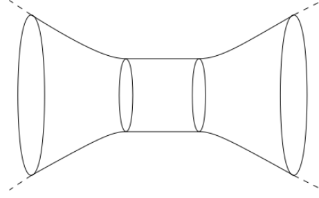
FIGURE 1.4 – Le plongement d'un cylindre euclidien prévient la s -injectivité de I_m
