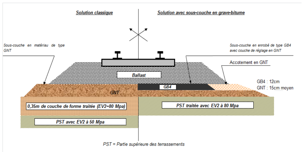
Figure II.1 – Les deux structures de la LGV BPL
