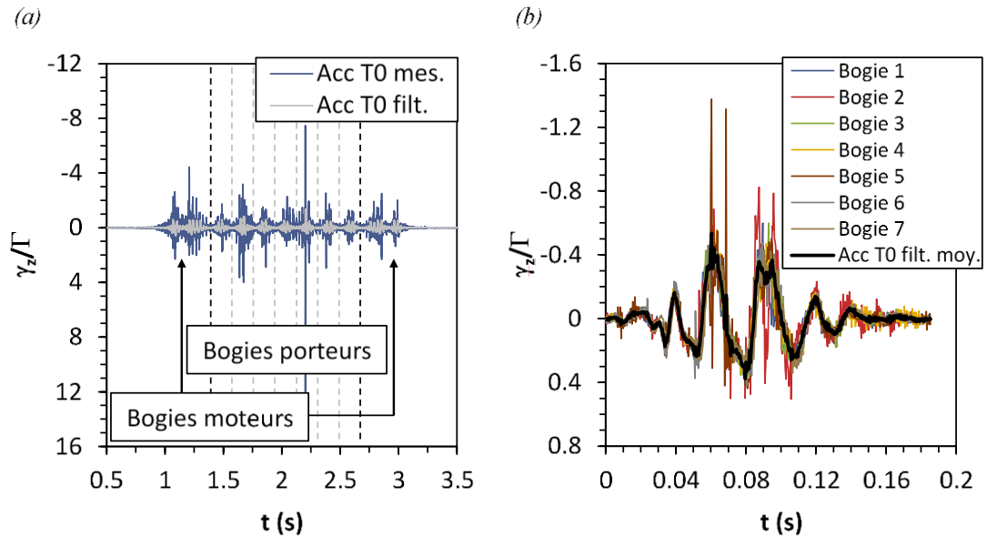
Figure I.14 - Filtrage et séquençage du signal mesuré par un capteur lors du passage d'une rame de TGV à 362 \text{ km.h}^{-1} . (b) Illustration de la méthode dite de cumul des bogies porteurs pour le passage du TGV précédent (Martin, 2014)
