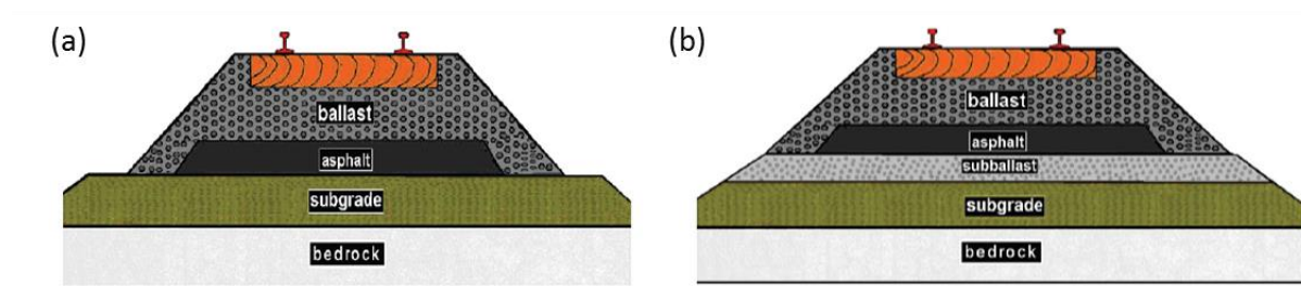
Figure I.37 – (a) Section de ligne avec GB et sans GNT (b) Section de ligne avec GB et GNT (Rose et al., 2010)
