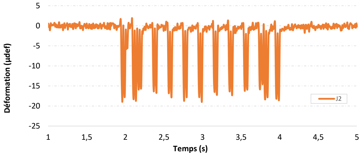
Figure III.21 - Profil temporel de déformation verticale issu de la jauge verticale placée dans la couche granulaire sous l'axe du rail externe pour le passage de train le 2 décembre 2016 à V=340 \text{ km.h}^{-1}
