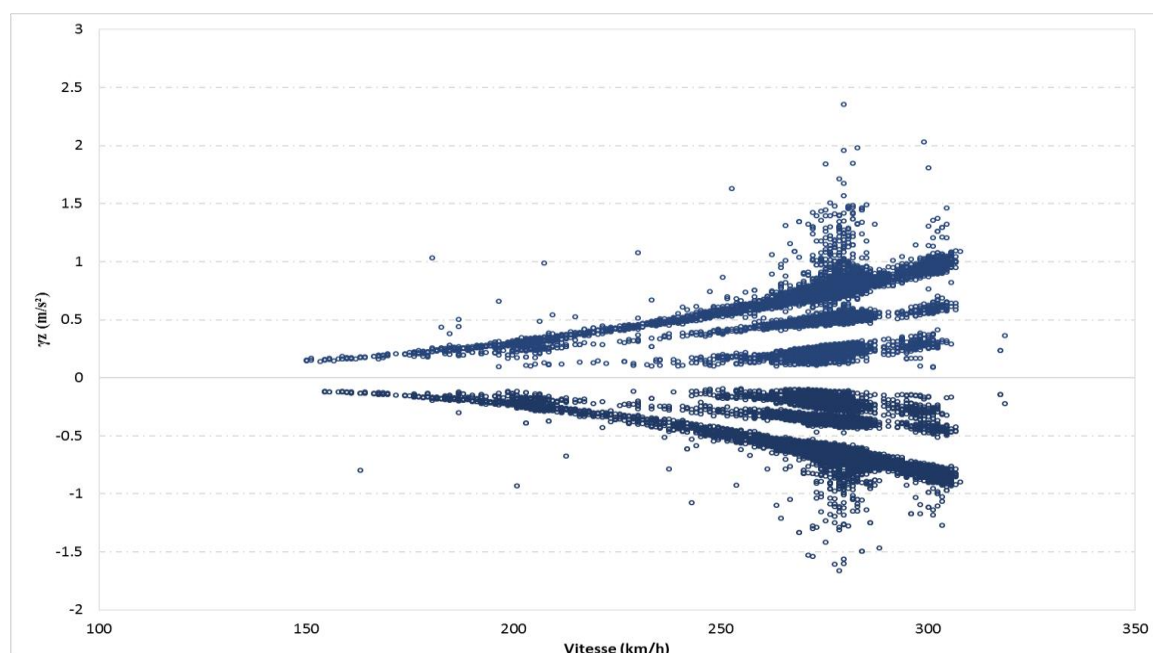
Graphique 35 - Accélérations verticales maximales et minimales mesurées par l'accéléromètre A5, situé sous l'axe du rail, sur la section bitumineuse, en fonction de la vitesse de passage des trains.
