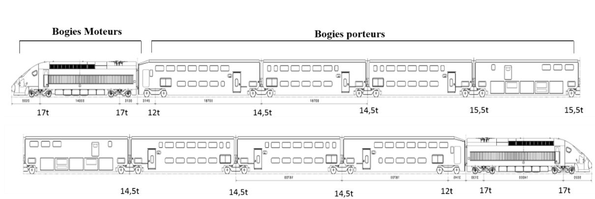
Figure III.1 - TGV de la phase de montée en vitesse
