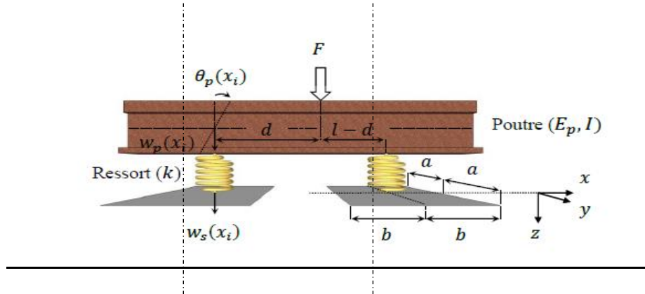
Figure VII.4 – Représentation schématique du système d'armement rail/traverse. Décomposition en segment périodique figuré entre les deux lignes pointillées (Martin, 2014).
