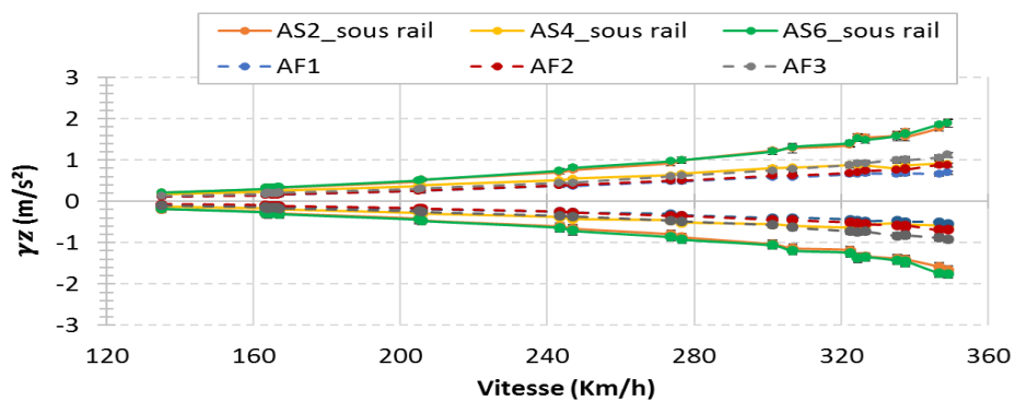
Graphique 3 - Comparaison entre les accélérations verticales maximales positives et négatives en fonction de la vitesse, des accéléromètres au sommet de la sous-couche granulaire installés sous l'axe du rail et ceux à la base, pour les passages de train dans le sens 2 sur la section 2 pendant la phase de montée en vitesse
