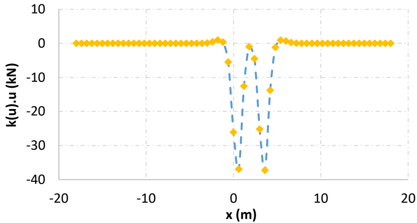
Figure VII.9 – Distribution de la force k(u).u sur les blochets pour une valeur de l'exposant \alpha=1.26 de la loi de raideur k(u) .
