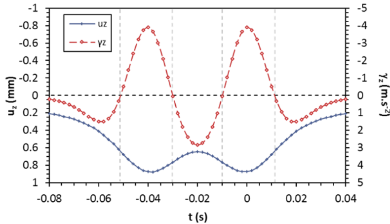
Figure I.13 - Profils temporels du déplacement vertical et de l'accélération verticale calculés au droit d'une traverse ( x=0 ) sous l'axe d'un rail ( y=0 ) et près de la surface du ballast ( z=0.05 \text{ m} ). (A. Martin, 2014)
