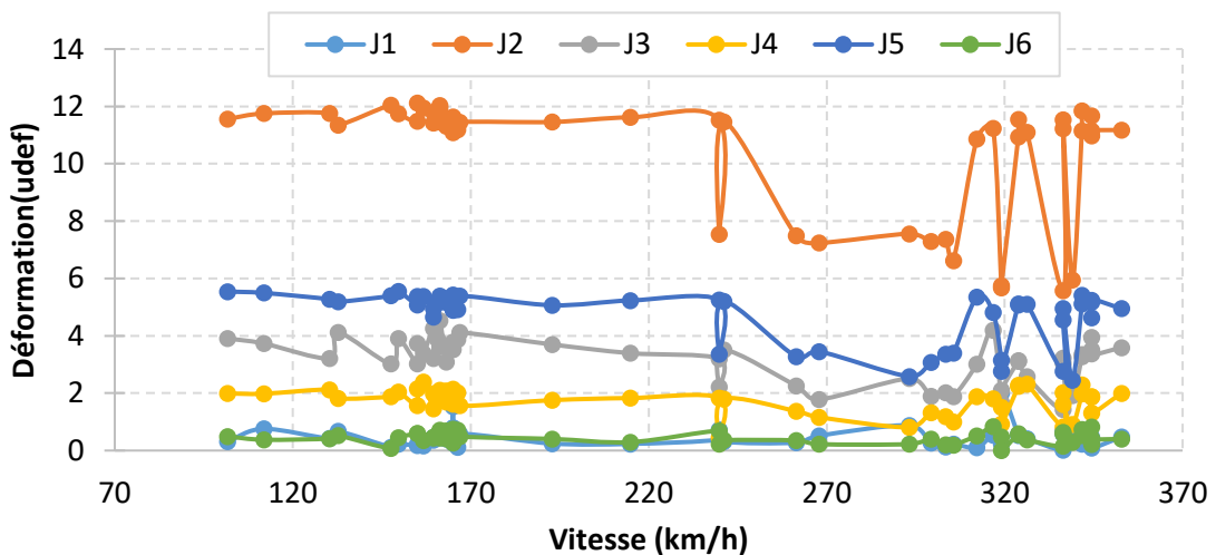
Figure III.24 - Comparaison des déformations verticales maximales en fonction de la vitesse, des jauges verticales placées dans la sous-couche granulaire, pour les passages de train sur la section 4 pendant la phase de montée en vitesse
