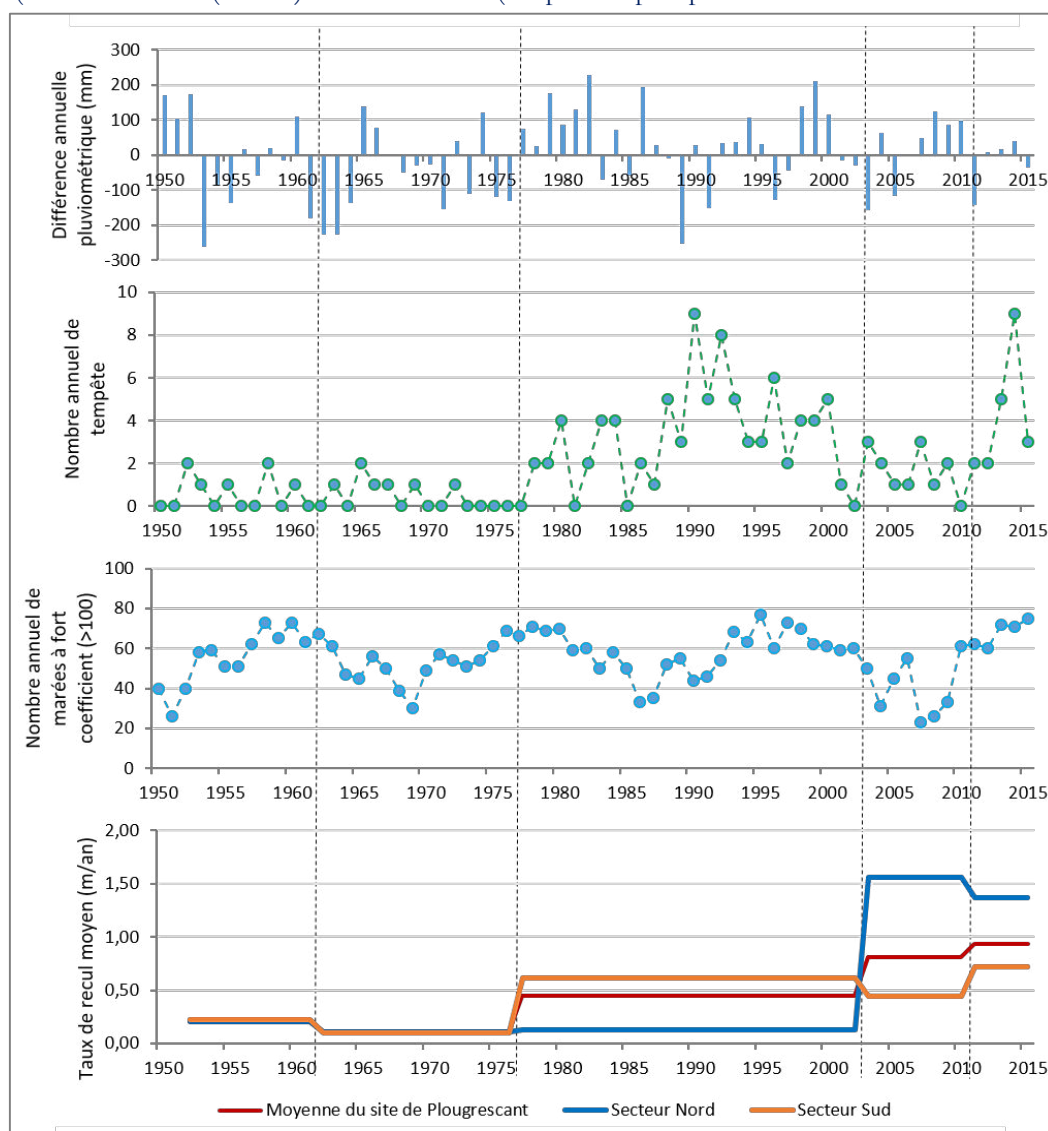
Fig. 111 : Taux de recul moyen des falaises de Pors-Hir et chroniques des conditions météo-marines entre 1950 et 2015 (sources : SHOM (marées) et Météo-France (tempêtes et précipitations à la station de l'Île-de-Bréhat)).
