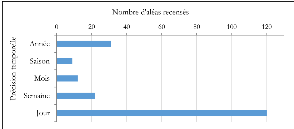
Fig. 81 : Précision temporelle des aléas d'érosion recensés.
