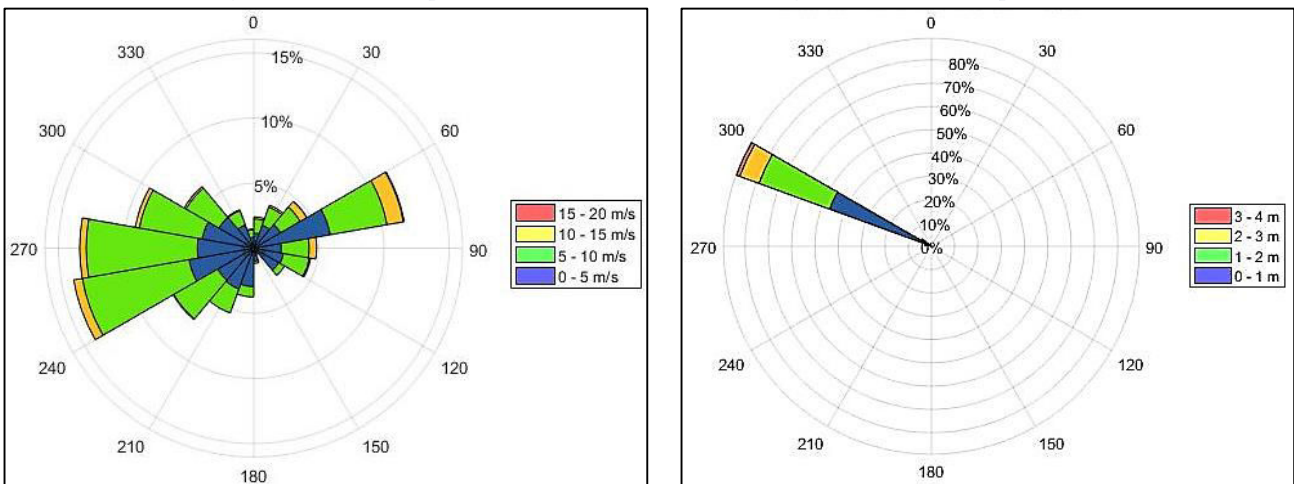
A : Rose des vents (1997-2010) à la station Météo-France de Ploumanac'h
