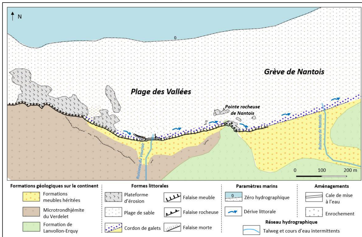
Fig. 46 : Carte géomorphologique du site de Pléneuf-Val-André.
