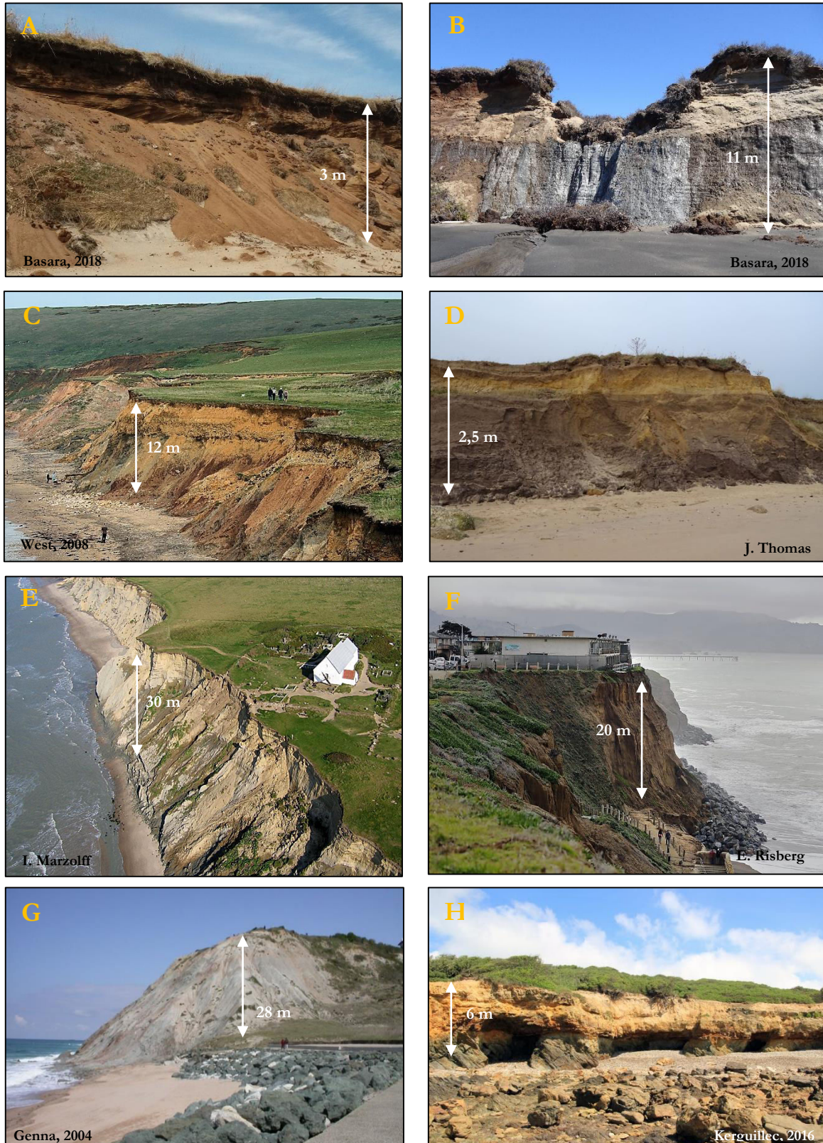
A : falaise de sable de Val-Marguerite (Québec). B : falaise de sable et de silt marin de Rivière-Saint-Jean (Québec) ; C : falaise d'alluvions pléistocènes de l'île de Wight (Royaume-Uni) ; D : falaise de sable et d'argile de Fraisthorpe (Royaume-Uni) ; E : falaise d'argile et de silt de Marup Kirke (Danemark) ; F : falaise d'alluvions et de sable de Pacifica (Californie) ; G : falaise de marne de Bidart (Pays basque, France) ; H : falaise de micaschistes altérés, surmontés de sables quaternaires à Jard-sur-Mer (côte vendéenne, France).
