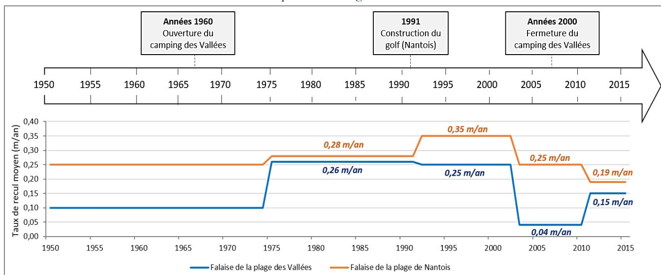
Fig. 106 : Évolution des taux de recul des falaises de la plage des Vallées et de la grève de Nantois mise en relation avec la chronique des aménagements entre 1950 et 2015.
