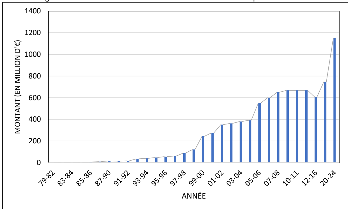
Figure 10 : Évolution du montant des droits télévisés du Championnat de France
