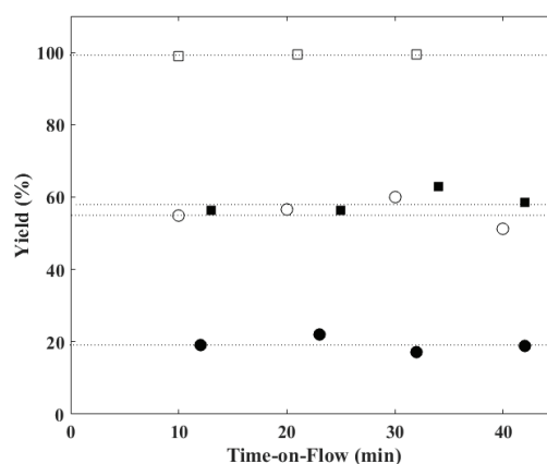
Pd (0) Strem
