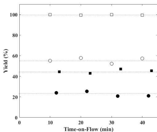
Pd(0) Siliacat
