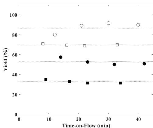
Pd(II) Siliacat
