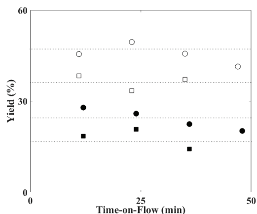
Pd/Alumina
