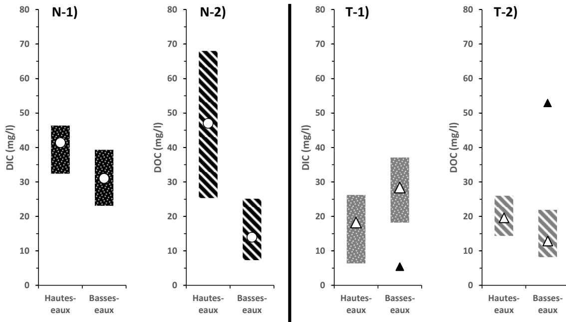
Figure III.8 : Saisonnalité des concentrations en carbone dissous inorganique (DIC, N-1 et T-1) et organique (DOC, N-2 et T-2) observées sur les sites échantillonnés à la fois en S1 (hautes-eaux) et S2 (basses-eaux) dans la Nyando (N) et la Tukela (T). Les marqueurs blancs représentent la moyenne des concentrations de la Nyando (ronds) et de la Tukela (hors 'Little Tukela at Wintertown', triangles). Les triangles noirs représentés en période de basses-eaux sur les sous-figures T-1 et T-2 représentent la concentration du site 'Little Tukela at Wintertown'.
