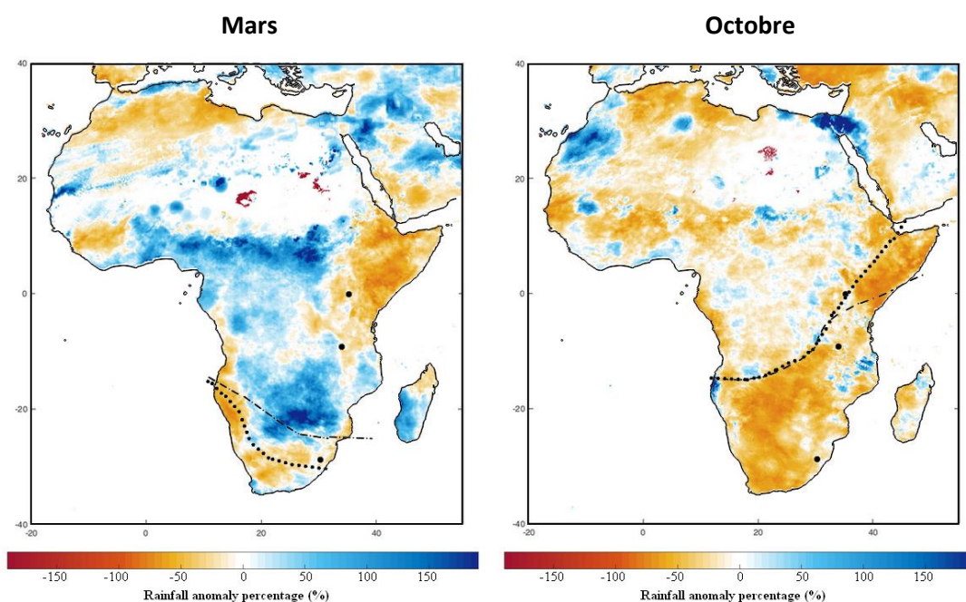
Figure 0.13 : Distribution des anomalies de pluies en mars et en octobre 2016 en Afrique, exprimées en pourcent par rapport à la moyenne mensuelle entre les années 1981 à 2017 (Funk et al., 2015; The Climate Hazards Group, 2018). La limite sud de la ZCIT est figurée par une ligne tiretée pour sa position moyenne entre 1981 et 2017 et par une ligne pointillée pour l'année 2016. Les trois points noirs situent les bassins étudiés.
