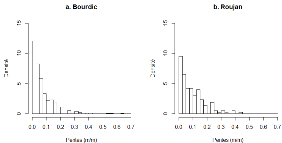
FIGURE 2.5 – Répartition des pentes sur les biefs de longueur supérieure à 15 m : a) Pour le bassin versant du Bourdic, b) Pour le sous-bassin versant de Roujan
