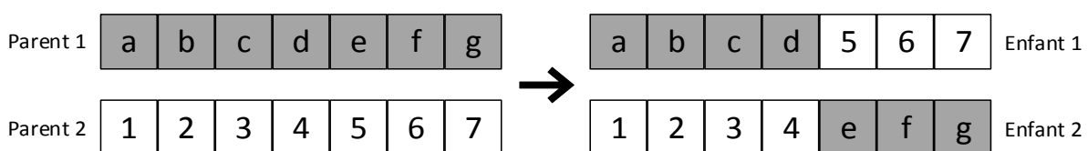
Figure 3.10 : Opération de croisement avec un point de coupe
