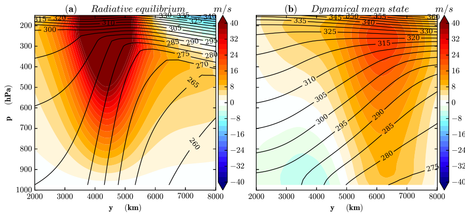
FIGURE 2.12 – Équilibres radiatifs et statistiques. Gauche : Champ de température potentielle à l'équilibre radiatif (contours, en K, tous les 5 K), et vent zonal (couleurs, m/s) associé dans le cadre d'un équilibre géostrophique (équilibre du vent thermique) sous l'hypothèse d'un vent nul à la surface. Droite : Champ de température potentielle (contours, en K, tous les 5 K), et vent zonal (couleurs, m/s), en moyenne temporelle et zonale, sur une intégration de la simulation CTRL .
