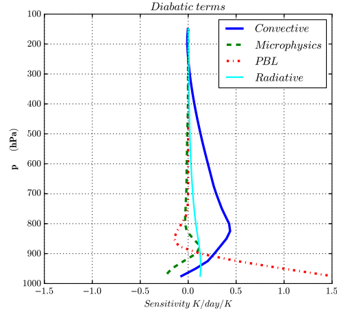
FIGURE 3.6 – Profils de chauffage et bilan de chaleur à la verticale des tourbillons. Les différents termes Q_i(x,y,z) du bilan de chaleur sont calculés localement pour chaque point de l'espace, à partir d'une régression linéaire entre les anomalies de chauffage et les anomalies de SST ( SST_{eddy} ). L'anomalie de chauffage est calculée en soustrayant la moyenne zonale. Les profils Q_i(p) présentés sont les coefficients de régressions (en K/jour/K), à partir des réalisations de Q_i(x,y,z) et SST_{eddy}(x, y) sur la bande de latitudes comprises entre y=3600 km et y=5400 km. Les courbes correspondent aux chauffages associés au schéma de convection (bleu), au schéma radiatif (cyan), au schéma de couche limite (rouge) et à la microphysique (vert) tels que décomposés dans le modèle WRF.
