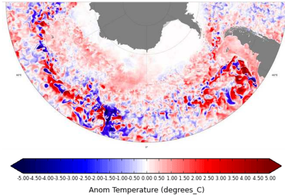
FIGURE 4 – Champ instantané d’anomalie de SST sur une partie de l’hémisphère Sud. Écarts des SST (en K) à leur moyenne climatologique au 01/07/2018, issus de l’analyse opérationnelle MERCATOR.
