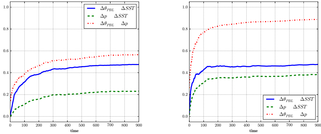
FIGURE 2.2 – Corrélations selon les durées de moyenne utilisées. (a) Coefficients de corrélation spatiale entre les champs de Laplacien de pression de surface ( \nabla^2 p_s ), de température potentielle moyenne entre 0 m et 500 m ( \nabla^2 \theta_{PBL} ), et de SST ( \nabla^2 SST ). Les champs correspondent à des moyennes temporelles sur des durées de plus en plus longues, indiquées sur l’axe des abscisses. Les courbes sont obtenues à partir de la simulation EDDY 1K , en se restreignant à la bande de latitude entre 3600 et 5400 km pour laquelle les variations de la température de surface de l’océan ont la plus grande amplitude. (b) Même chose, à partir de la simulation EDDY .
