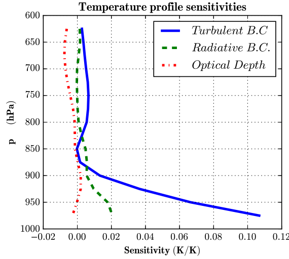
FIGURE 2.11 – Prise en compte des SST dans le schéma radiatif. Coefficients de régressions linéaires spatiale (en K/K), obtenus pour les anomalies du champ de SST \text{EDDY}_{1K} , entre les profils de température potentielle moyens \theta^*(x, y, p) , et le champ de SST \text{SST}^*(x, y) . Les trois courbes correspondent à des moyennes temporelles sur de courtes simulations (1 an) pour lesquelles les différents effets possibles des SST sont isolés : effet sur les flux turbulents à la surface (bleu), effet sur le flux radiatif à la surface (vert), effet sur l'épaisseur optique D (rouge).
