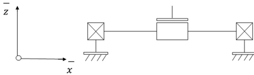
Figure 9 Représentation cinématique de l'interface DEMA, vue de face
