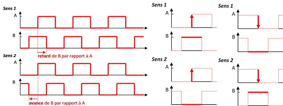
Figure 16 Exemple de déphasage entre les voies A et B (à gauche) ; Front montant et descendant (à droite)
