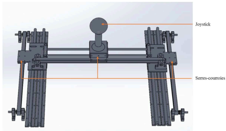
Figure 12 DEMA vu de \frac{3}{4} face
