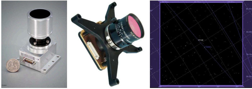
FIGURE 4.1 – Capteurs optiques envisageables : Viseur d'étoiles Auriga de Sodern (France), imageur C1U de GomSpace (Pays-Bas), à droite simulation de champ de vue ( 5^\circ \times 5^\circ ) avec objet d'avant-plan.
