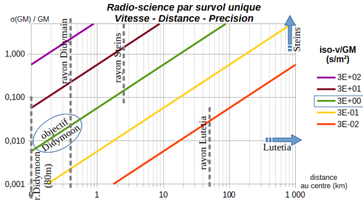
FIGURE 2.7 – Précisions atteintes par radio-science lors d’un survol unique ( \sigma_v = 0.02 \text{ mm/s} , quelques iso- (v/GM) donnés en table 2.4).
