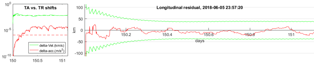
FIGURE 6.5 – Synthèse filtre séquentiel. Haut en bas : i) synthèse sur tout le scénario ; ii) convergence du filtre à chaque ré-initialisation (statut vert/rouge/gris, et residu longitudinal) ; iii) zoom à la date 150 : convergence du filtre, iv) ellipsoïde 3\sigma ; v) (à g.) convergence des vitesses et accélérations, (à dr.) détail des résidus longitudinaux (droite). \sigma_{opt} = 0.2''
