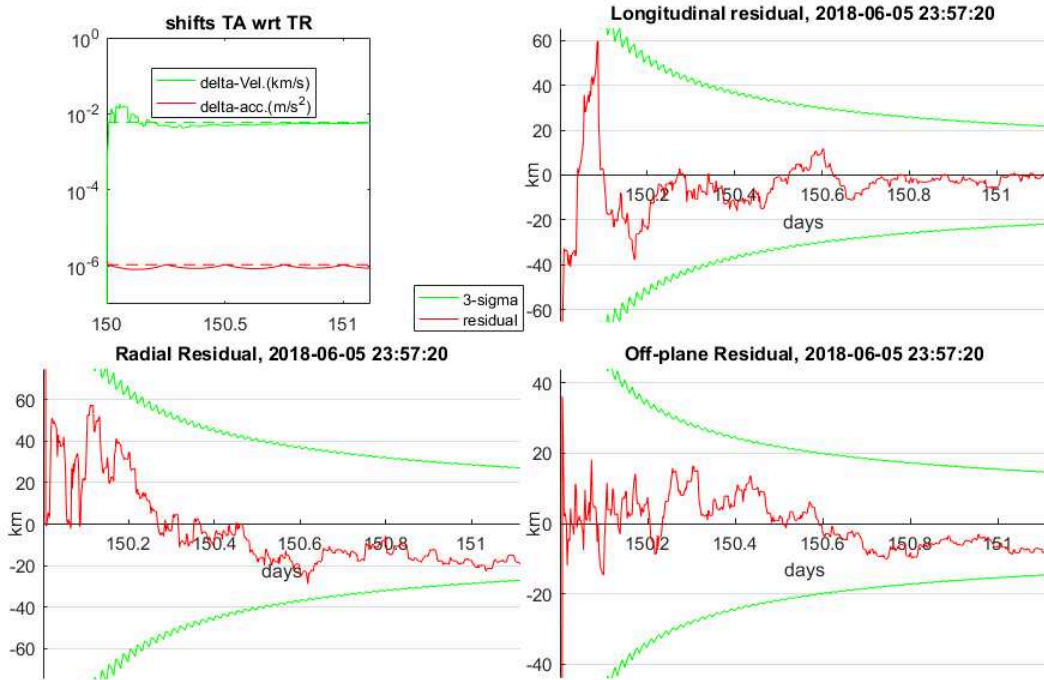
FIGURE 6.6 – Filtre UKF (non-linéaire) . Haut : Synthèse sur tout le scénario avec état de convergence du filtre à chaque ré-initialisation. Centre et bas : convergences vitesse et accélération (centre gauche), résidus longitudinaux (centre droite), radiaux (bas gauche), normaux (bas droite). \sigma_{opt} = 0.2'' .
