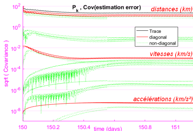
FIGURE 6.1 – Évolution de P_k^+ : termes \sqrt{(S P_k^+ S)_{i,j}} diagonaux en rouge, non diagonaux en vert ; ordonnées en km, km/s ou km/s 2 .
