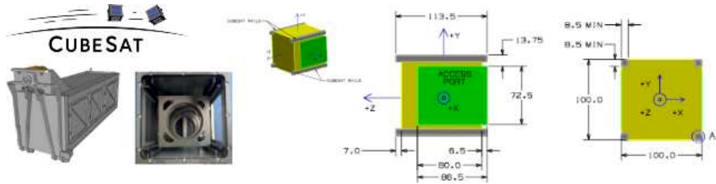
FIGURE 2.1 – Extractions du CubeSat Design Specification, Rev.13 : à gauche le dépoyeur (design extérieur et photo de l'intérieur), à droite les dimensions pour 1U
