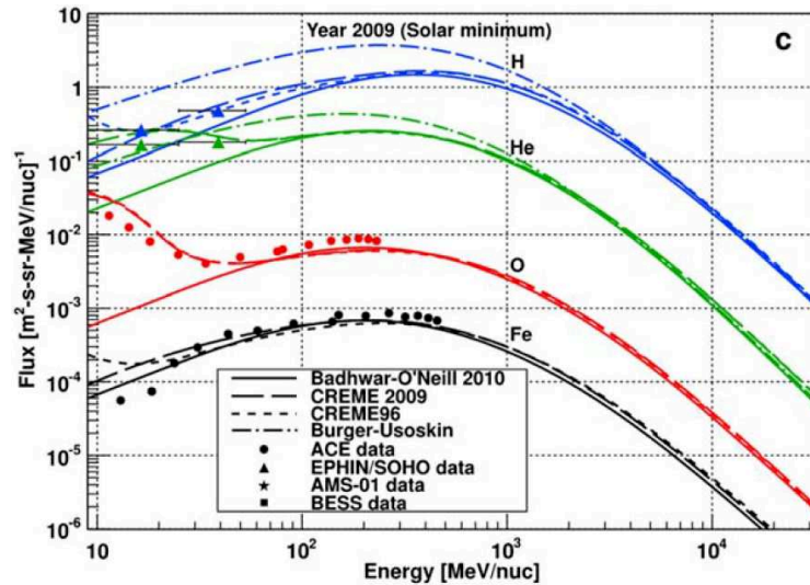
FIGURE 2.3 – Modèles d'abondances de différentes particules cosmiques galactiques ( H , He , O , Fe ) en fonction de leur énergie Mrigakshi et al. [2]
