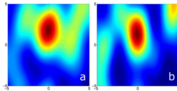
FIGURE 3.5 – Image radio de VENUS EXPRESS, obtenues avec 7 (a) et 8 (b) antennes du réseau VLBI EVN, échelles en millisecondes d’angle (exemples, Duev et al. [36]).
