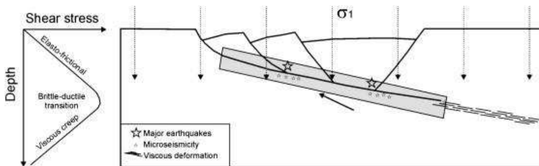
Figure 25: représentation schématique (Collettini, 2011) d'une faille normale à faible pendage, dans laquelle viennent s'enraciner des failles à pendage plus élevée. Une telle géométrie est suspectée par exemple dans les Apennins ou dans le golfe de Corinthe. Du glissement lent, accompagné de micro-sismicité, a lieu sur le détachement, alors que les failles normales inclinées peuvent porter des séismes majeurs (ex. Aquila, 2009).
