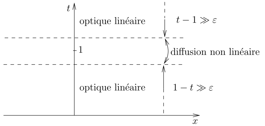
FIG. 3.4 – Propagation linéaire, caustique non linéaire.
