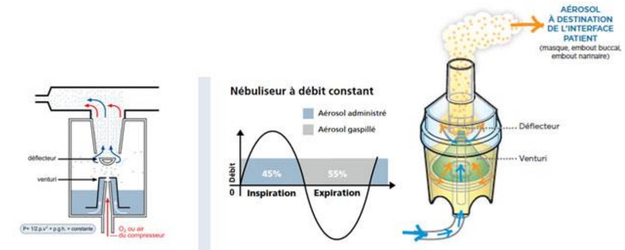
Figure 21 - Exemple de système de nébulisation pneumatique Systam© : système Venturi à débit constant
