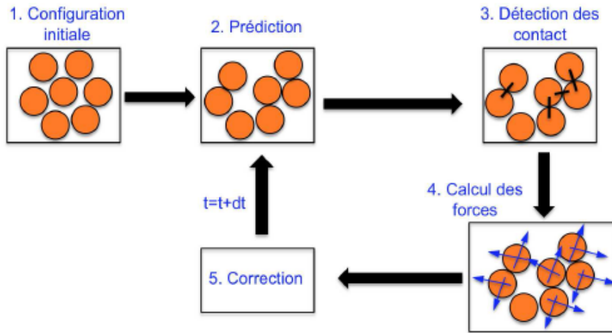
FIGURE 9.1 – Illustration des phases principales du code "LMGC90"
