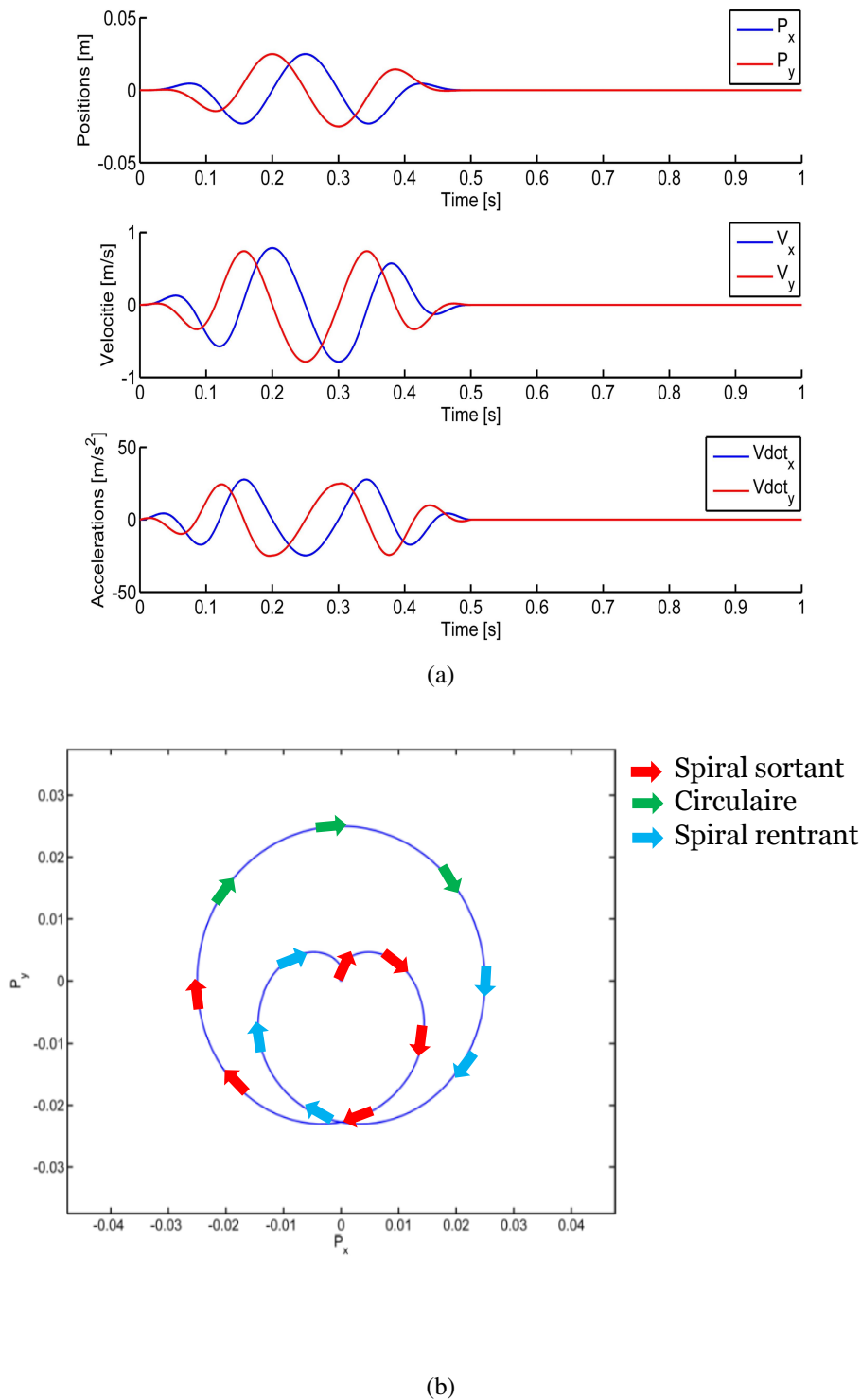
FIGURE 6.10 – Fonctions de contraintes (a) et la trajectoire du support (b)
