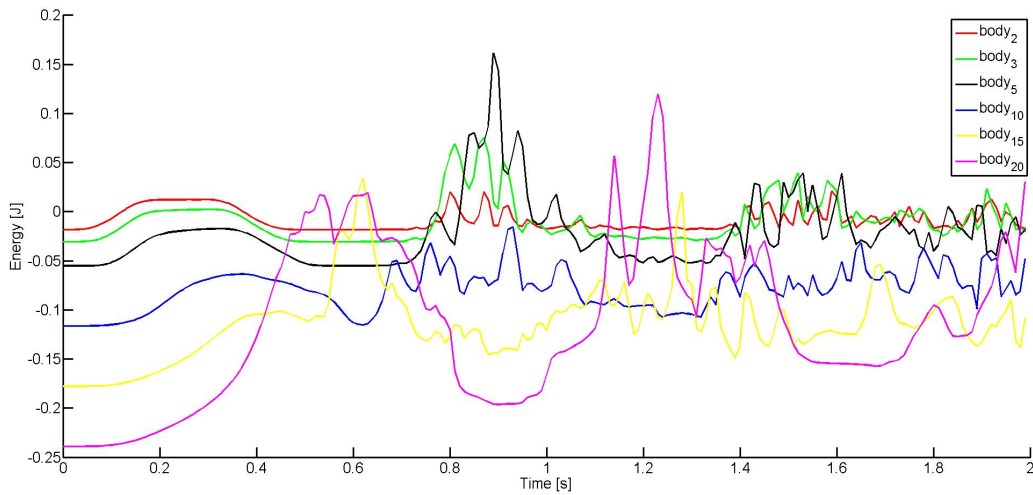
FIGURE 6.11 – Énergie totale des différents éléments illustrant la propagation de l'onde spirale
