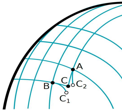
FIGURE 8.1 – La méthode du filet [Boisse, 2004]
