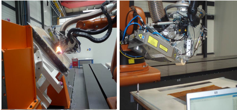
FIGURE 2.6 – Machine de placement de fils pré-impregnés développée par Coriolis Composites [Barasinski, 2012]
