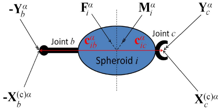
FIGURE 4.9 – Diagramme de corps libre d'un sphéroïde i appartenant à une fibre \alpha [Ross and Klingenberg, 1997]
