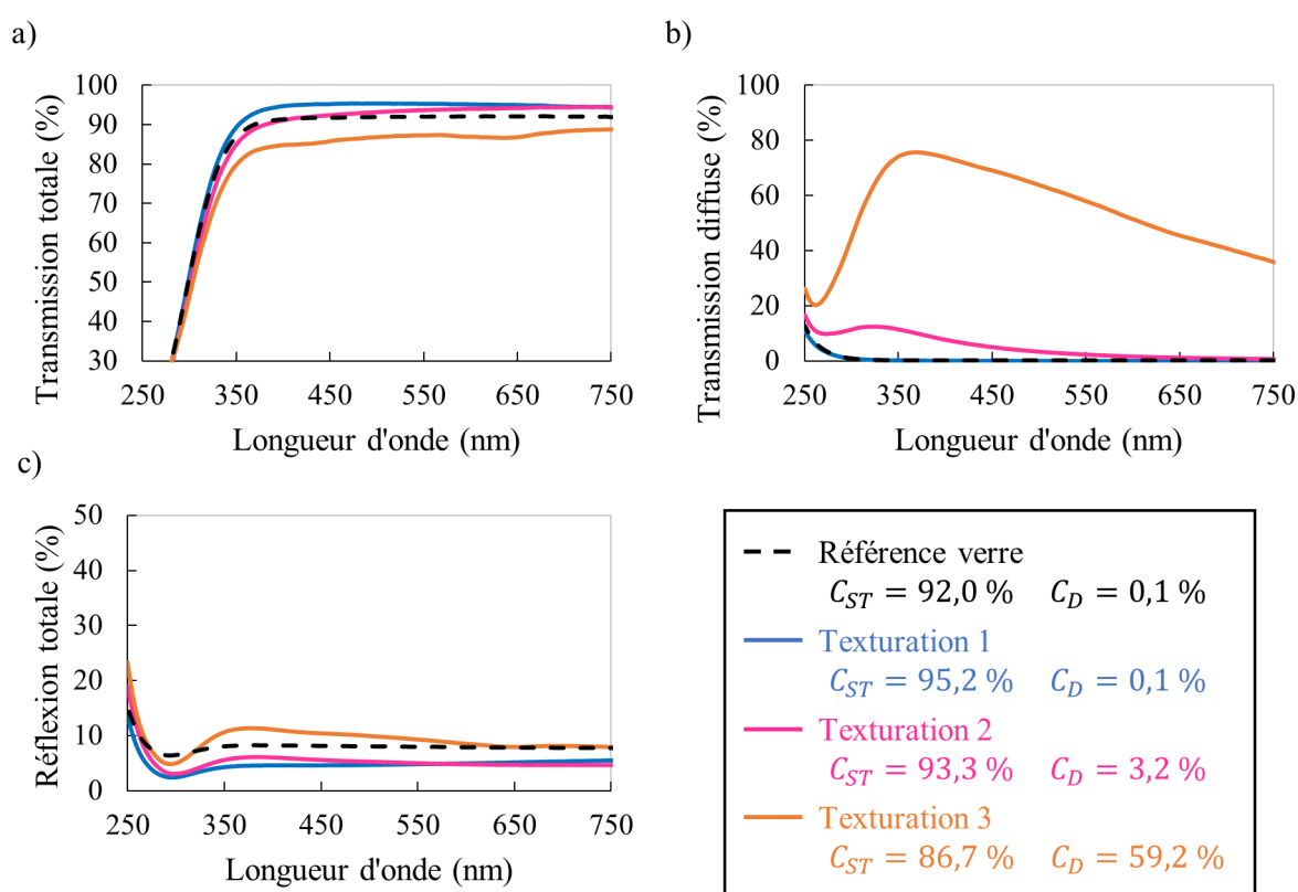
Figure 3-14. Transmission a) totale, b) diffuse et c) réflexion totale d'un substrat en verre texturé. Les valeurs du critère de semi-transparence et de diffusion sont également reportées.
