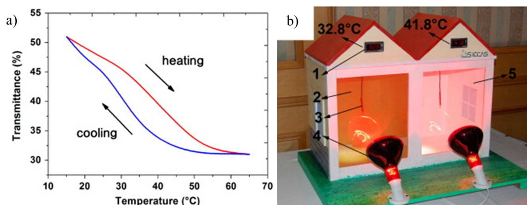
Figure 1-11. Gestion thermique par thermochromie [60] : a) hystérésis d'un film VO 2 dopé W et b) exemple d'utilisation sous lampe infrarouge avec à gauche la température derrière un verre VO 2 et à droite derrière un verre flotté vierge.
