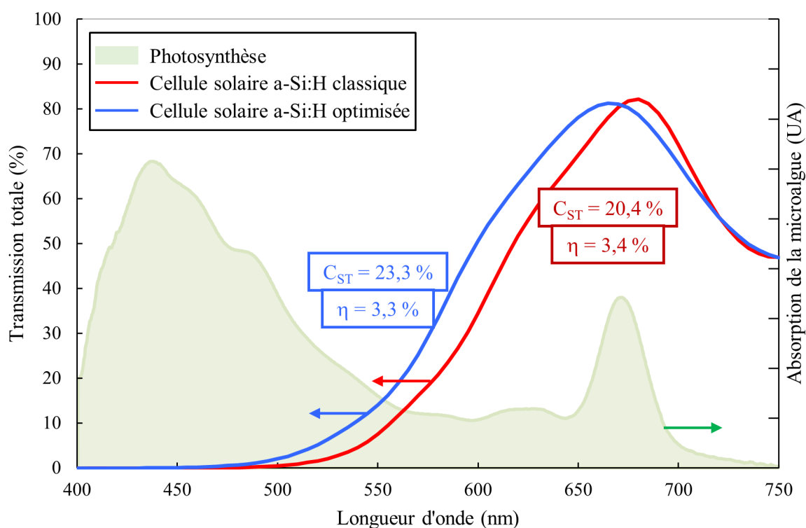
Figure 3-8. Comparaison de la transmission et du rendement PV d'une cellule solaire optimisée par simulation puis réalisée avec une cellule solaire à l'empilement classique.
