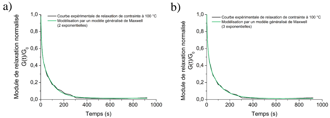
Figure 3-31 : Modélisation de la relaxation de contrainte à 100 °C du matériau hybride C ( Ti : -CO_2H = 1 : 1,5 ) par un modèle généralisé de Maxwell à a) deux ou b) trois exponentielles.
