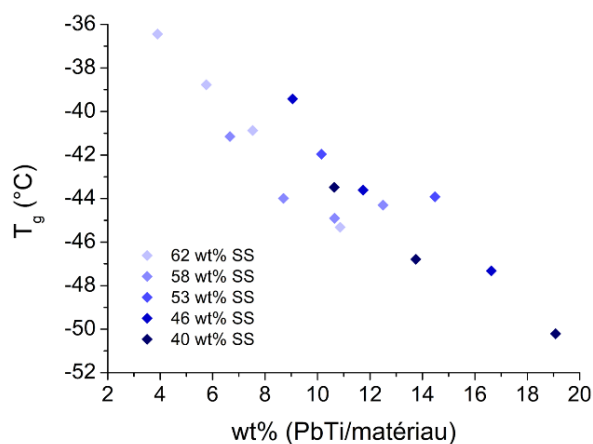
Figure 2-51 : Valeurs des transitions vitreuses en fonction du pourcentage massique de polydiethyltitanate dans le matériau.
