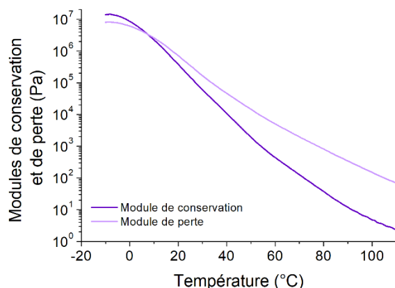
Figure 2-20 : Modules de conservation et de perte du prépolymère C obtenus par rhéologie ( F_N = 0,01 \text{ N} , \gamma = 1 \% , \omega = 1 \text{ s}^{-1} ).
