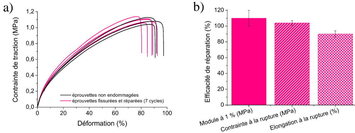
Figure 3-23 : a) Courbes élancement/rupture du matériau hybrC (1 : 2), après 7 réparations de fissure à 110 °C pendant 15 min sous 60 bars, et de son témoin ; b) Efficacités de réparation correspondantes.
