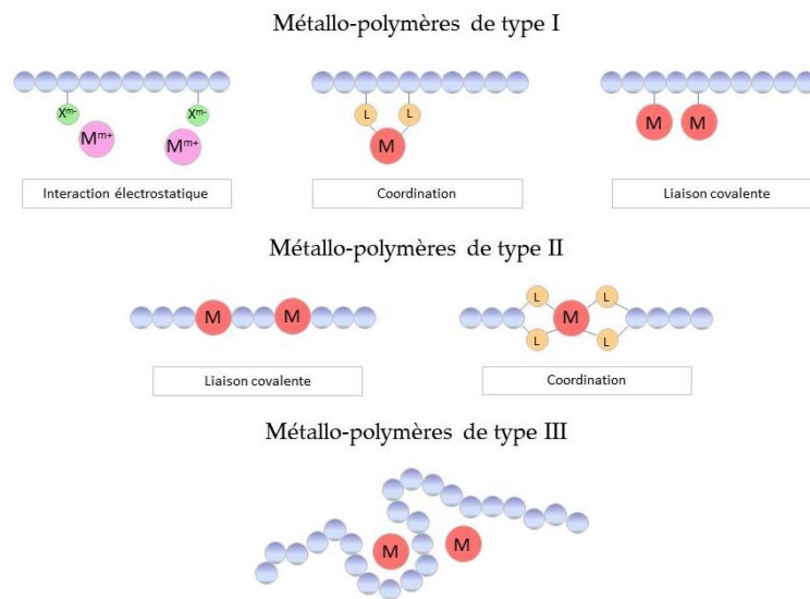
Figure 2-1 : Les différentes classes de métallo-polymères. [7]
