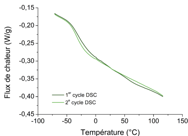
Figure 4-18 : Thermogrammes obtenus pour le matériau hybrC (1 : 2) testé à 90 %HR pendant 24 heures à 50 °C (1 er et 2 e cycles) (exo up).
