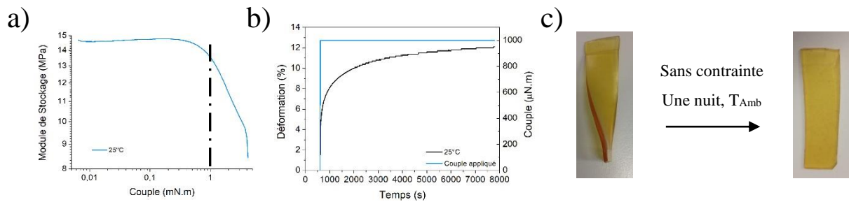
Figure 3-45 : Pour un matériau hybride hybrC (1 : 2), a) test de balayage en amplitude (1 à 10 %) à 25 °C ; b) courbe de fluage à 1 mN.m à 25 °C et c) devenir du matériau à température ambiante sans contrainte.
