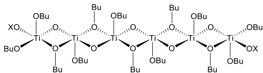
Figure 2-28 : Représentation plus réaliste du polydibutyltitanate (pour n = 6 ) avec X = \text{Ti} ou -\text{Bu} et avec le titane en coordinence 5 comme pour \text{Ti}(\text{OBu})_4 qui est sous forme trimère.
