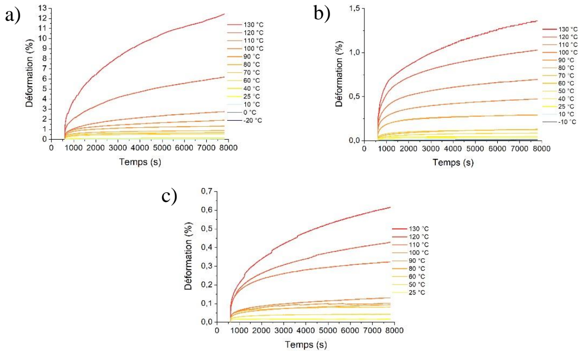
Figure 3-35 : Courbes de fluage pour les matériaux hybrides a) hybrC (1 :2) ( \sigma = 2\ 000\ Pa ), b) hybrC (1 : 1,5) ( \sigma = 2\ 000\ Pa ) et c) hybrC (1 : 1) ( \sigma = 10\ 000\ Pa ).
