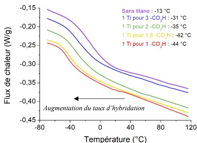
Figure 2-49 : Thermogrammes obtenus par DSC à 10\text{ °C/min} du prépolymère C et des différents hybrides synthétisés à partir de ce prépolymère (exo up). Les thermogrammes ont été décalés en ordonnée pour des raisons de lisibilité.
