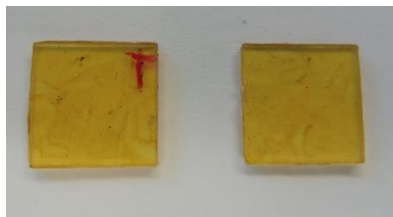
Figure 4-27 : Matériaux hybrC (1 : 2) témoin (à gauche) et ayant subi les conditions d'humidité élevée (50 °C, 50 %HR, 24 heures) (à droite) réparés sous presse à compression (110 °C / 15 min / 60 bars).
