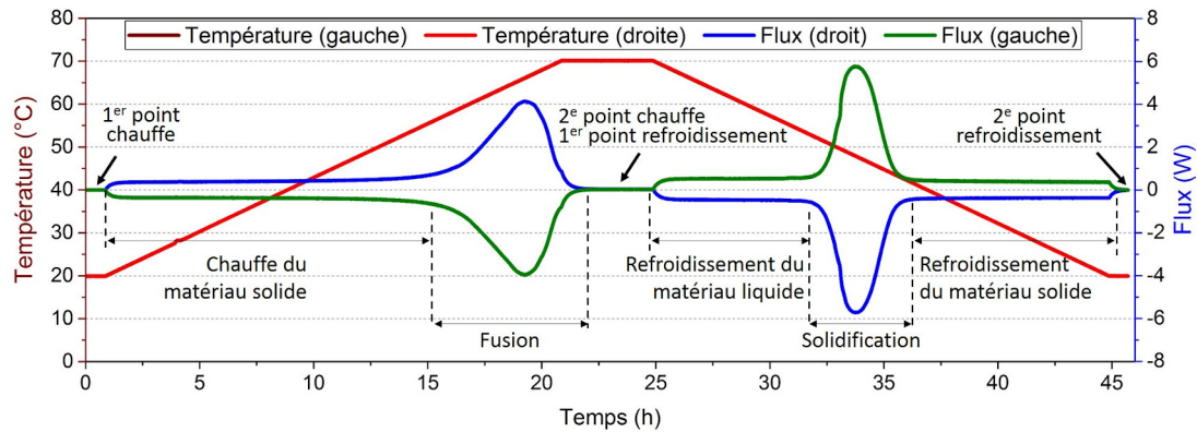
Figure 3.8 – Analyse d'un cycle des différentes phases du processus et de fusion et de solidification, obtenu sur le BF à partir d'une chauffe et d'un refroidissement ( 2,5\text{ }^{\circ}\text{C.h}^{-1} ). Les températures (courbes rouges, superposées à faible vitesse) dépendent de l'axe des ordonnées de gauche, celui du flux (courbes bleue et verte) de l'axe de droite. Les points d'intégration du flux ont également été repérés.
