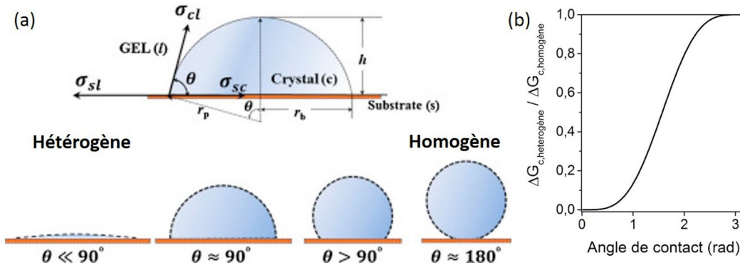
Figure 2.10 – (a) Calcul de l'angle de contact pour la formation d'un germe entre 3 phases (SL : substrat-liquide ; SC : substrat-cristal ; CL : cristal-liquide), adapté de [109] et (b) Variation du rapport d'enthalpie libre hétérogène critique sur l'enthalpie libre homogène critique de formation d'un cristal en fonction de l'angle de contact [21]
