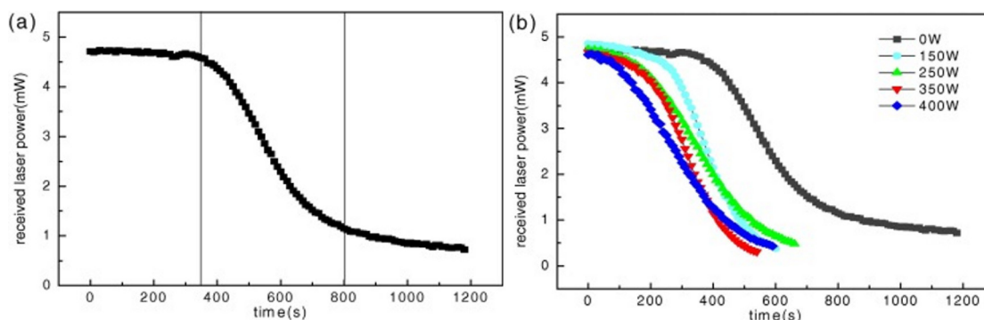
Figure 2.29 – (a) Les différentes étapes de solidification par laser (essai à 0 W) (b) Étude de l'influence des ultrasons sur l'opacification du laser [180]
