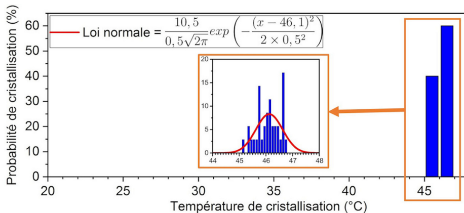
Figure 7.14 – Distributions des probabilités de cristallisation en fonction de la température, et approximation par une loi normale, pour l'échantillon contenant un ajout d'eau (AST54%)
