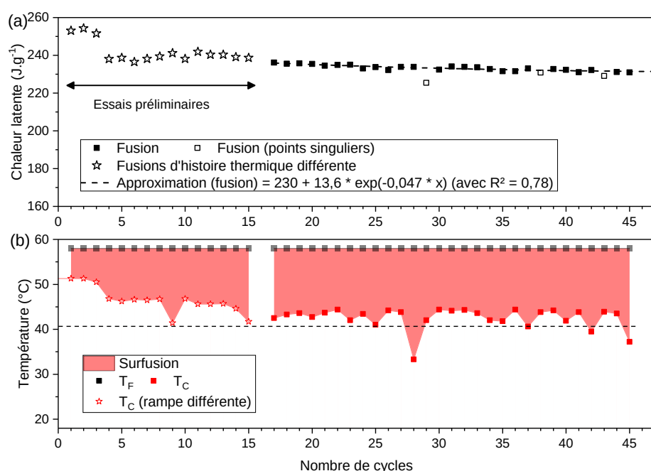
Figure 7.9 – Évolution (a) de la chaleur latente et (b) du degré de surfusion sur 45 cycles d'un deuxième échantillon de concentration brute ( w_{AS} = 0,603 )
