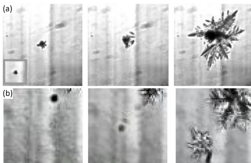
Figure 2.21 – (a) Cristaux de glace générés par une bulle à 0,55 bar, -3,26 °C à différents instants ( t=0.030 s ; t=0.055 s ; t=0.255 s) (b) Différents cristaux générés par une seule bulle se déplaçant vers le ventre de pression à -3,2 °C et 1,2 bar à différents instants ( t=0 s ; t=0.022 s ; t=0.053 s) [158]
