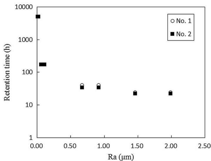
Figure 2.2 – Temps de maintien de la surfusion de solutions d'acétate de sodium en fonction de la rugosité Ra à 15\text{ }^{\circ}\text{C} . L'expérience a été répétée deux fois [46].
