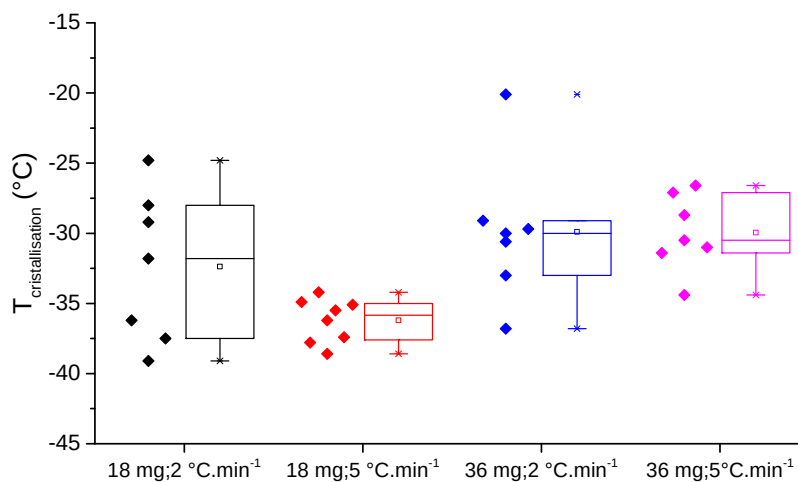
Figure 3.10 – (a) Détermination de la température de cristallisation à partir de l' onset (croisement des tangentes du pic exothermique) et (b) Évolution de la température de cristallisation en fonction de deux conditions de volume et de vitesses de refroidissement
