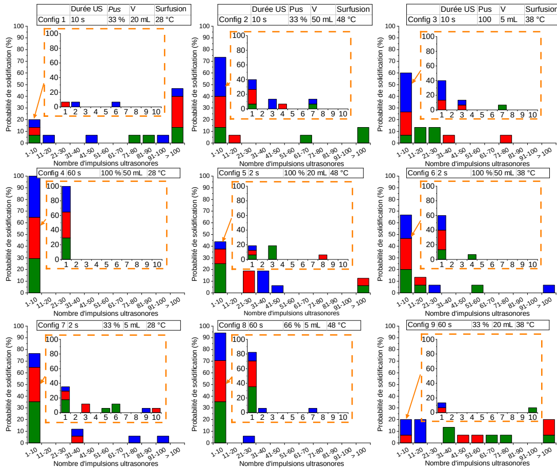
Figure 6.6 – Probabilités de solidification, calculées par l'équation 6.1, pour les différentes configurations d'essai du plan d'expérience. Config : configuration, V : Volume, Pus : Puissance fournie par ultrasons (% puissance nominale). En vert : tube 1 ; en rouge : tube 2 ; en bleu : tube 3. Une vue détaillée des 10 premiers cycles apparaît aussi pour l'ensemble des configurations d'essais
