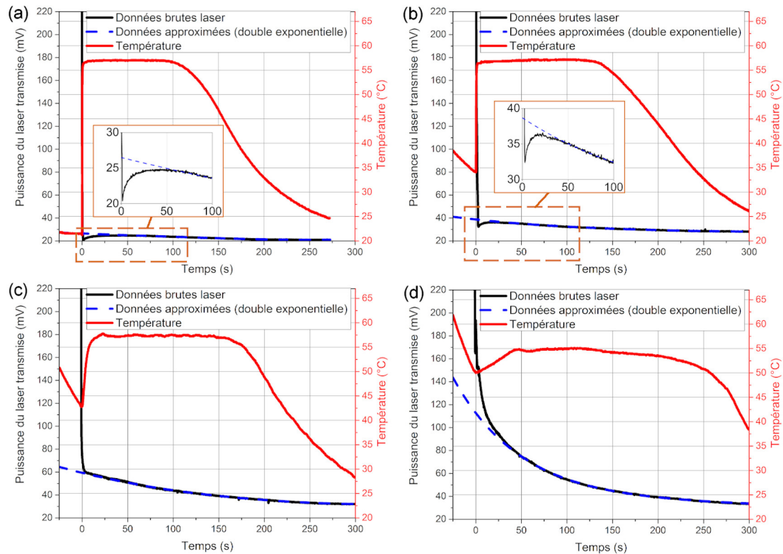
Figure 5.6 – Température et puissance laser reçue au cours du temps pour différentes surfusions : (a) \Delta T = 37\text{ °C} ; (b) \Delta T = 24\text{ °C} ; (c) \Delta T = 15\text{ °C} ; (d) : \Delta T = 8\text{ °C} . L'instant initial (Temps = 0 secondes) correspond au moment où la recalescence a été détectée par le thermocouple.
