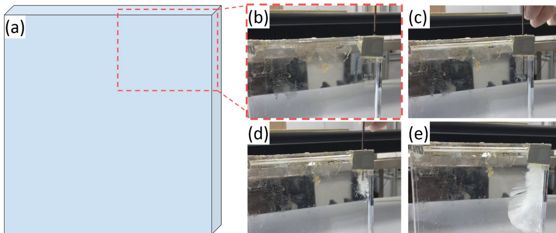
Figure 3.17 – Solidification par ensemencement avec une baguette de soudure. (a) Schéma de la brique en PMMA sortie du banc pour permettre une visualisation du phénomène. Vue détaillée à (b) l'état initial avant son insertion ; (c) l'insertion ; (d) le démarrage de la cristallisation et (e) la croissance du cristal dans le volume.
