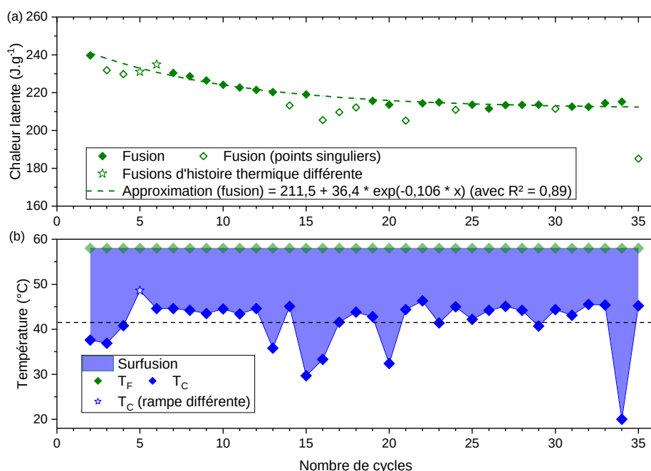
Figure 7.7 – Évolution (a) de la chaleur latente et (b) du degré de surfusion sur 35 cycles d'un échantillon de concentration brute ( w_{AS} = 0,603 ). Les valeurs des cycles 5 et 6, d'histoire thermique différente, sont représentées par des étoiles et n'ont pas été utilisées pour la loi de décroissance exponentielle et l'analyse de vieillissement
