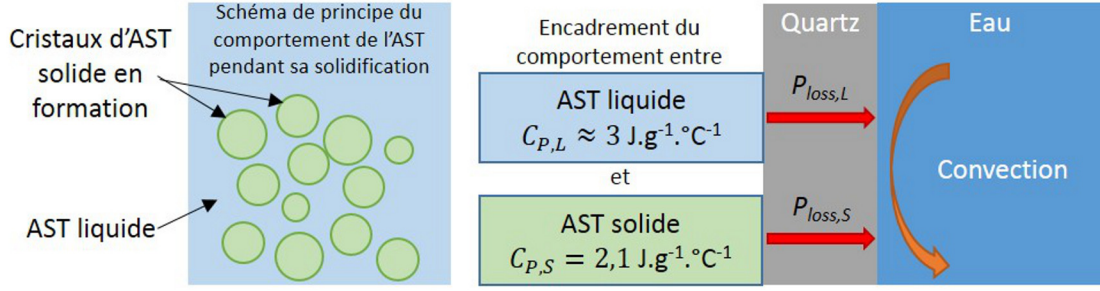
Figure 5.4 – Encadrement du comportement théorique de notre matériau entre celui d'un matériau complètement liquide et complètement solide
