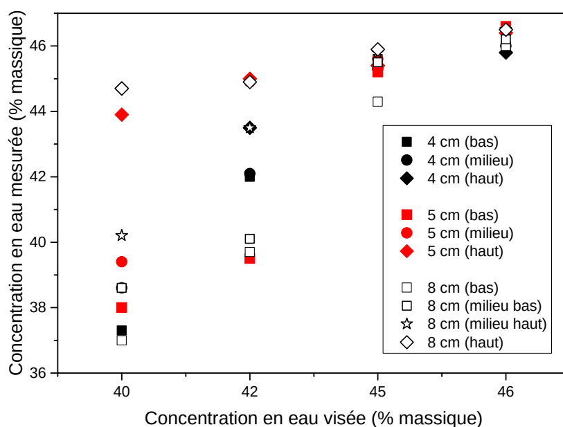
Figure 2.34 – Mesure de la concentration en eau pour différentes positions d'échantillons (bas, milieu, haut) dans des récipients de différentes hauteurs (4 ; 5 ; 8 cm), surfondues pendant 131 jours. Adapté de [206]
