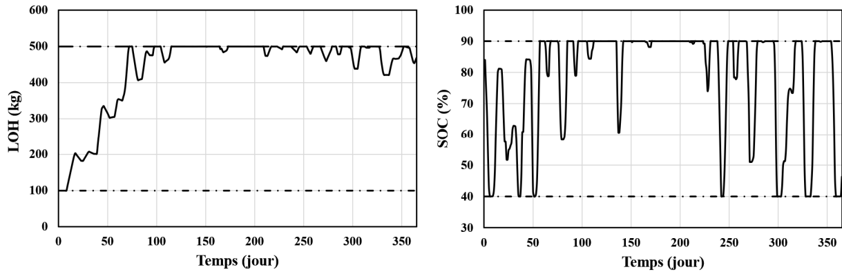
Figure 4.8. Niveau du réservoir d'hydrogène (gauche) et état de charge de la batterie (droite).
