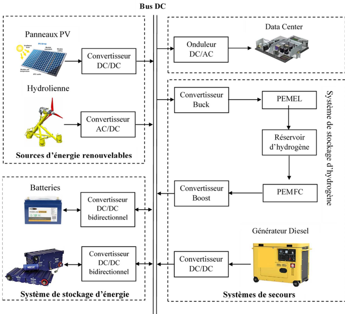
Figure 1.13. Architecture d'un système hybride isolé.
