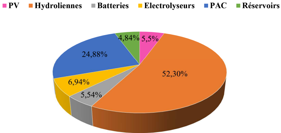
Figure 3.26. Contribution de chaque source d'énergie au coût actuel net (NPC).
