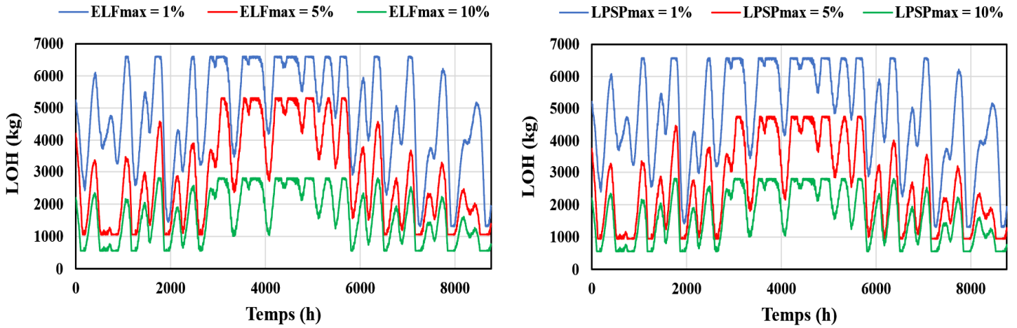
Figure 3.25. Quantité d'hydrogène dans les réservoirs pour différents indices de fiabilité (configuration Hydrolienne/PV/Batterie/H 2 ).
