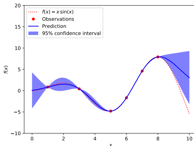
FIGURE 1.4 – Le Krigeage formule un modèle de substitution à partir d’observations de la fonction à approximer. Une estimation de l’incertitude est disponible pour chaque prédiction du modèle [127].
