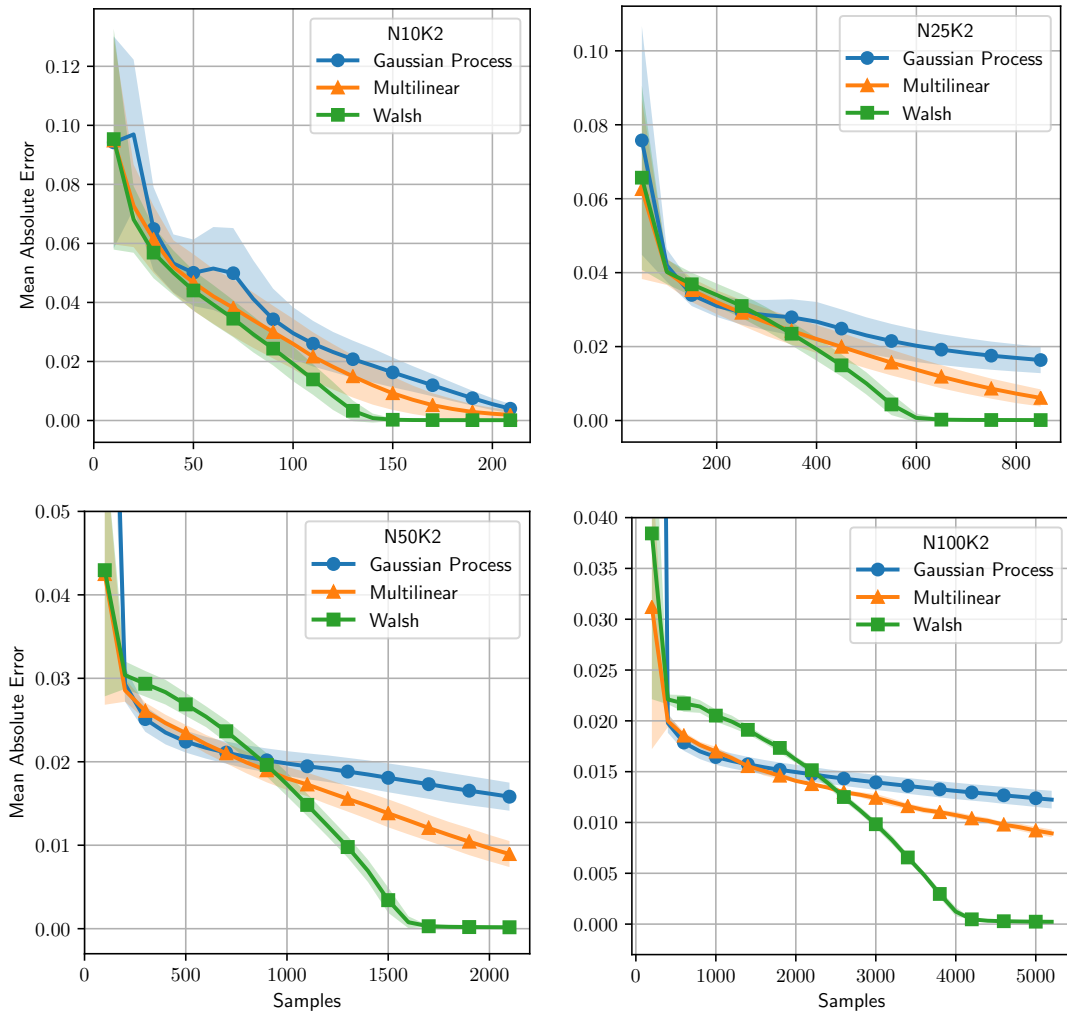
FIGURE 6.3 – Moyenne de l’erreur absolue sur un échantillon de test et intervalles de confiance des méta-modèles sur des paysages N_K de diverses dimensionnalités, en fonction du nombre d’échantillons aléatoires dédiés à leur apprentissage. Le paramètre k est fixé à 2.
