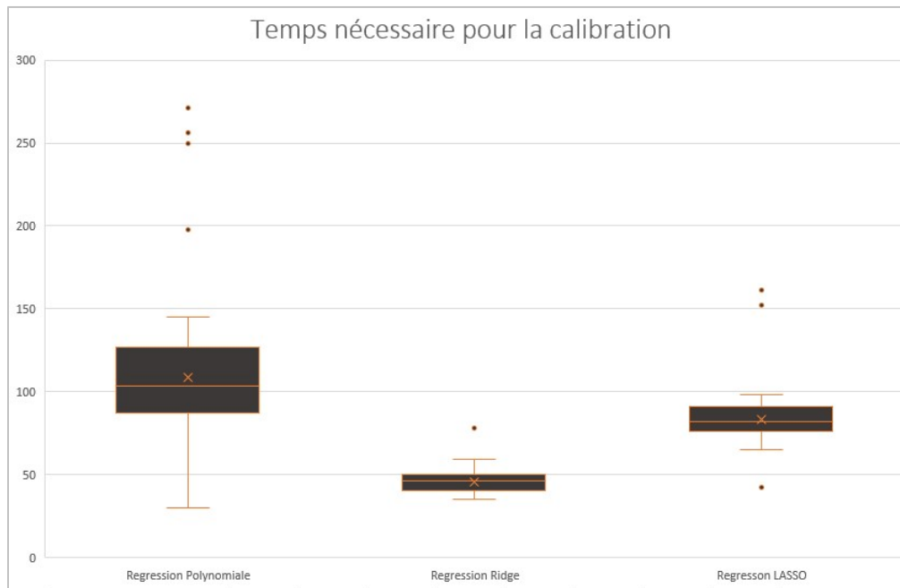
Figure V.16: Distribution des temps de chargement de chaque modèle sur l'échantillon des 500 références
