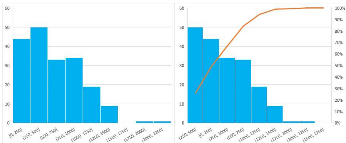
Figure V.20: La distribution de l'erreur de prévision du modèle de régression Ridge.
