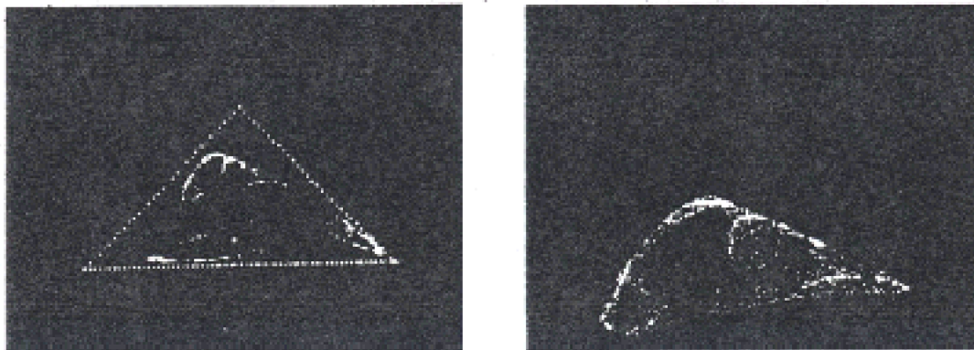
État asymptotique et agrandissement (x3) [STEIN, P., ULAM, S., 1964], p. 475
