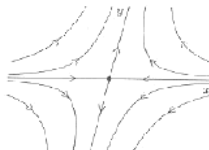
Col : il passe deux courbes intégrales (et deux seulement)
