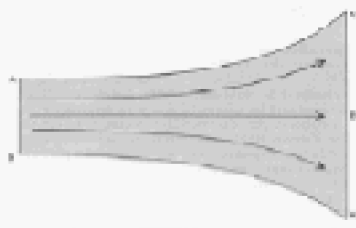
Figure A : étirement des trajectoires
