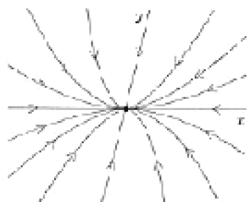
Nœud : une infinité de courbes intégrales passent par le point
