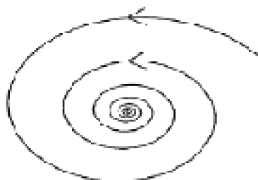
Foyer : les courbes intégrales s'enroulent en spirale
