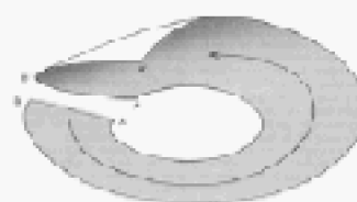
Figure B : repliement des trajectoires
