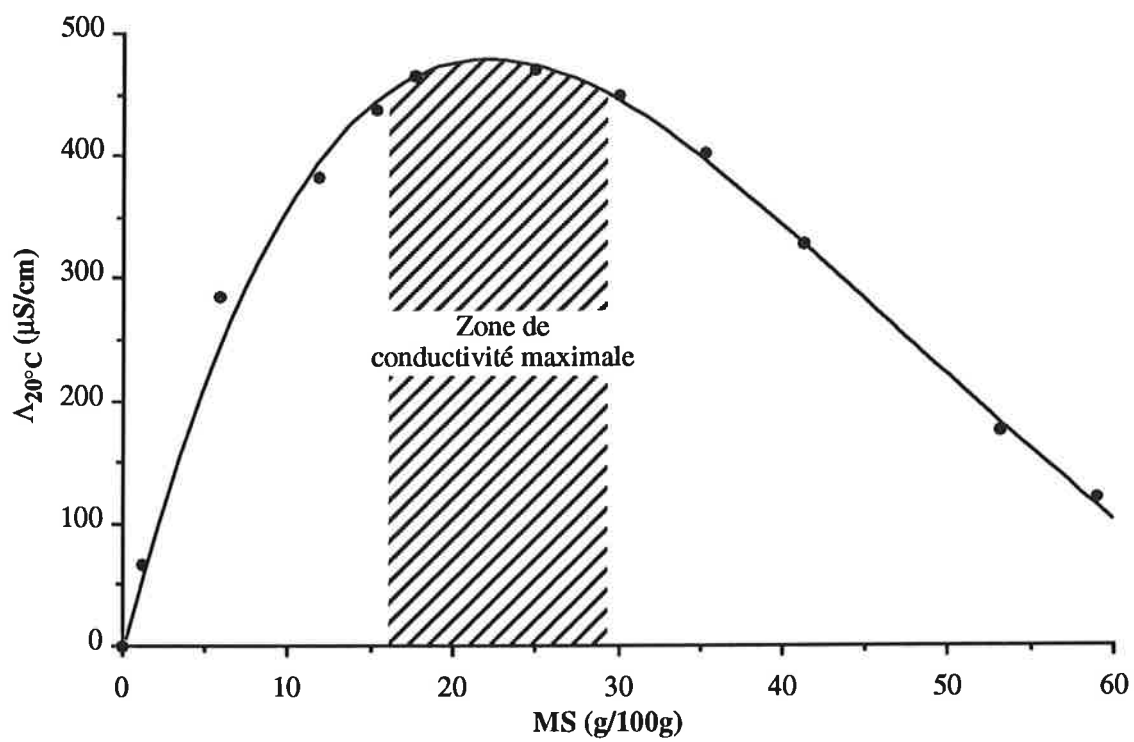
Figure I.14 : évolution de la conductivité à 20 °C d'un sirop de sucre roux ( \Delta_{20^{\circ}\text{C}} ) en fonction de sa teneur en matière sèche (MS) [lot 3].
