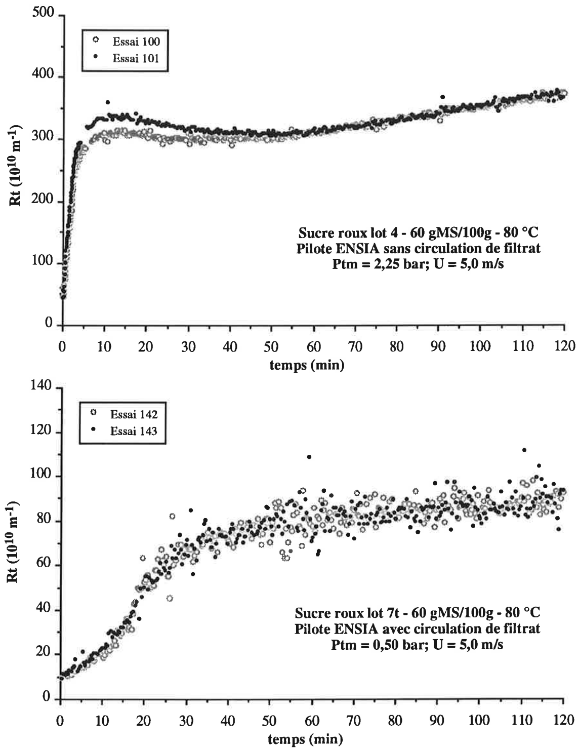
Figure I.12 : exemple d'évolution de la résistance hydraulique totale (Rt) au cours de filtrations réalisées dans des conditions identiques [membrane MEMBRALOX 1,4 µm].
