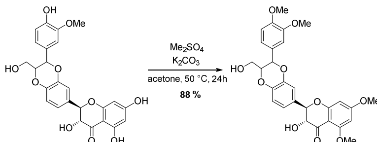
Schéma 163 Protection sélective des alcools phénoliques de la Silibinine
