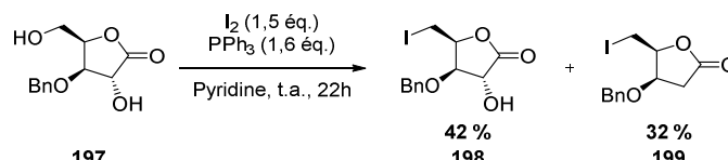
Schéma 120 Iodation et déshydroxylation sur une lactone
