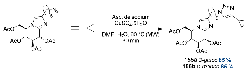
Schéma 49 Synthèse des composés monovalents D-gluco-et D-mannoimidazoles via CuAAC
