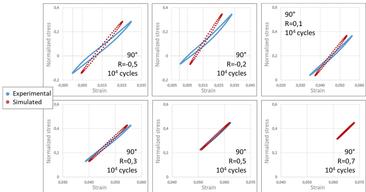
Figure A-3 : Boucles d'hystérèse calculées et expérimentales dans la direction de sollicitation pour des essais uniaxiaux menés sur éprouvettes Dogbone à 90^\circ pour une durée de vie d'environ 10^4 cycles et pour différents rapports de charge
