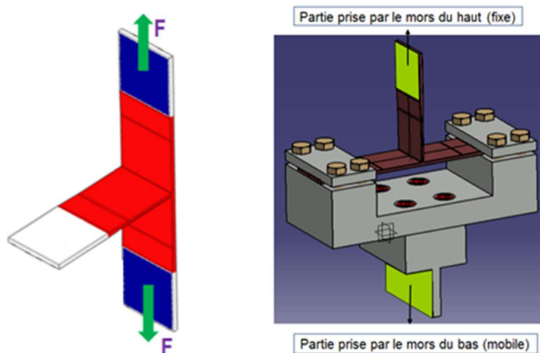
Figure 1-18 : Schématisation des conditions appliquées en traction (à gauche) et en flexion (à droite) aux éprouvettes T-Bone pour une étude de la réponse en fatigue multiaxiale d'un PA66GF50 [Serr15]
