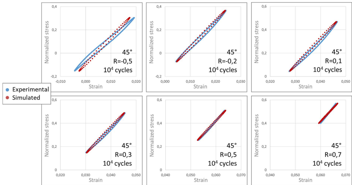
Figure A-2 : Boucles d'hystérèse calculées et expérimentales dans la direction de sollicitation pour des essais uniaxiaux menés sur éprouvettes Dogbone à 45^\circ pour une durée de vie d'environ 10^4 cycles et pour différents rapports de charge
