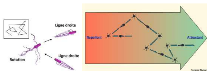
FIGURE 1.3 – À gauche, les mécanismes de mouvement d'une bactérie E. Coli : elle alterne une phase de mouvement en ligne droite et une phase de rotation avec un angle aléatoire. À droite, le mouvement d'une bactérie dans un milieu hétérogène : l'angle de rotation reste aléatoire mais favorise en moyenne les déplacements vers le milieu favorable (en vert). Sources : cronodon.com et [139].
