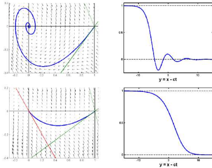
FIGURE 1.16 – Portraits de phase associés à (1.17), avec le profil du front solution. En haut pour c = \frac{1}{2} , en bas pour c = 2 . En vert, la direction instable de l'équilibre (1, 0) , et en rouge la direction stable de l'équilibre (0, 0) .
