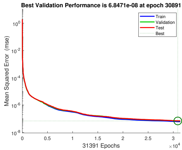
(b) 3L-ANN
