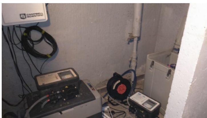
Figure II.29: Système de prélèvement d'un échantillon d'eau sur le parking référence
